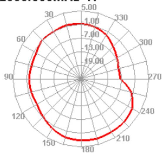
2500.000MHz H
