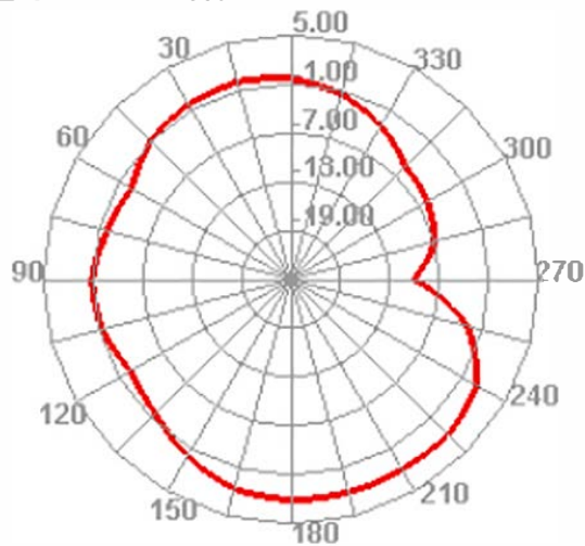
2450.000MHz H
