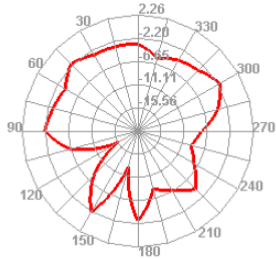
2500.000MHz E2
