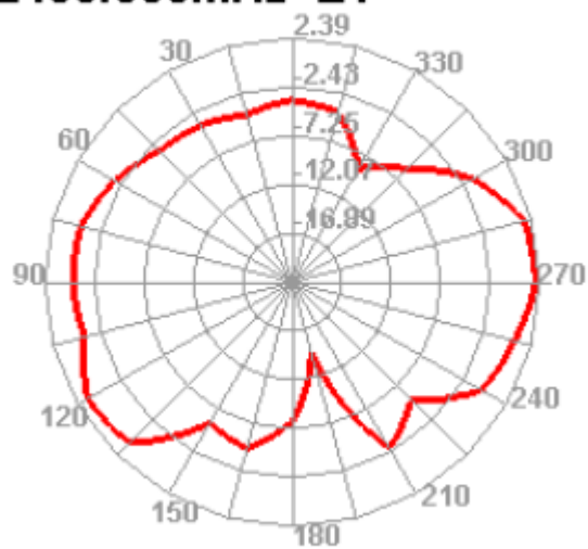
2450.000MHz E1
