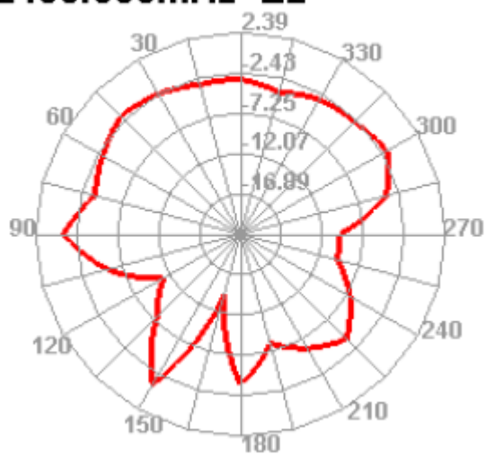
2450.000MHz E2
