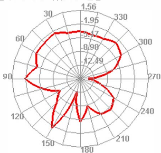
2400.000MHz E2
