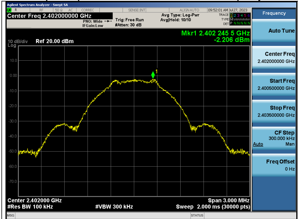
Test_Graph_ANT1_2402_Reference Level
