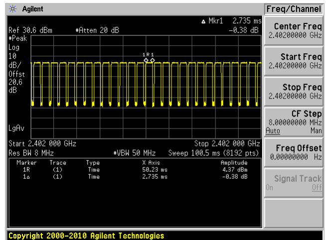
8DPSK Mode
