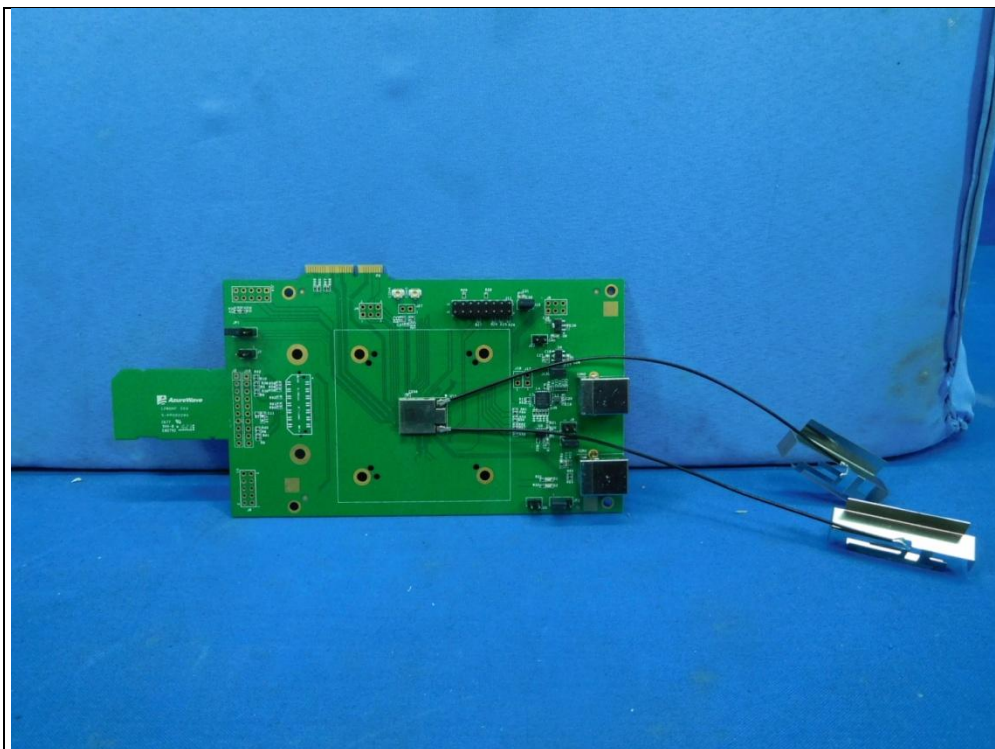
EUT + Test tool + Antenna
