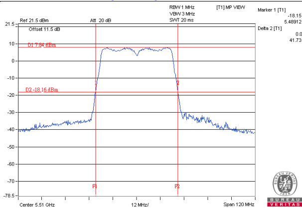
8802.11ac (VHT40)_Chain 1 / CH102
