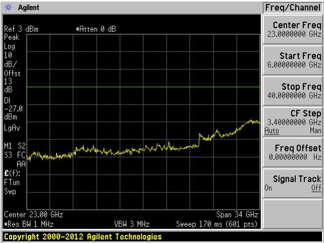
802.11n40 High 5230 MHz (6-40GHz)
