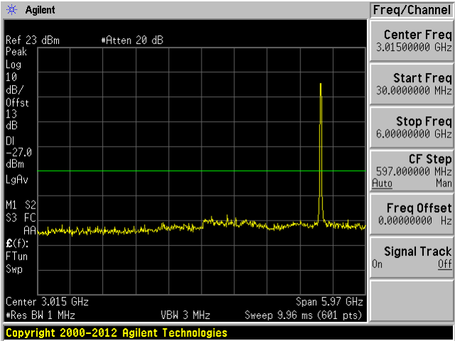
802.11n20 Low 5180MHz (30MHz-6GHz)
