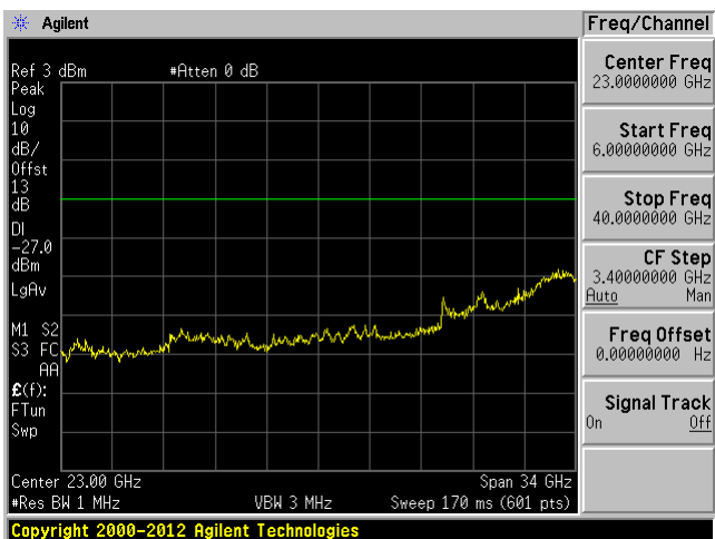
Low 5180 MHz (6-40GHz)
