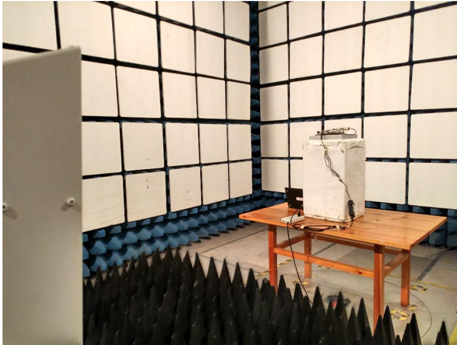
Above 1GHz(RFID)
