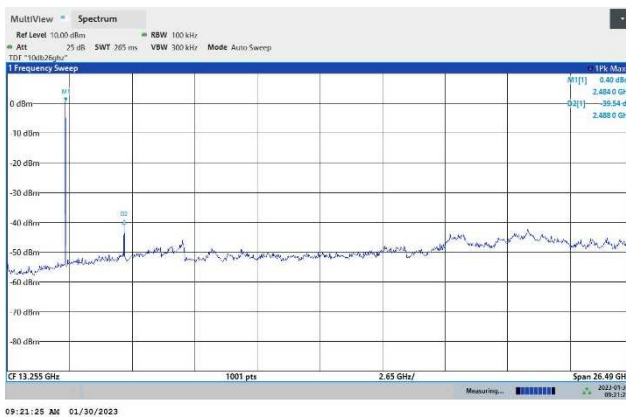
TX 2480: 10 – 26000 MHz
