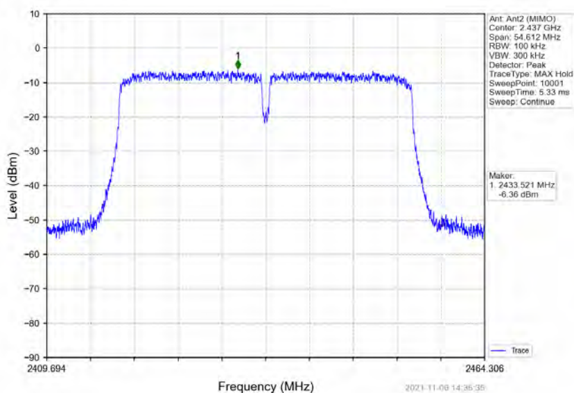
802.11n(HT40) MCH_2437MHz_Ant2 (MIMO) NTNV
