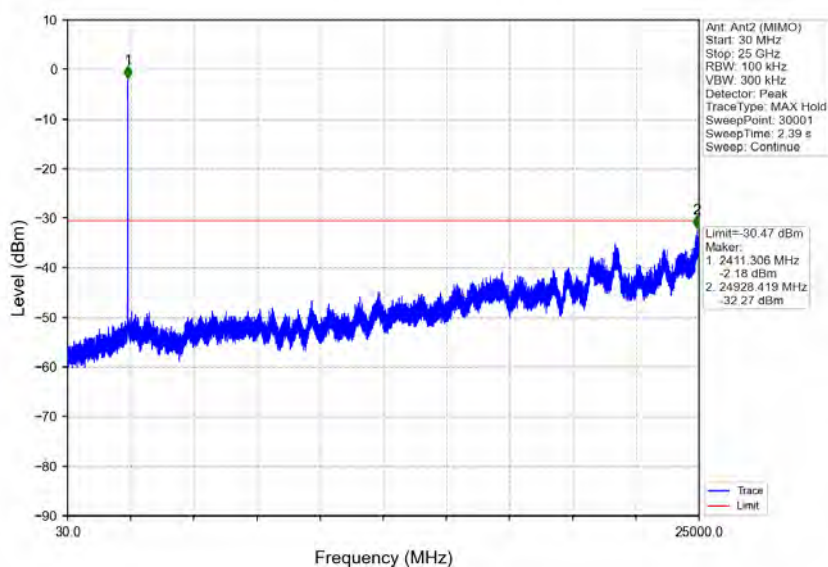
802.11n(HT20)_LCH_2412MHz_Ant2 (MIMO)_NTNV
