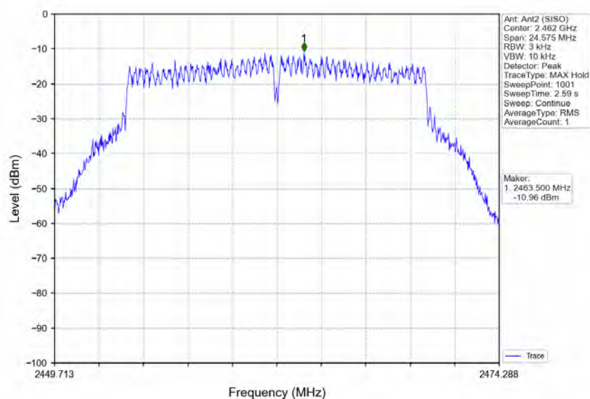
802.11g_HCH_2462MHz_Ant2 (SISO)_NTNV
