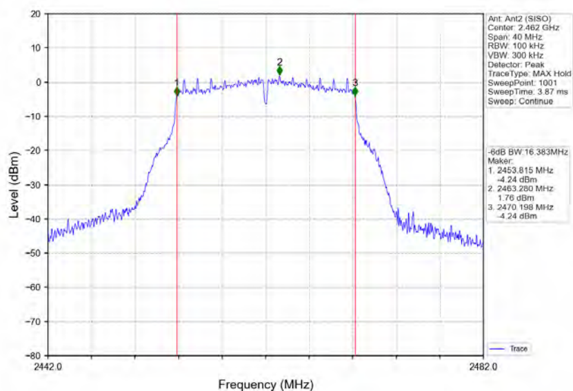
802.11g_HCH_2462MHz_Ant2 (SISO)_NTNV
