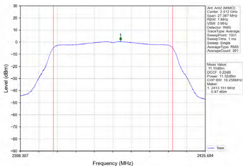
802.11n(HT20)_LCH_2412MHz_Ant2 (MIMO)_NTNV
