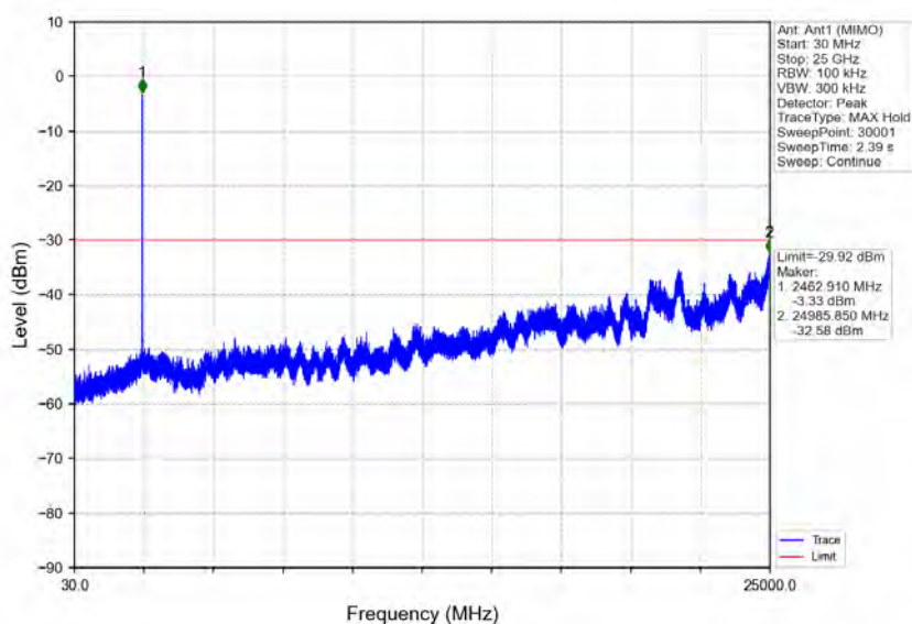
802.11n(HT20) HCH 2462MHz Ant1 (MIMO) NTN
