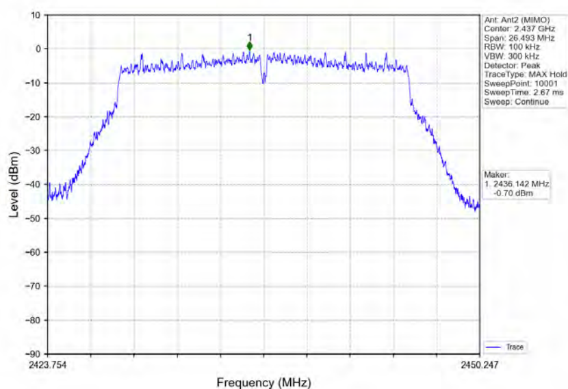
802.11n(HT20) MCH 2437MHz Ant2 (MIMO) NTVN
