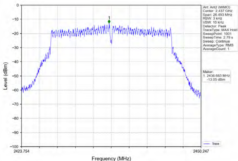
802.11n(HT20)_MCH_2437MHz_MIMO_NTN
