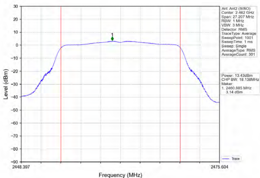
802.11g_HCH_2462MHz_Ant2 (SISO)_NTNV
