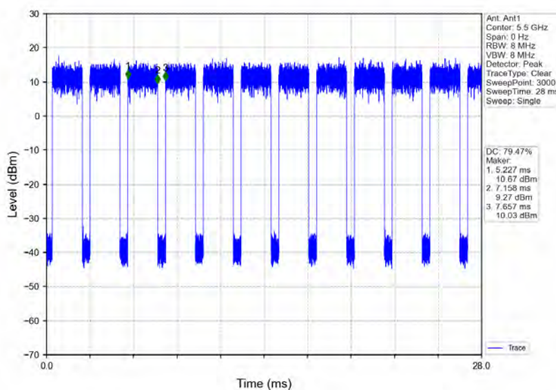
802.11ac(VHT20) LCH 5500MHz Ant1 NTV
