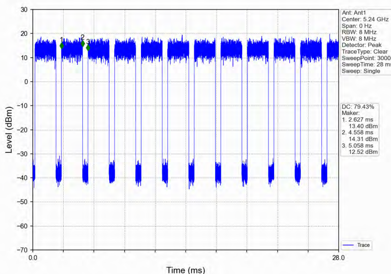
802.11ac(VHT20) HCH 5240MHz Ant1 NTVN
