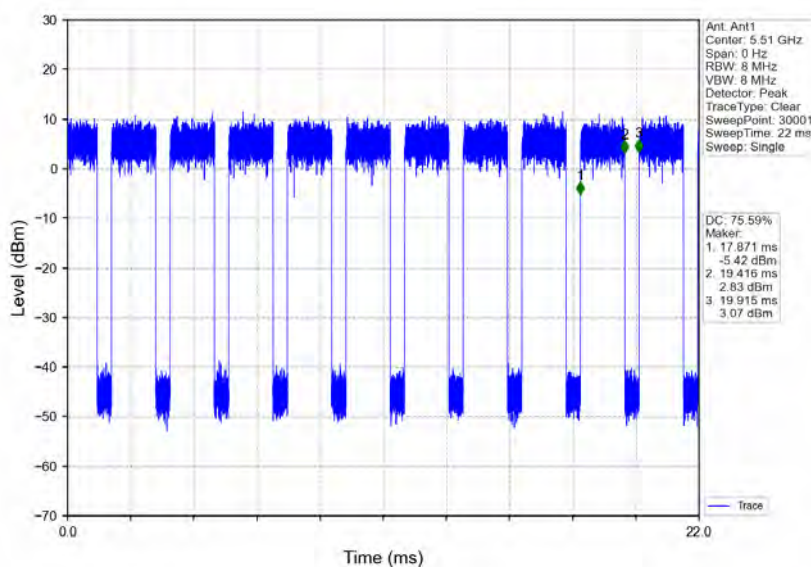
802.11ac(VHT40) LCH 5510MHz Ant1 NTV
