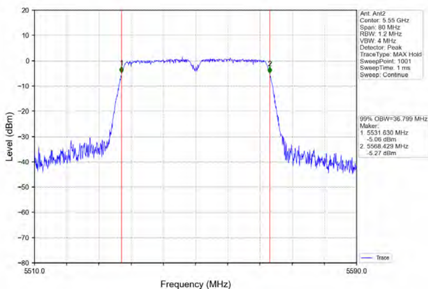
802.11ac(VHT40) MCH 5550MHz Ant2 NTV
