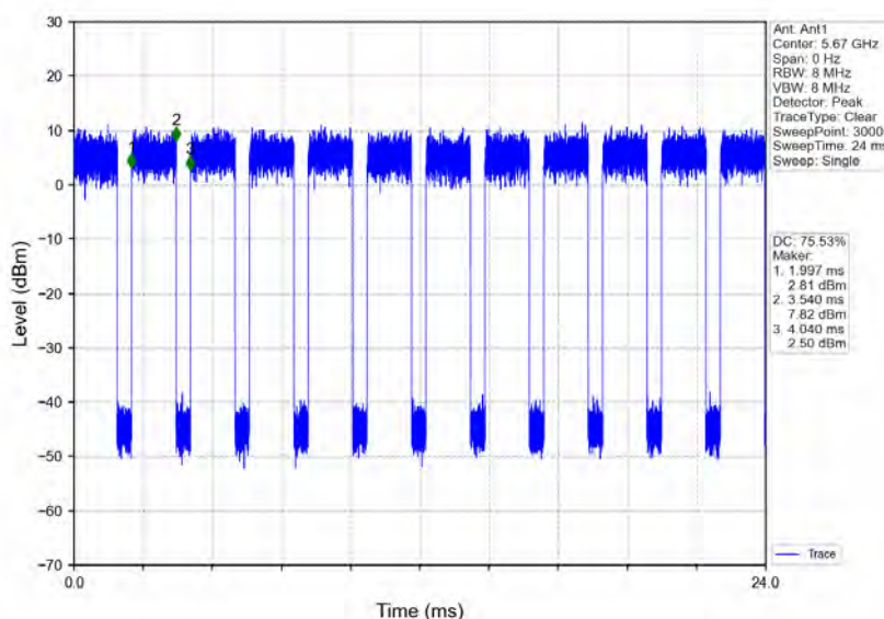
802.11ac(VHT40) HCH 5670MHz Ant1 NTVN
