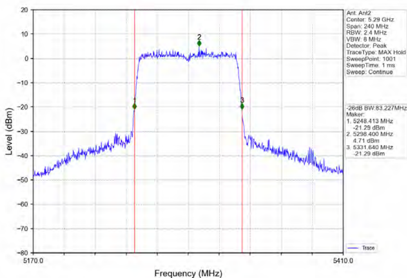
802.11ac(VHT80) MCH 5290MHz Ant2 NTV
