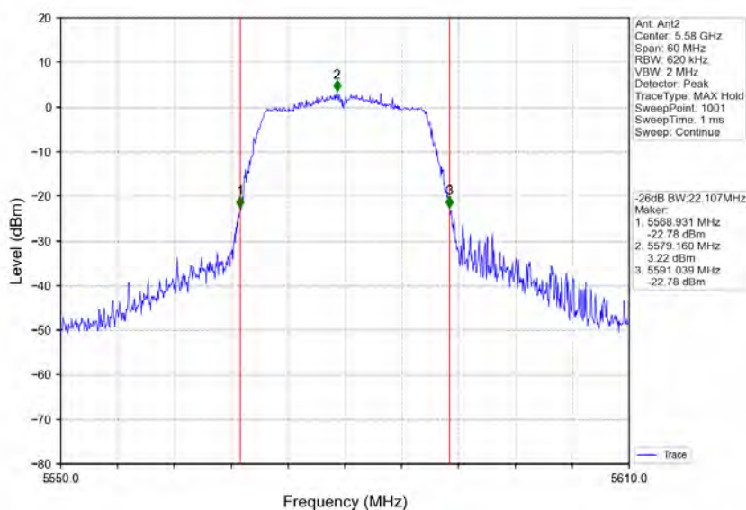
802.11ac(VHT20) MCH 5580MHz Ant2 NTVN
