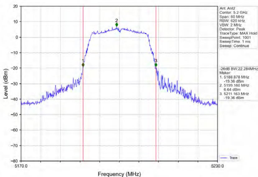
802.11ac(VHT20) MCH 5200MHz Ant2 NTV
