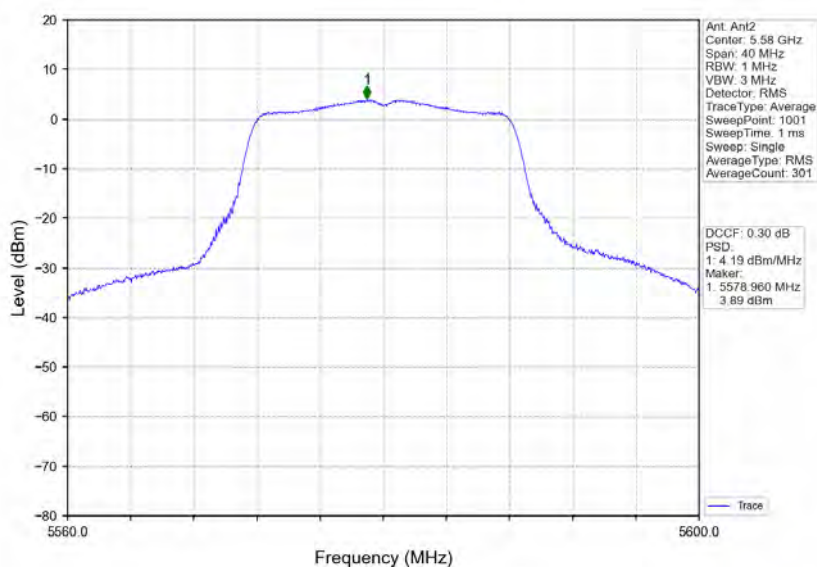
802.11a_MCH_5580MHz_Ant2_NTNV
