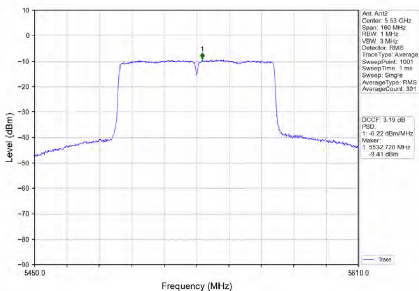
802.11ac(VHT80) LCH_5530MHz_Ant2_NTNV
