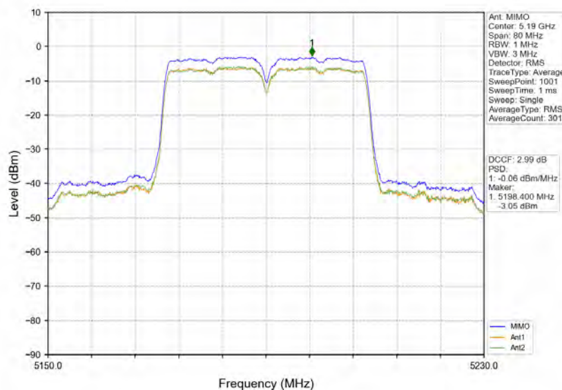
802.11n(HT40) LCH 5190MHz MIMO NTN
