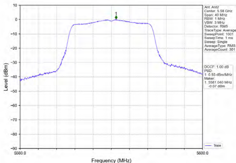
802.11ac(VHT20) MCH 5580MHz MIMO NTV
