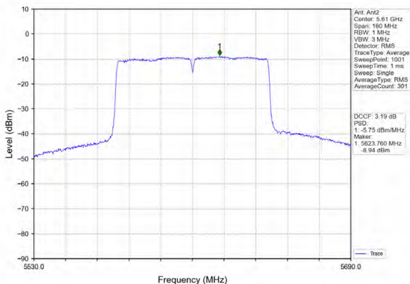
802.11ac(VHT80) HCH 5610MHz MIMO NTV
