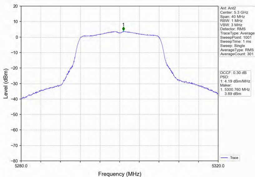
802.11a_MCH_5300MHz_Ant2_NTNV
