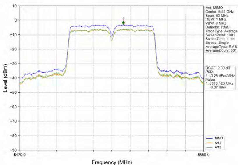
802.11n(HT40) LCH 5510MHz MIMO NTN
