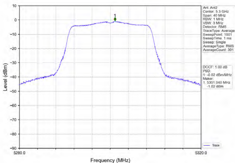
802.11ac(VHT20) MCH 5300MHz Ant2 NTVN
