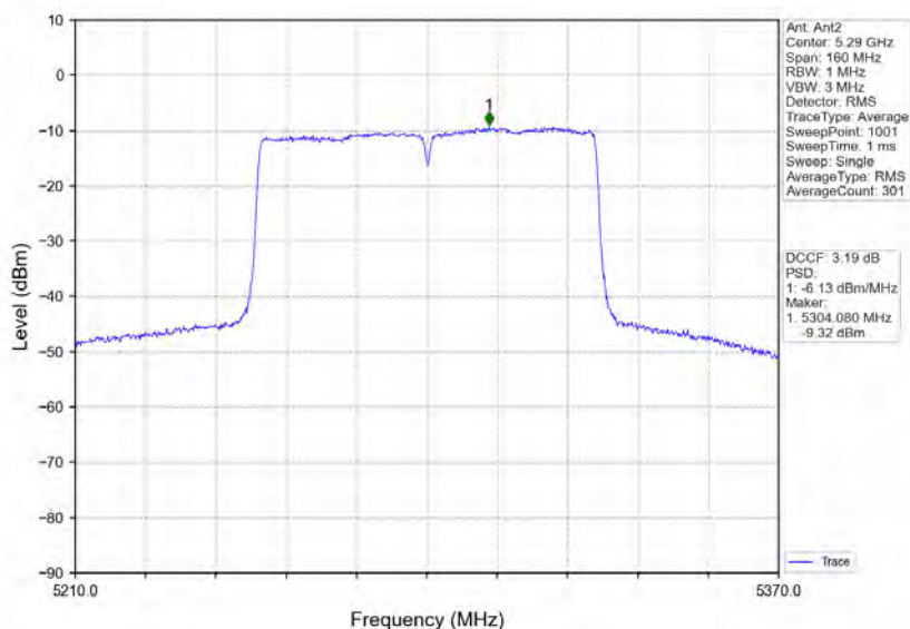
802.11ac(VHT80) MCH 5290MHz MIMO NTV
