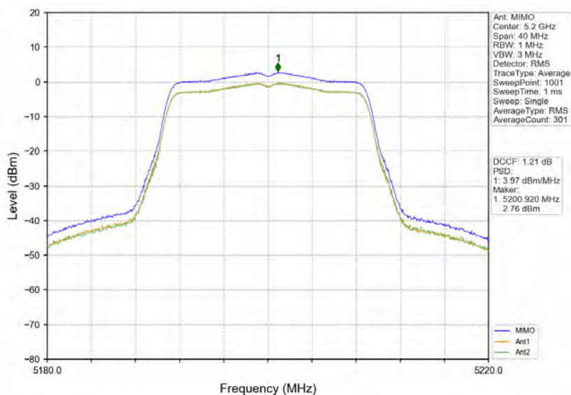
802.11ac(VHT20) MCH 5200MHz MIMO NTV
