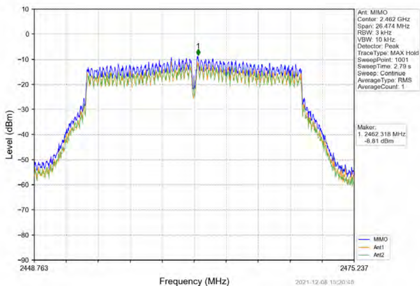
802.11n(HT20)_HCH_2462MHz_MIMO_NTNV
