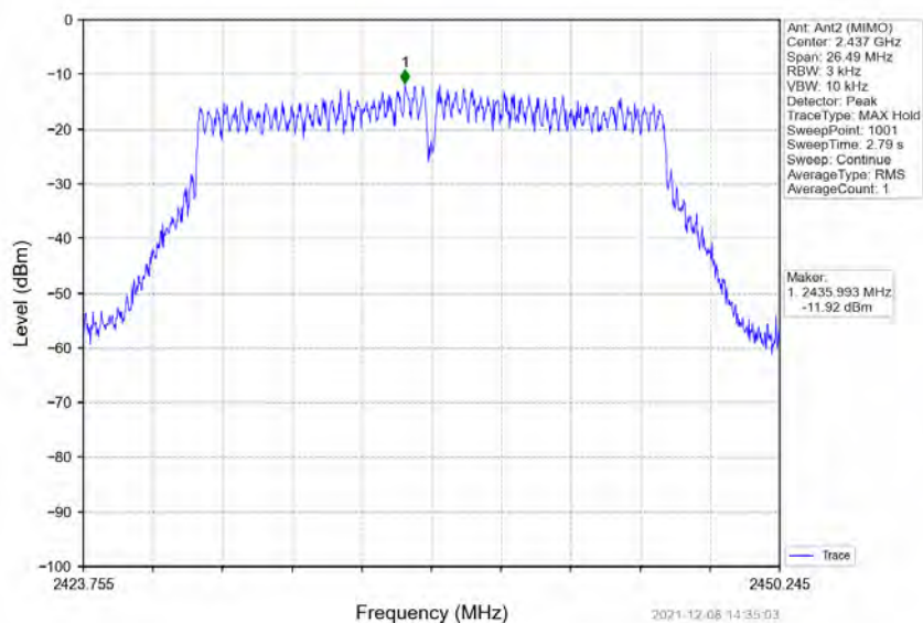
802.11n(HT20) MCH_2437MHz MIMO NTN
