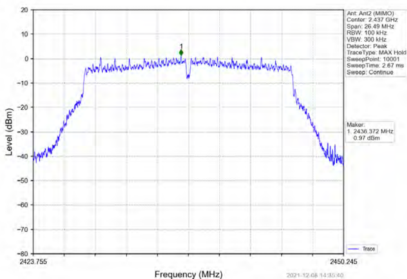
802.11n(HT20) MCH 2437MHz Ant2 (MIMO) NTV
