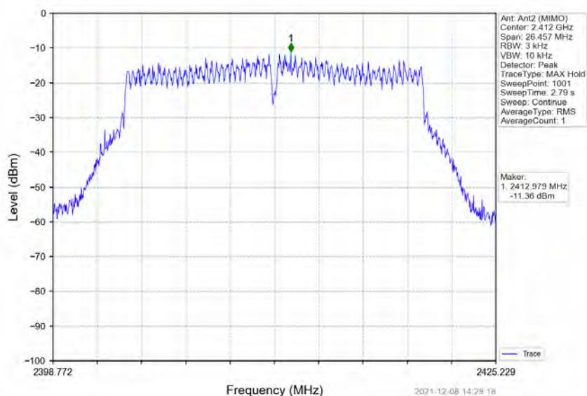
802.11n(HT20) LCH_2412MHz_MIMO_NTNV
