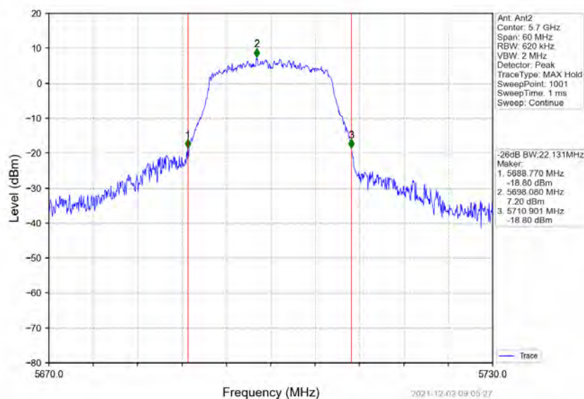
802.11a_HCH_5700MHz_Ant2_NTNV
