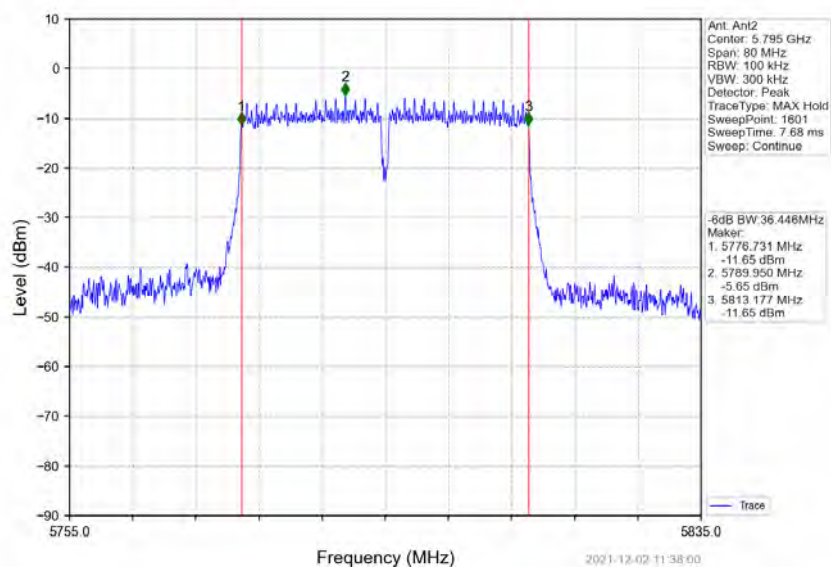
802.11n(HT40)_HCH_5795MHz_Ant2_NTNV
