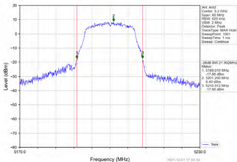
802.11a_MCH_5200MHz_Ant2_NTNV
