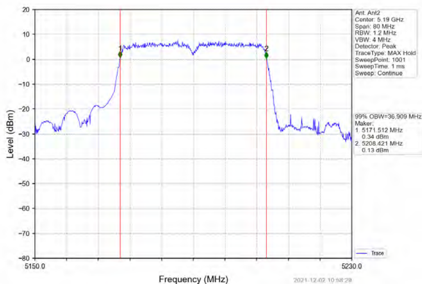
802.11n(HT40)_LCH_5190MHz_Ant2_NTNV
