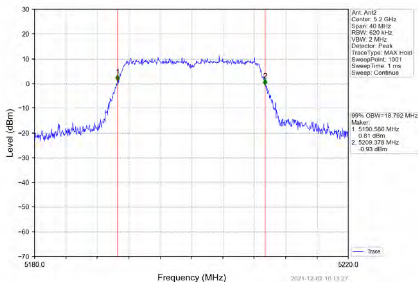
802.11n(HT20)_MCH_5200MHz_Ant2_NTNV
