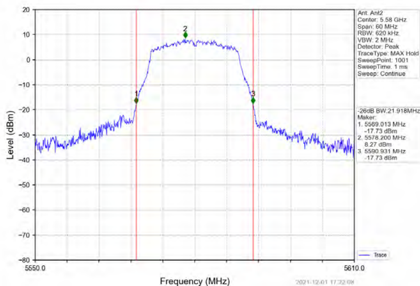
802.11a_MCH_5580MHz_Ant2_NTNV
