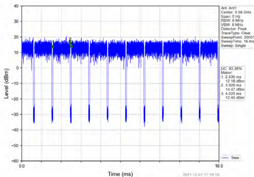
802.11a_MCH_5580MHz_Ant1_NTNV
