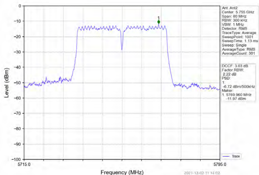
802.11n(HT40) LCH 5755MHz MIMO NTN
