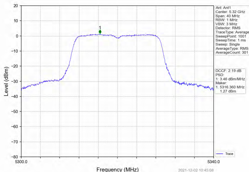
802.11n(HT20)_HCH_5320MHz_Ant1_NTNV
