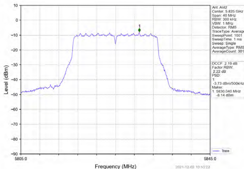
802.11n(HT20) HCH 5825MHz MIMO_NTNV
