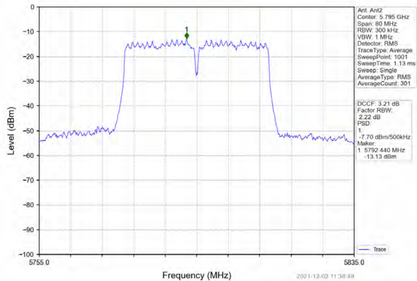
802.11n(HT40) HCH 5795MHz MIMO_NTNV
