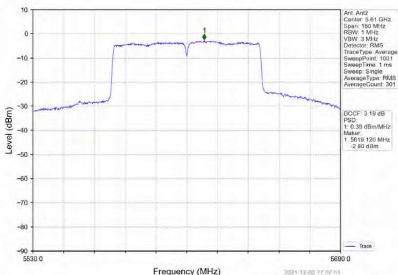
802.11ac(VHT80)_HCH_5610MHz_MIMO_NTNV
