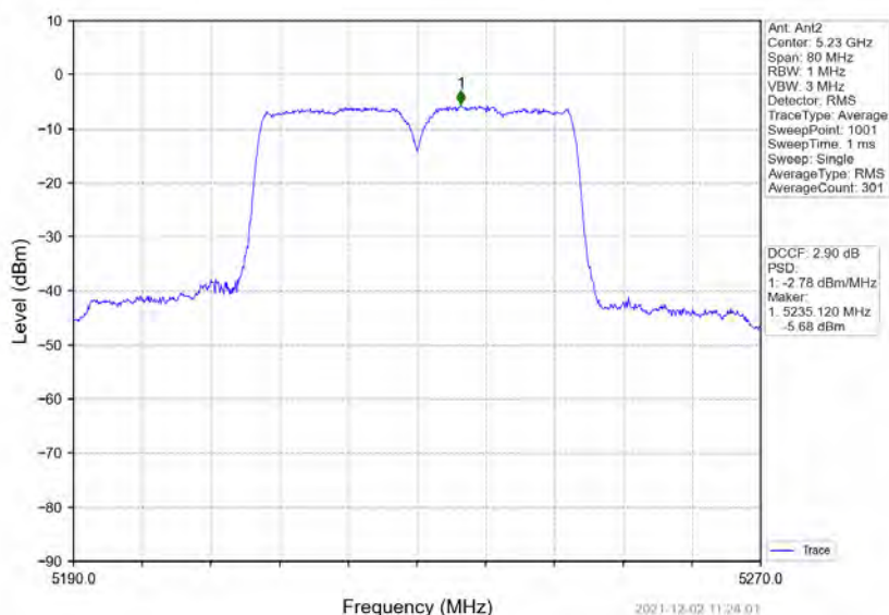
802.11n(HT40)_HCH_5230MHz_Ant2_NTNV
