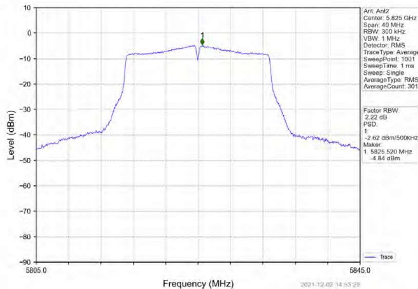
802.11ac(VHT20) HCH 5825MHz MIMO NTN
