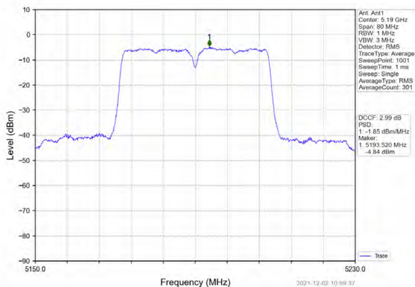
802.11n(HT40)_LCH_5190MHz_Ant1_NTNV
