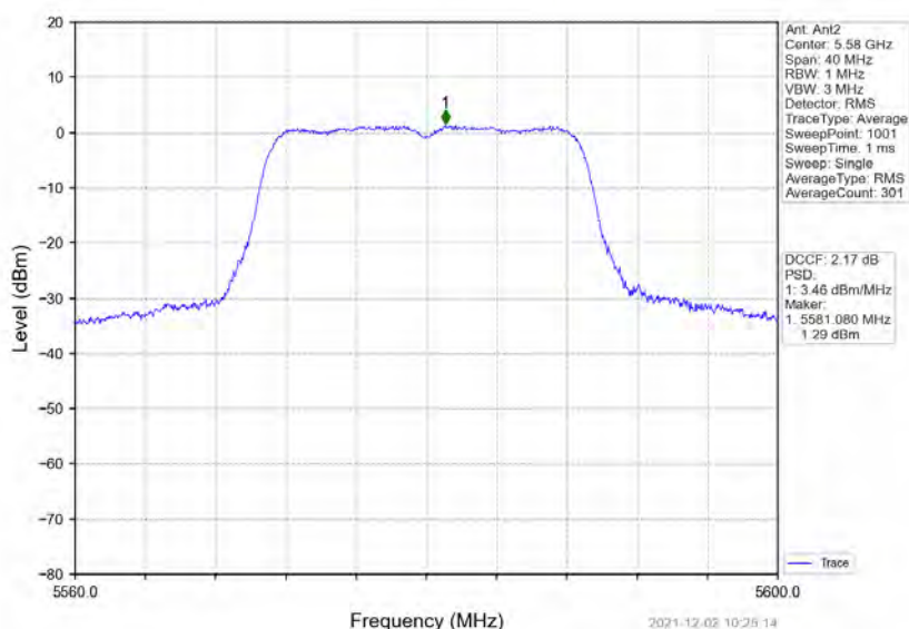
802.11n(HT20)_MCH_5580MHz_MIMO_NTNV
