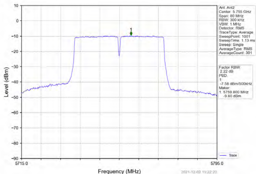
802.11ac(VHT40) LCH 5755MHz MIMO NTN
