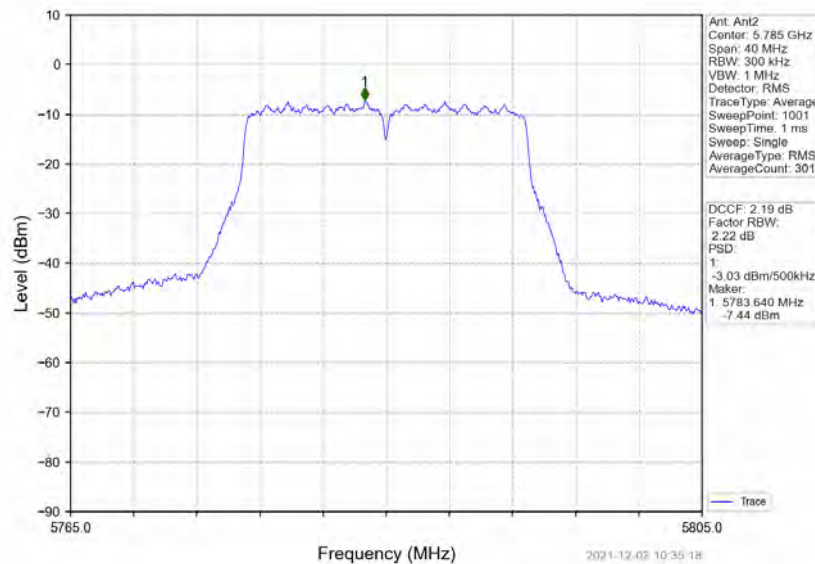
802.11n(HT20) MCH 5785MHz MIMO NTN
