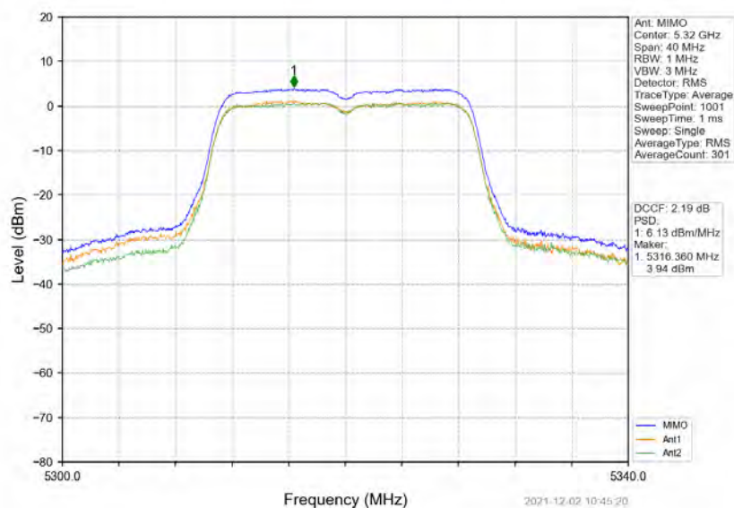
802.11n(HT20)_HCH_5320MHz_MIMO_NTNV
