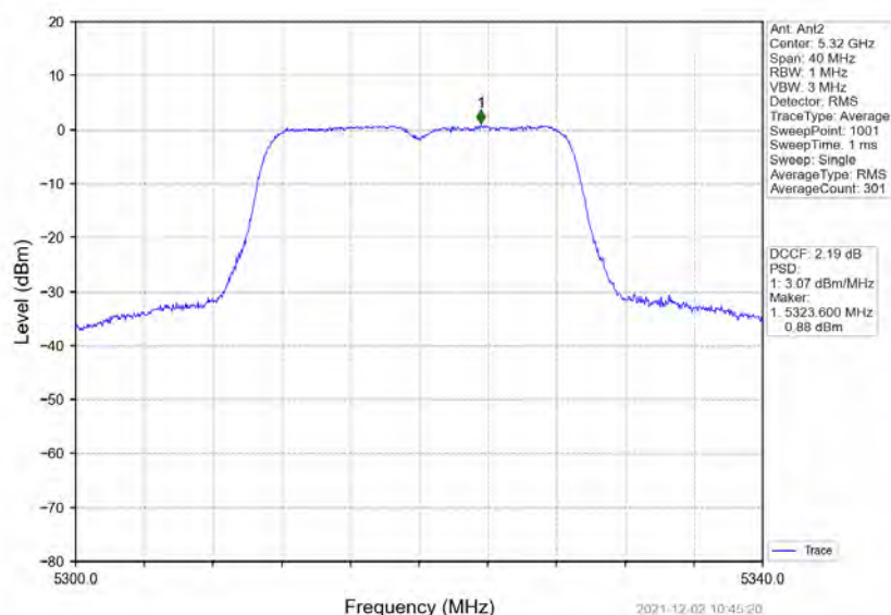
802.11n(HT20)_HCH_5320MHz_MIMO_NTNV
