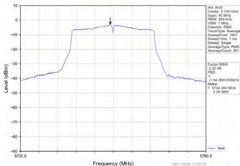
802.11ac(VHT20) LCH 5745MHz MIMO NTN
