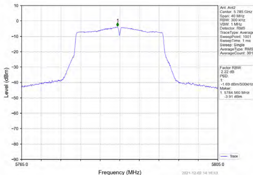
802.11ac(VHT20) MCH 5785MHz MIMO NTN
