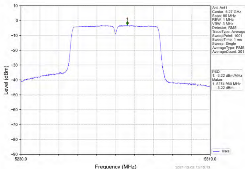
802.11ac(VHT40)_LCH_5270MHz_Ant1_NTNV
