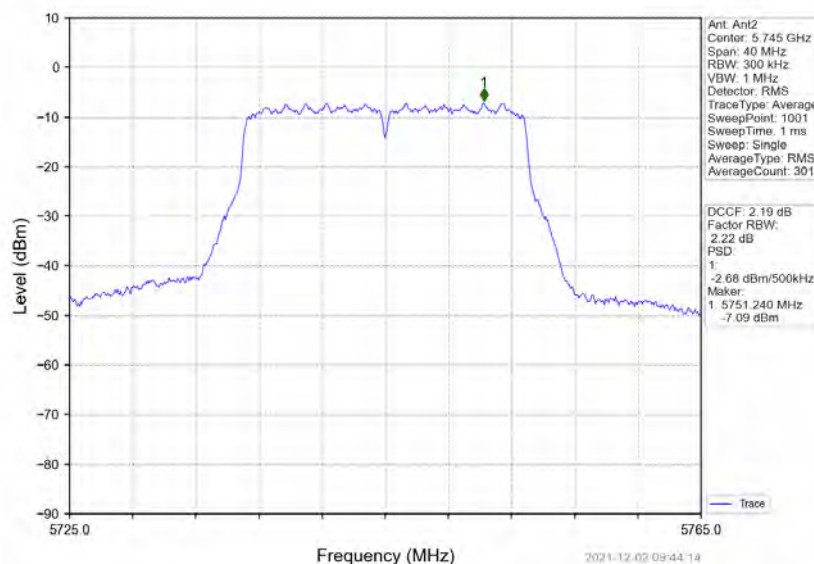
802.11n(HT20) LCH 5745MHz MIMO NTN
