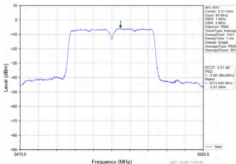
802.11n(HT40)_LCH_5510MHz_Ant1_NTNV
