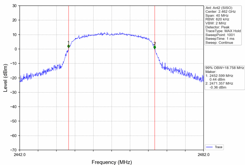
802.11n(HT20)_HCH_2462MHz_Ant2 (SISO)_NTNV
