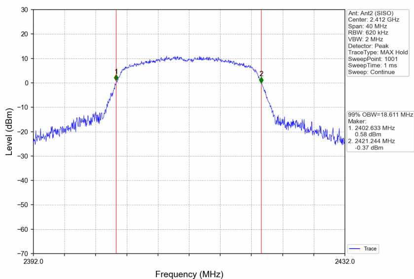
802.11n(HT20)_LCH_2412MHz_Ant2 (SISO)_NTNV
