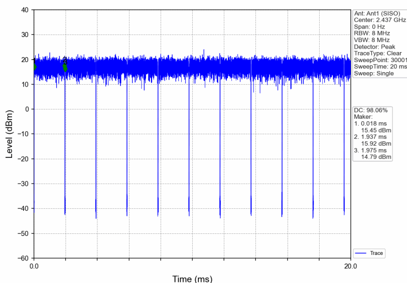
802.11n(HT20)_MCH_2437MHz_Ant1 (SISO)_NTNV
