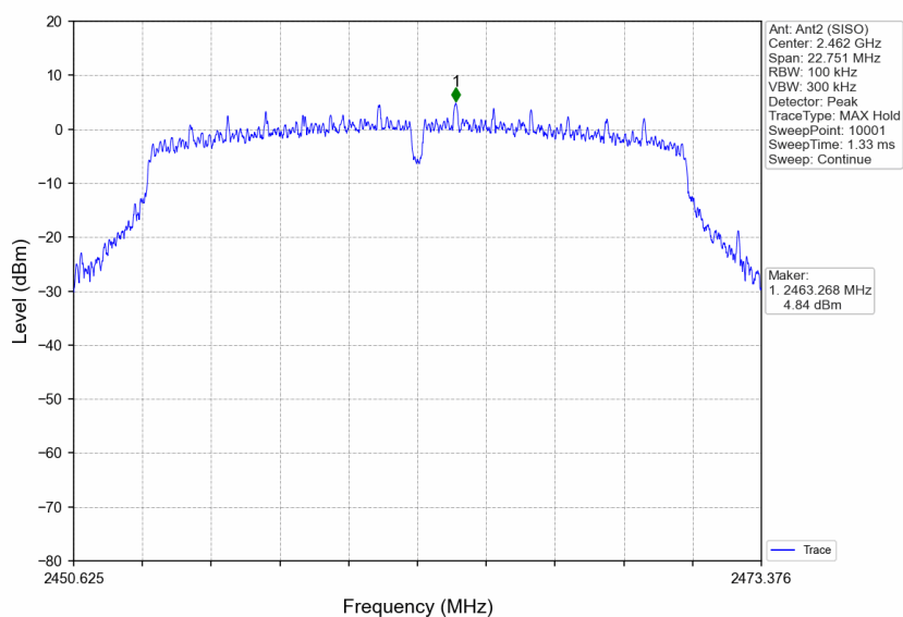
802.11n(HT20)_HCH_2462MHz_Ant2 (SISO)_NTNV
