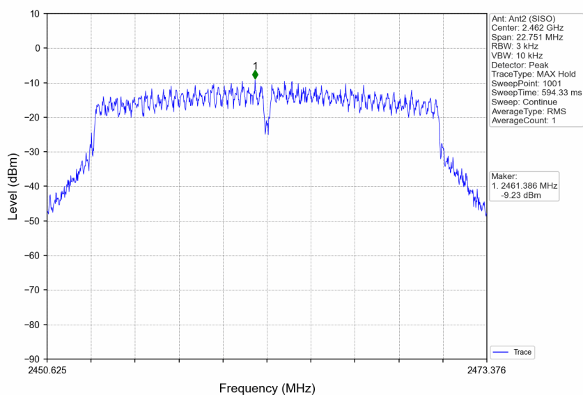
802.11n(HT20)_HCH_2462MHz_Ant2 (SISO)_NTNV
