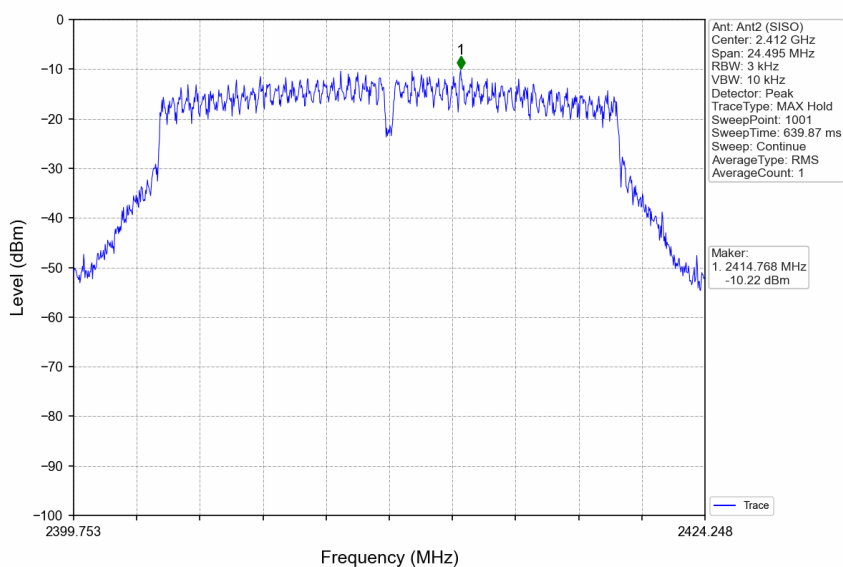
802.11n(HT20)_LCH_2412MHz_Ant2 (SISO)_NTNV
