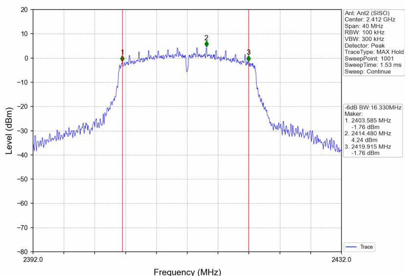
802.11n(HT20)_LCH_2412MHz_Ant2 (SISO)_NTNV
