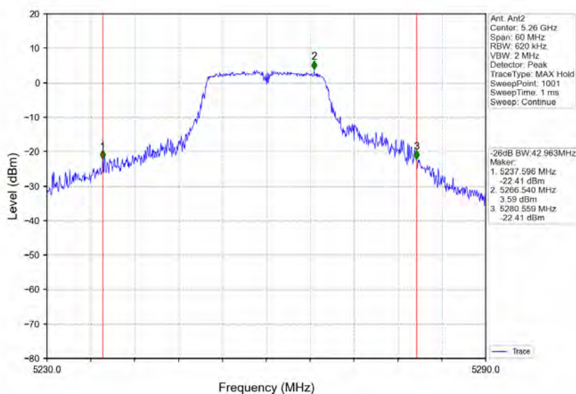
802.11a LCH_5260MHz_Ant2_NTNV
