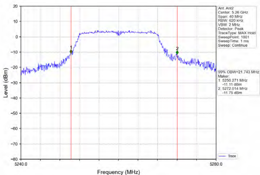
802.11a LCH_5260MHz_Ant2_NTNV
