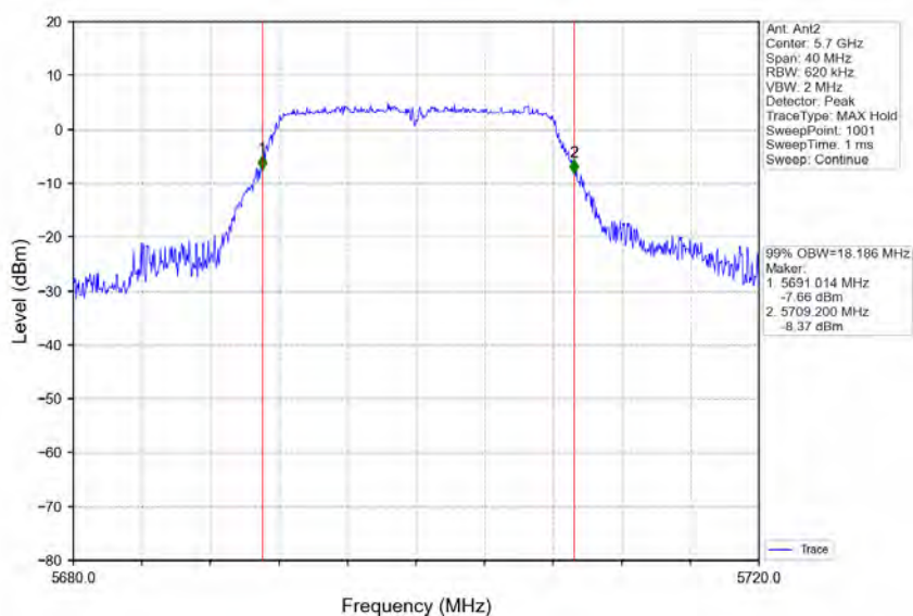
802.11a_HCH_5700MHz_Ant2_NTNV
