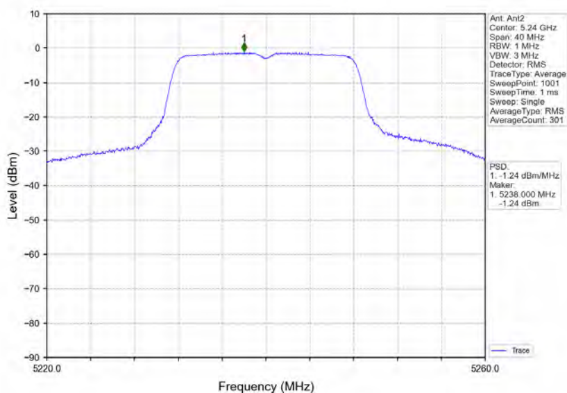
802.11a_HCH_5240MHz_Ant2_NTNV
