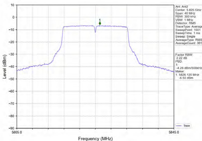
802.11a_HCH_5825MHz_Ant2_NTNV
