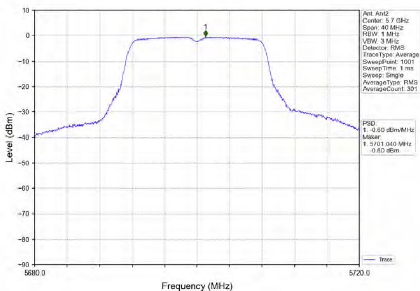
802.11a_HCH_5700MHz_Ant2_NTNV
