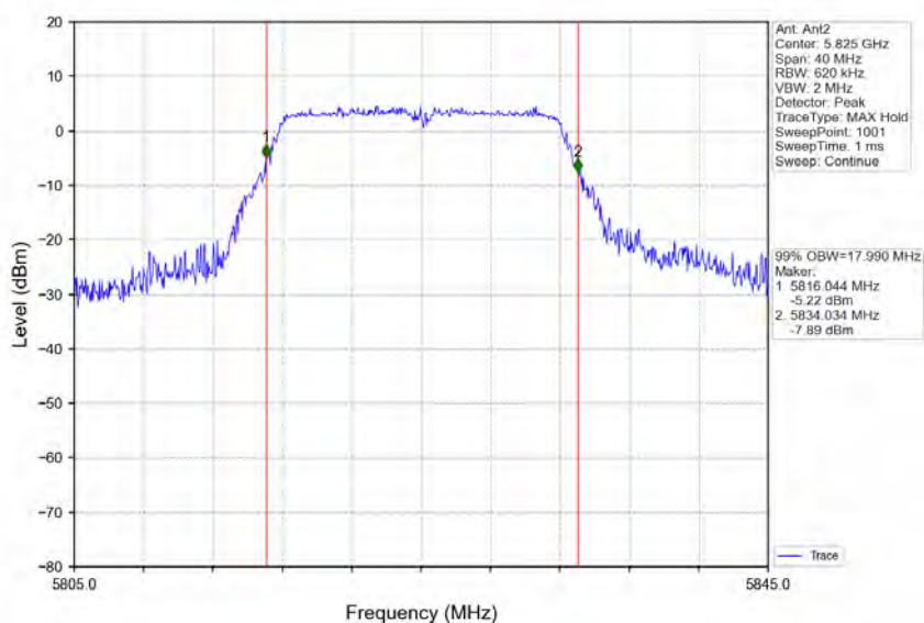
802.11a_HCH_5825MHz_Ant2_NTNV
