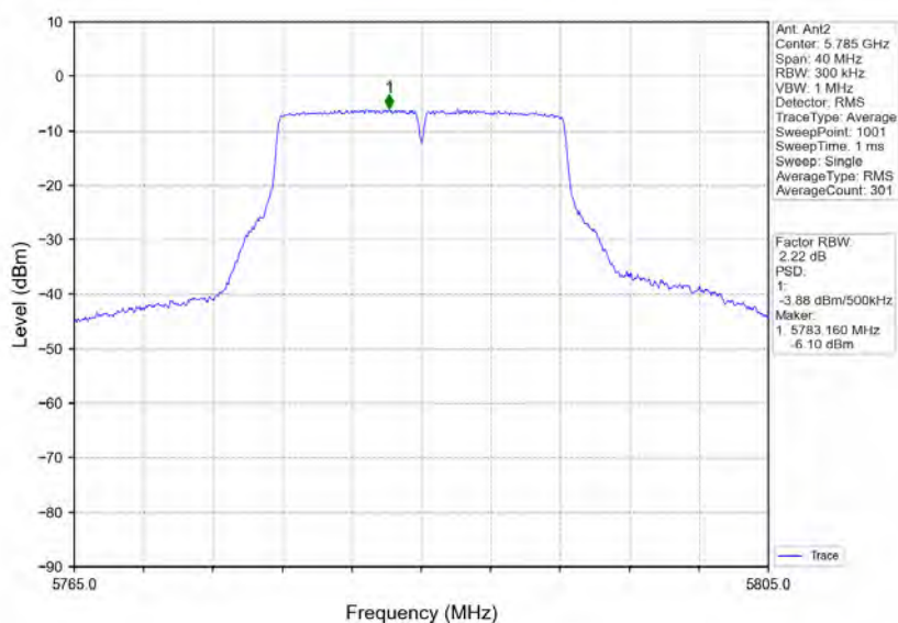
802.11a_MCH_5785MHz_Ant2_NTNV
