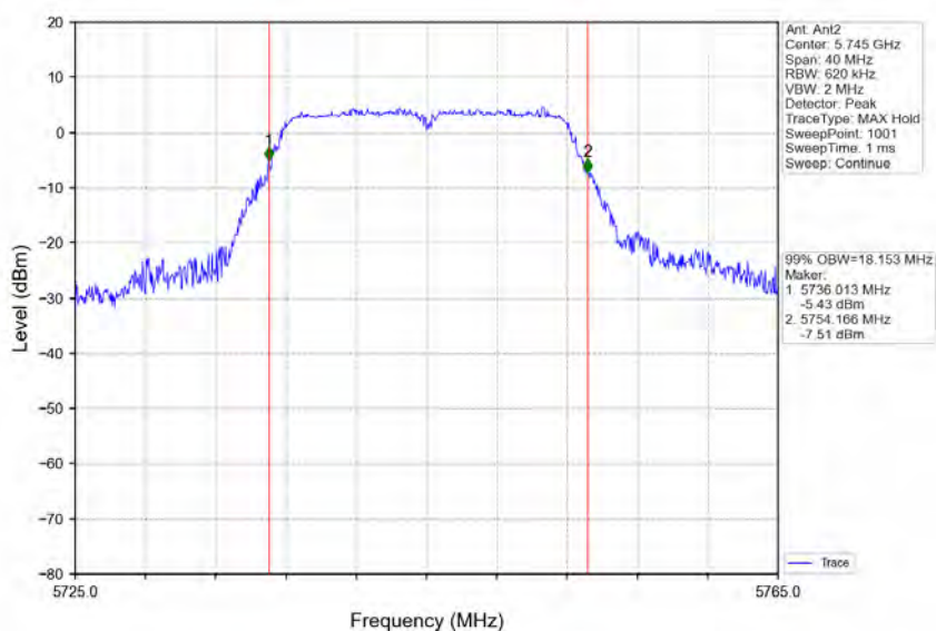
802.11a LCH_5745MHz_Ant2_NTNV
