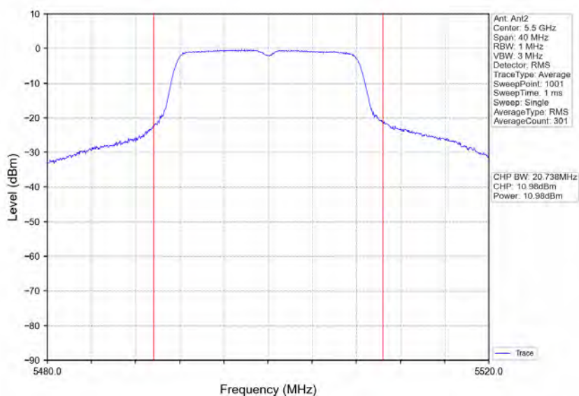
802.11a LCH_5500MHz_Ant2_NTNV
