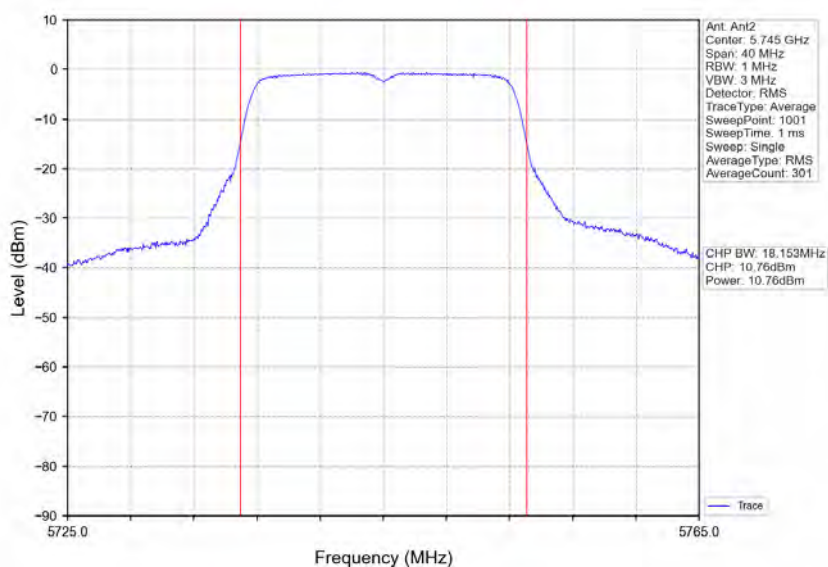
802.11a LCH_5745MHz_Ant2_NTNV
