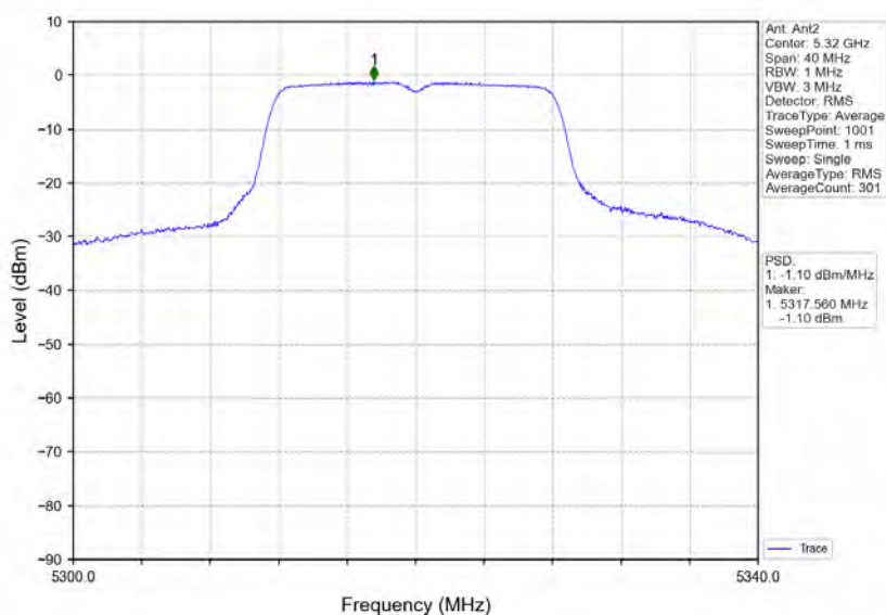
802.11a_HCH_5320MHz_Ant2_NTNV
