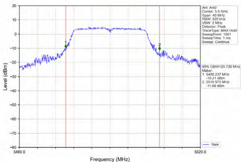
802.11a LCH_5500MHz_Ant2_NTNV
