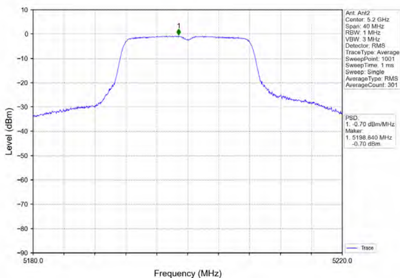
802.11a_MCH_5200MHz_Ant2_NTNV
