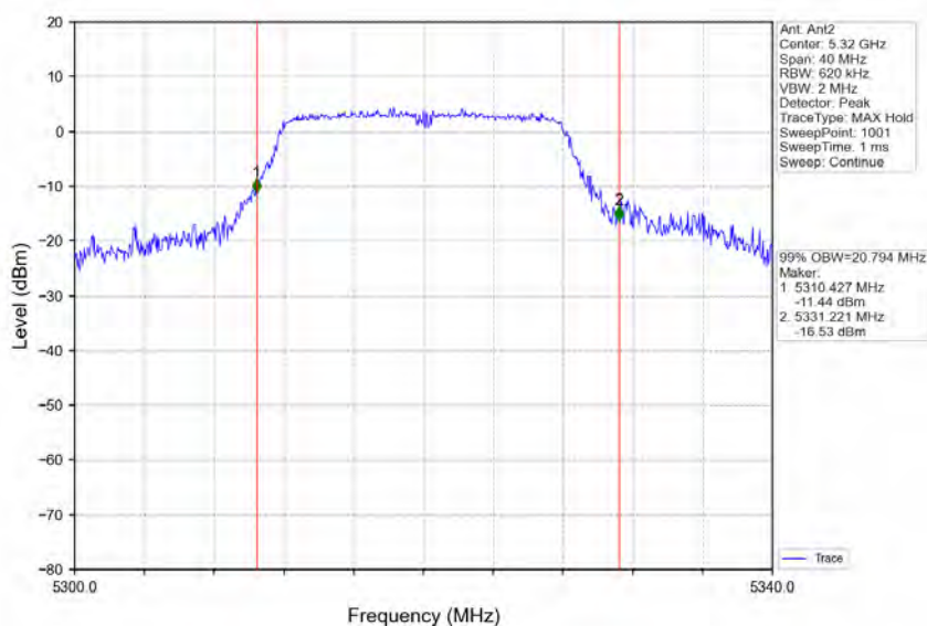
802.11a_HCH_5320MHz_Ant2_NTNV
