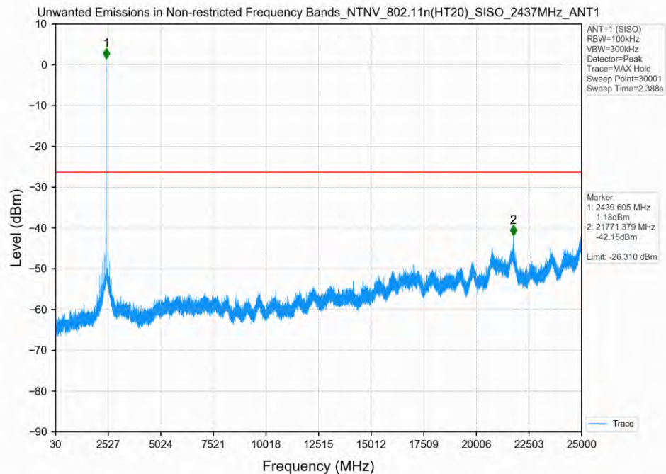
802.11n(HT20)_2437MHz_SISO_ANT1
