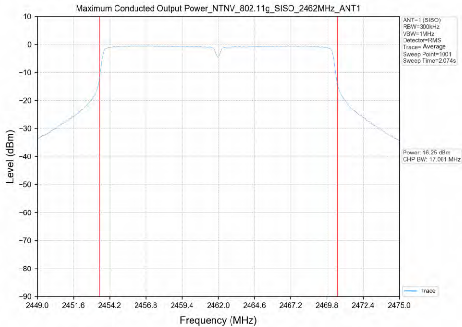
802.11g 2462MHz SISO ANT1
