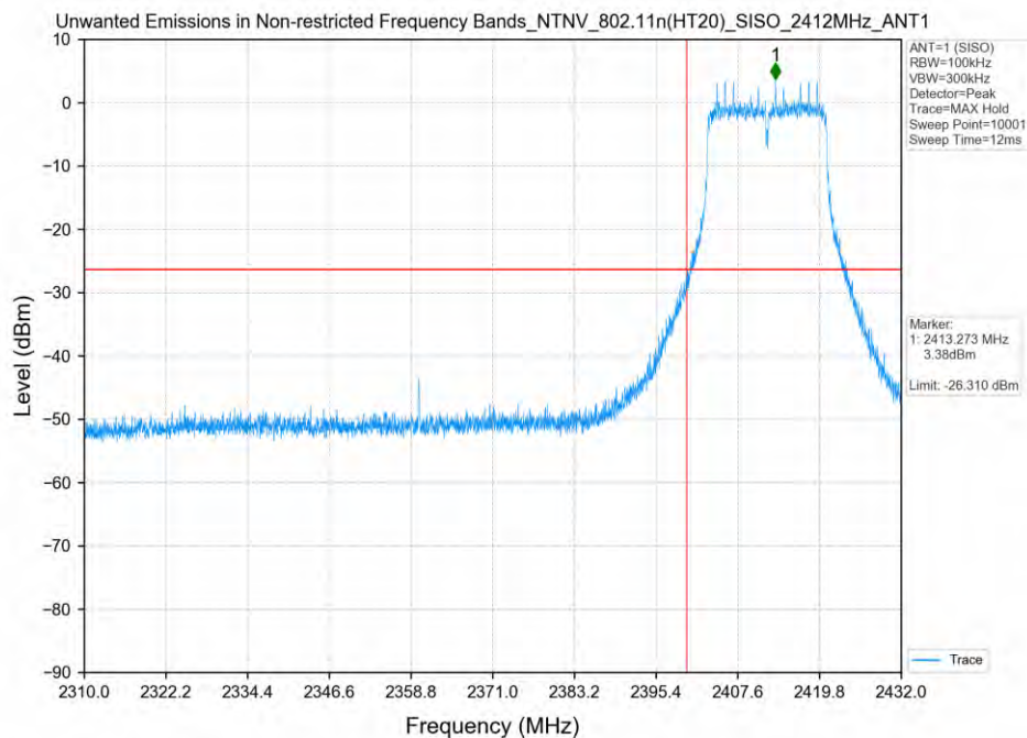
802.11n(HT20)_2412MHz_SISO_ANT1
