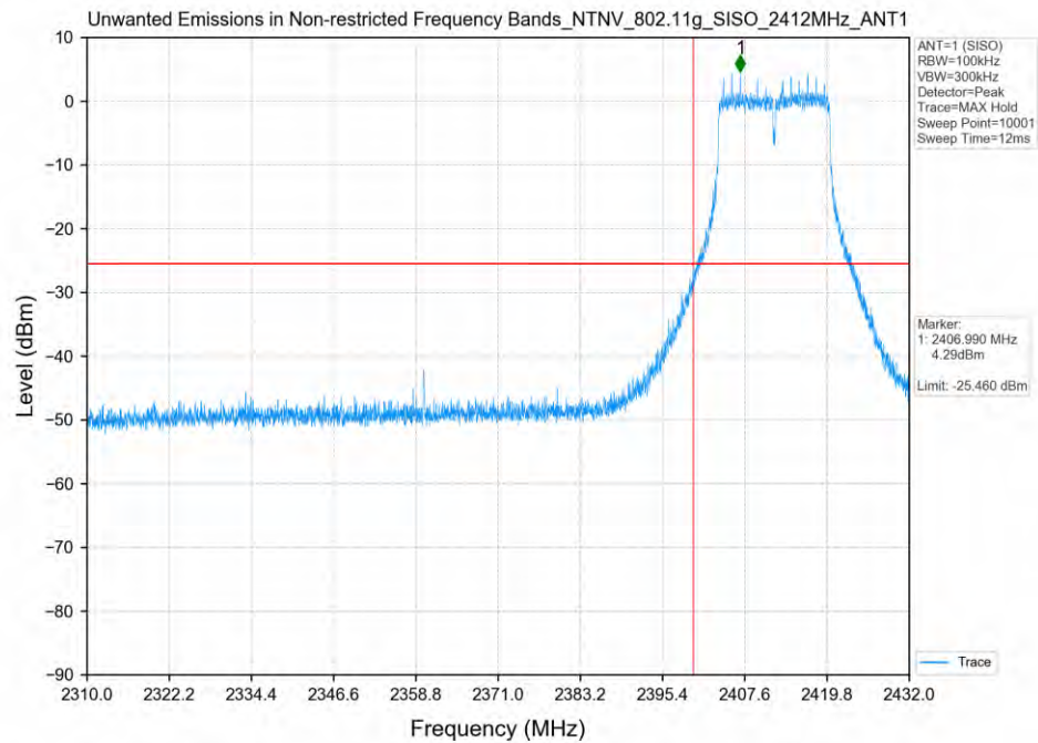
802.11g_2412MHz_SISO_ANT1
