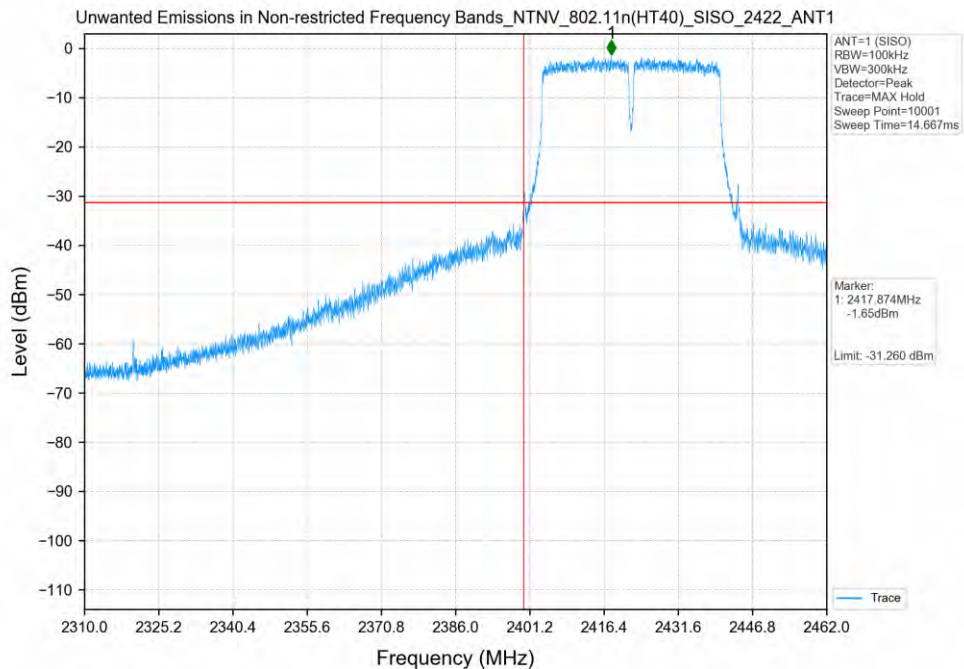
802.11n(HT40)_2422MHz_SISO_ANT1
