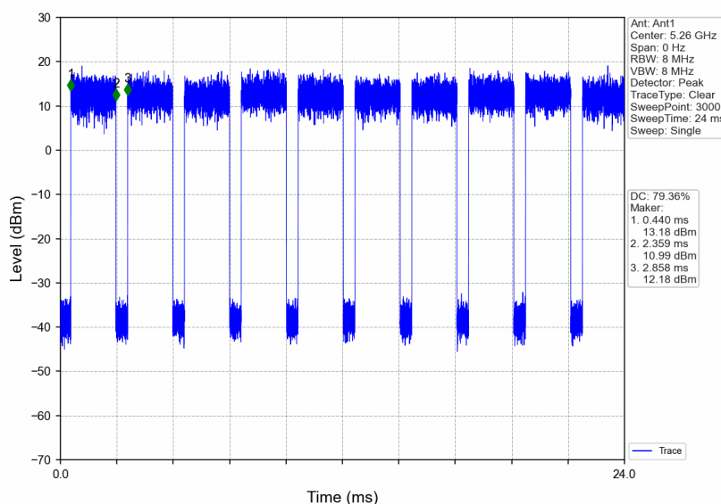
802.11n(HT20)_LCH_5260MHz_Ant1_NTNV
