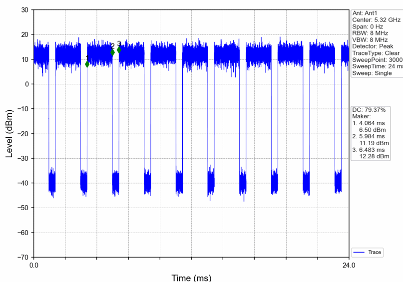
802.11n(HT20)_HCH_5320MHz_Ant1_NTNV
