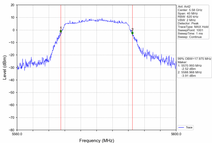
802.11a_MCH_5580MHz_Ant2_NTNV
