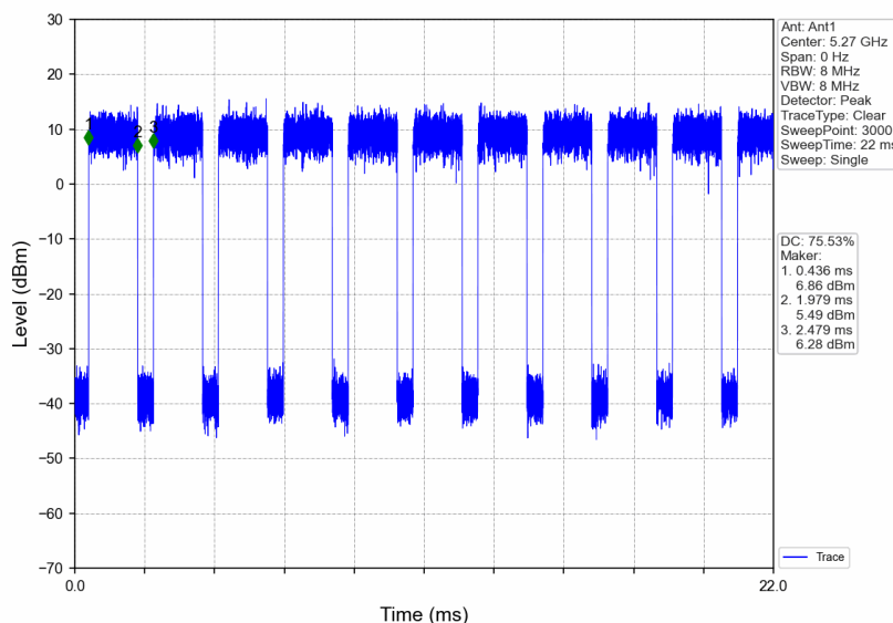
802.11ac(VHT40) LCH_5270MHz_Ant1_NTNV
