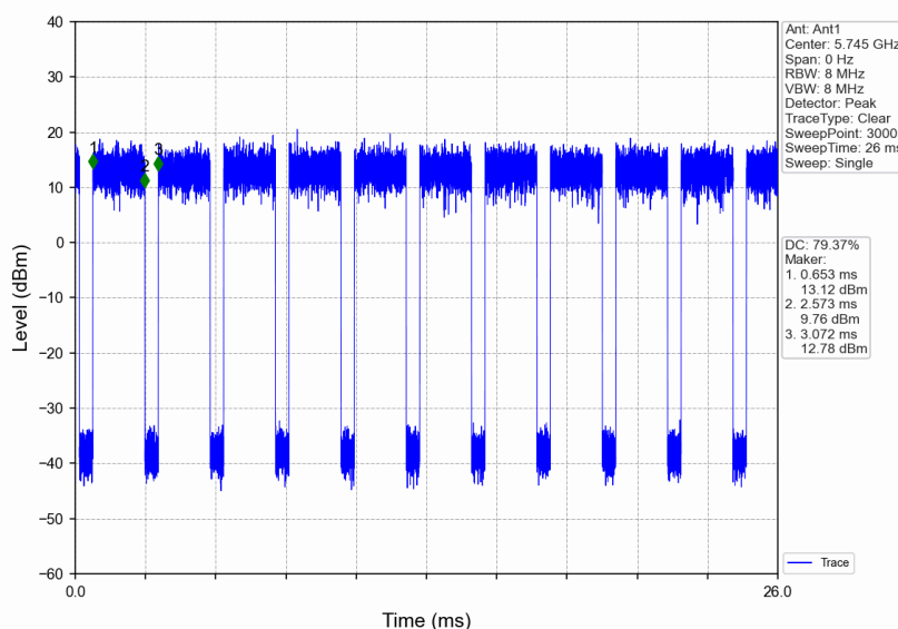
802.11n(HT20)_LCH_5745MHz_Ant1_NTNV
