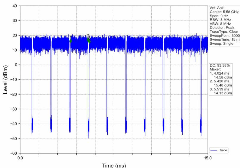
802.11a_MCH_5580MHz_Ant1_NTNV
