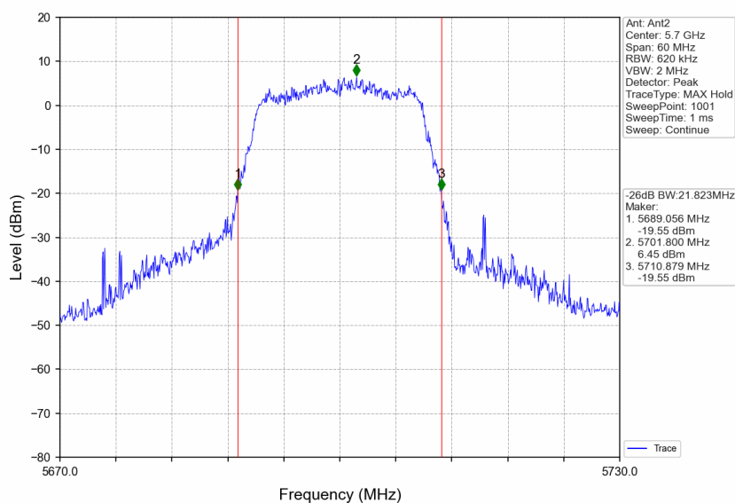
802.11n(HT20)_HCH_5700MHz_Ant2_NTNV
