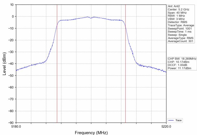
802.11n(HT20)_MCH_5200MHz_Ant2_NTNV
