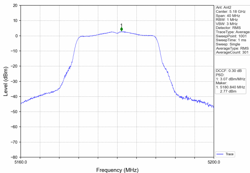
802.11a_LCH_5180MHz_Ant2_NTNV
