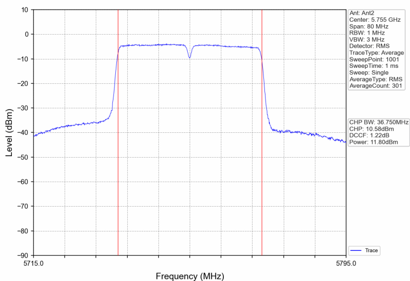
802.11ac(VHT40) LCH_5755MHz_Ant2_NTNV
