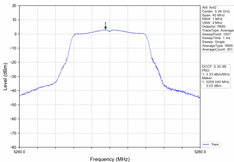
802.11a LCH_5260MHz_Ant2_NTNV
