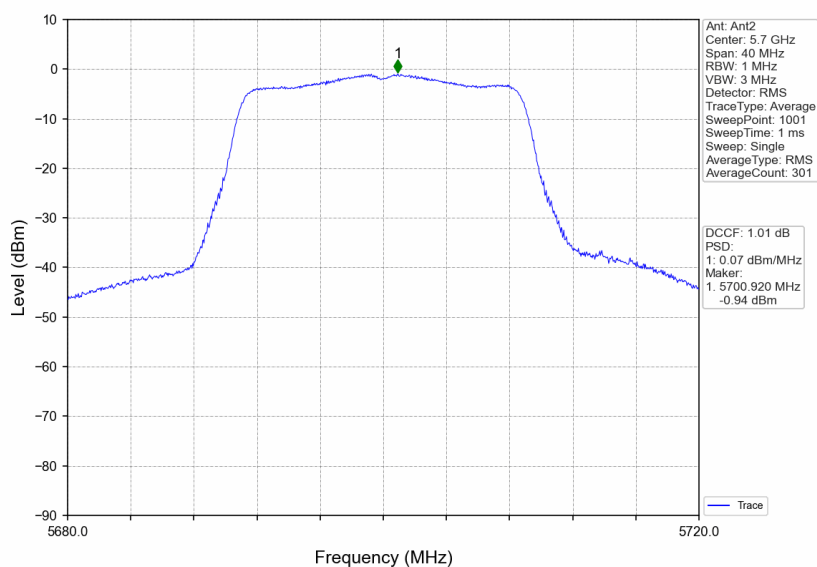
802.11n(HT20)_HCH_5700MHz_Ant2_NTNV
