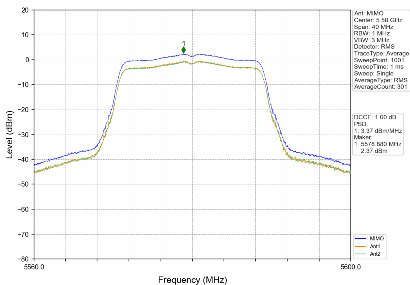
802.11n(HT20)_MCH_5580MHz_MIMO_NTNV
