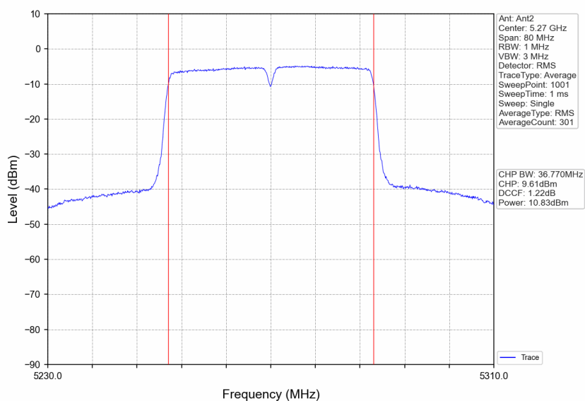
802.11ac(VHT40) LCH_5270MHz_Ant2_NTNV
