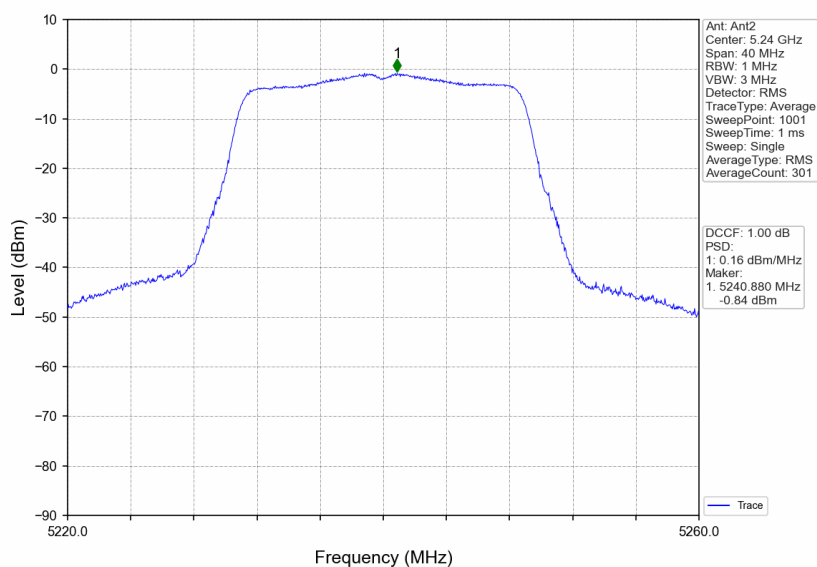
802.11ac(VHT20) HCH 5240MHz Ant2 NTV
