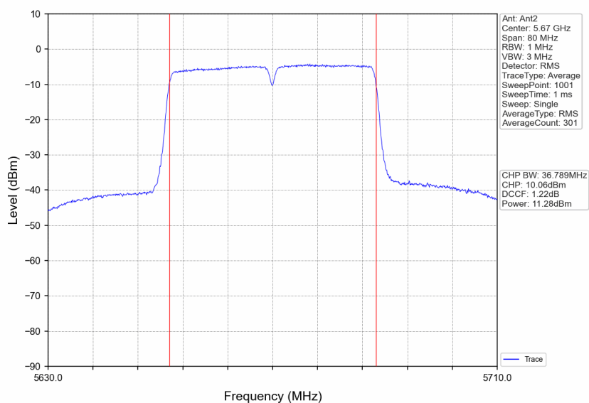
802.11ac(VHT40) HCH 5670MHz Ant2 NTNV
