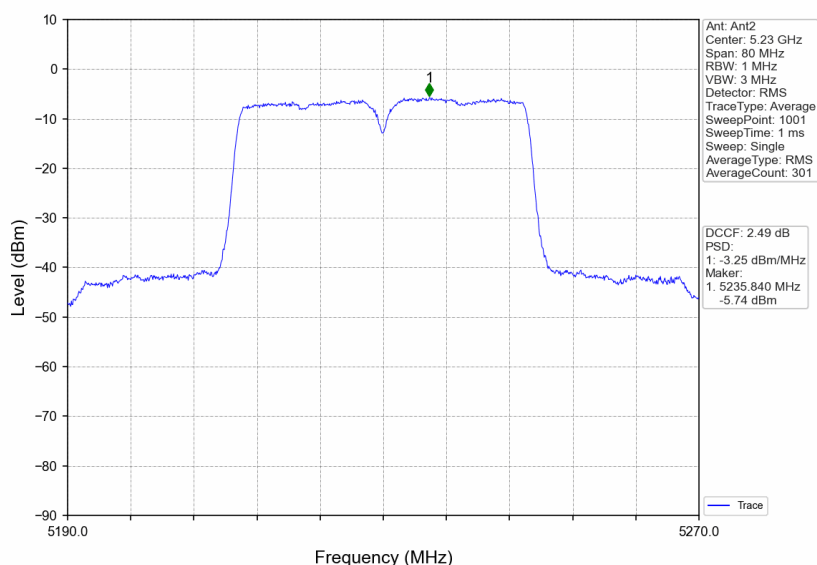
802.11n(HT40) HCH 5230MHz_Ant2_NTNV
