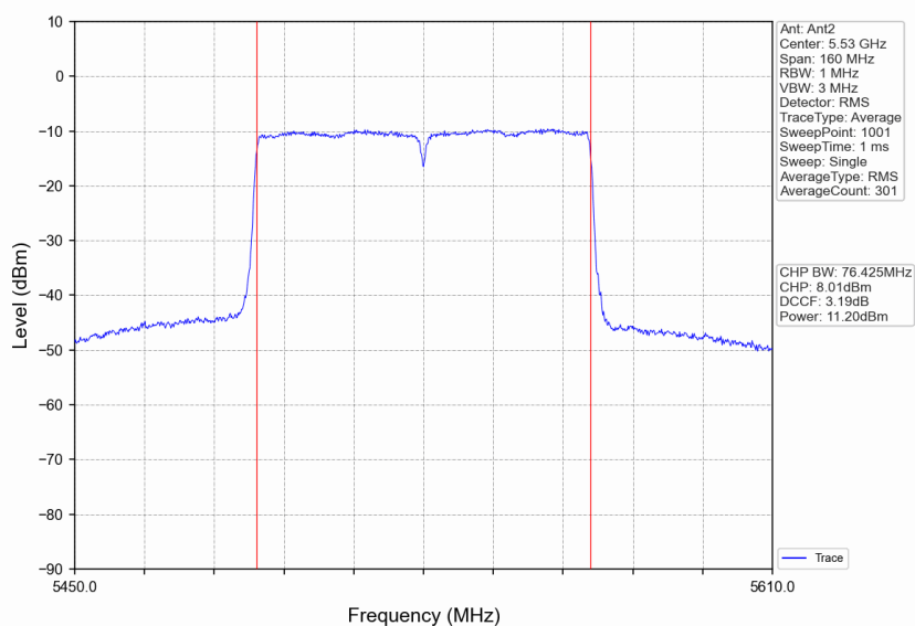
802.11ac(VHT80) LCH_5530MHz_Ant2_NTNV
