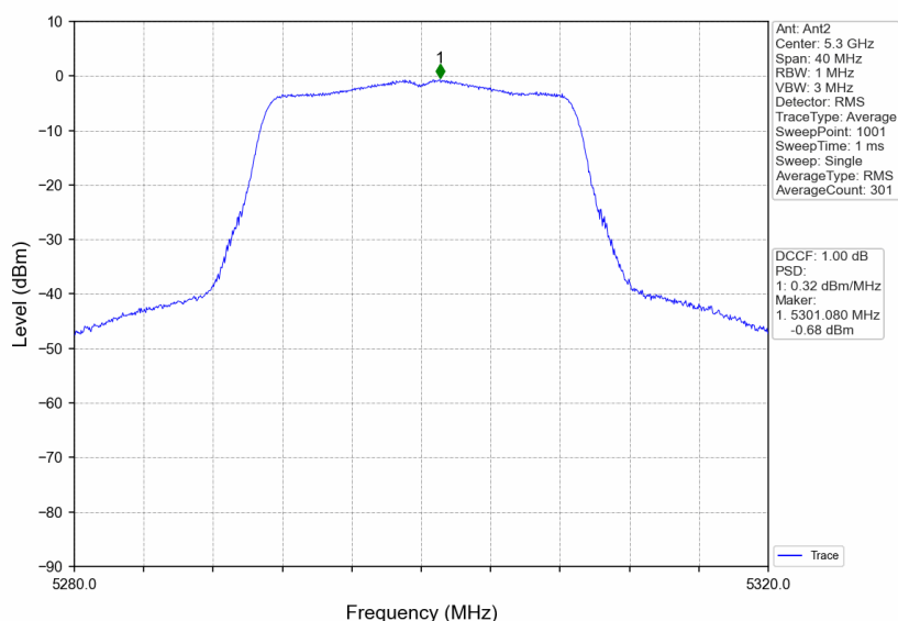
802.11ac(VHT20) MCH 5300MHz_Ant2_NTNV
