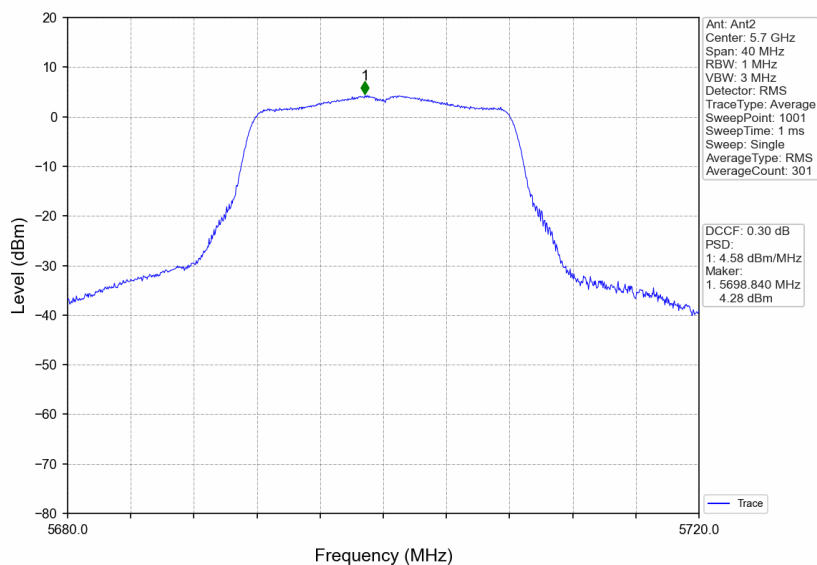
802.11a_HCH_5700MHz_Ant2_NTNV
