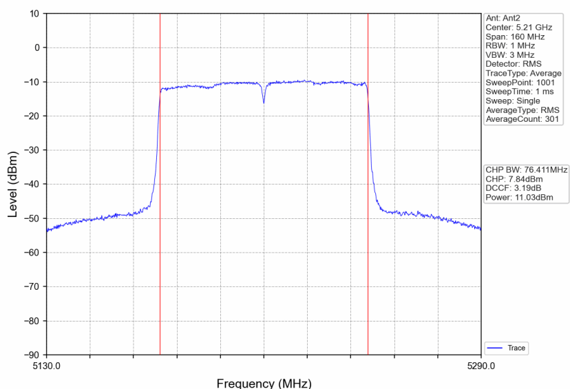
802.11ac(VHT80) MCH 5210MHz Ant2 NTVN
