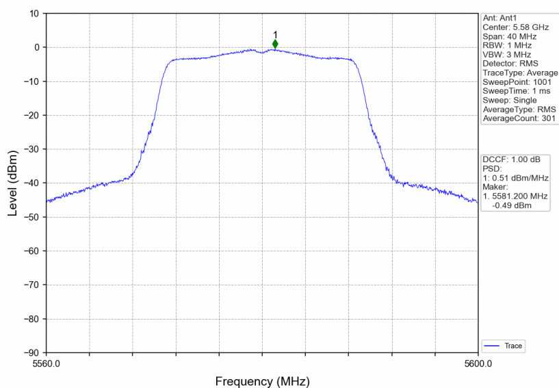
802.11n(HT20)_MCH_5580MHz_Ant1_NTNV
