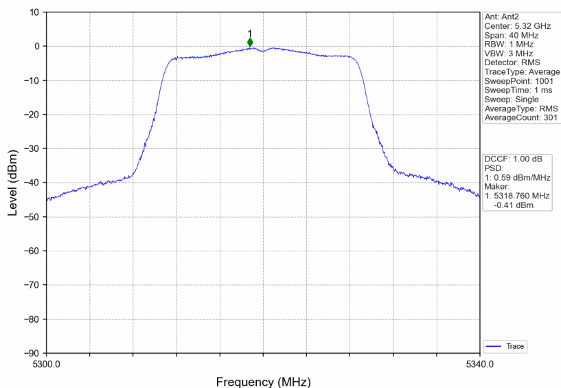
802.11n(HT20)_HCH_5320MHz_MIMO_NTNV
