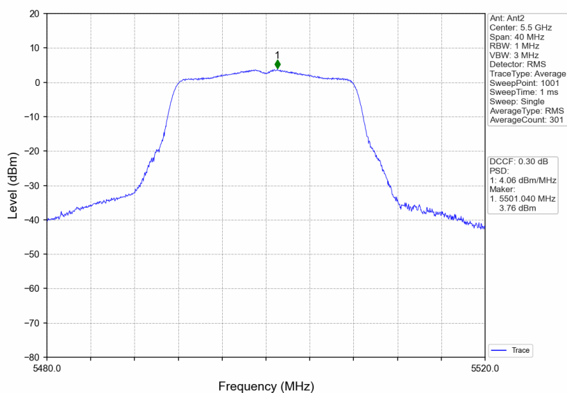
802.11a LCH_5500MHz_Ant2_NTNV
