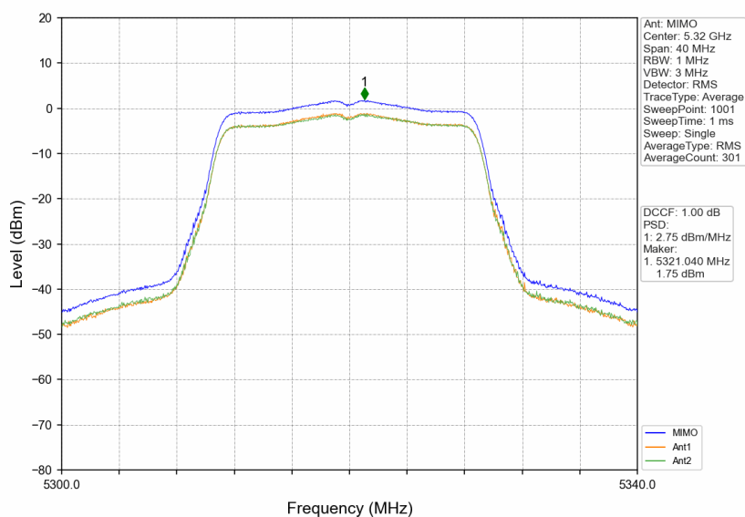
802.11ac(VHT20) HCH_5320MHz_MIMO_NTNV
