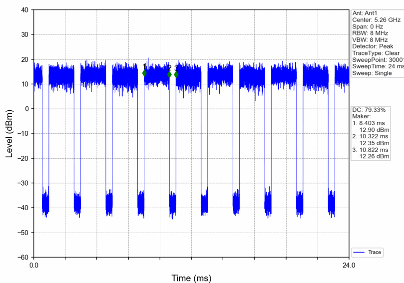
802.11n(HT20)_LCH_5260MHz_Ant1_NTNV
