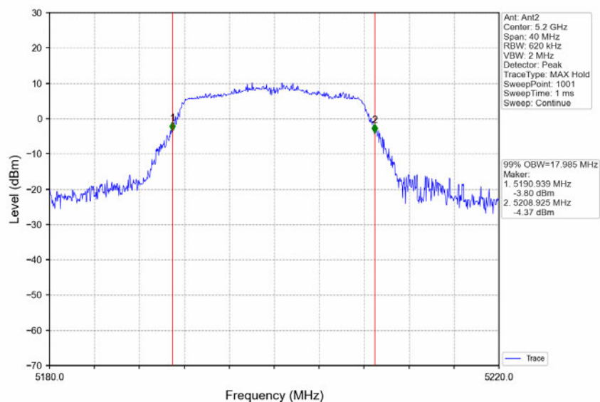
802.11a_MCH_5200MHz_Ant2_NTNV
