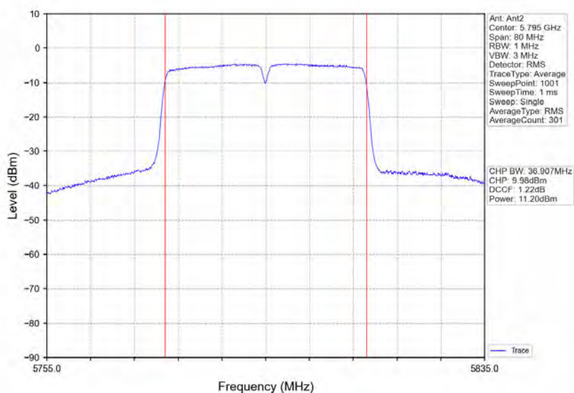
802.11ac(VHT40) HCH 5795MHz Ant2 NTV
