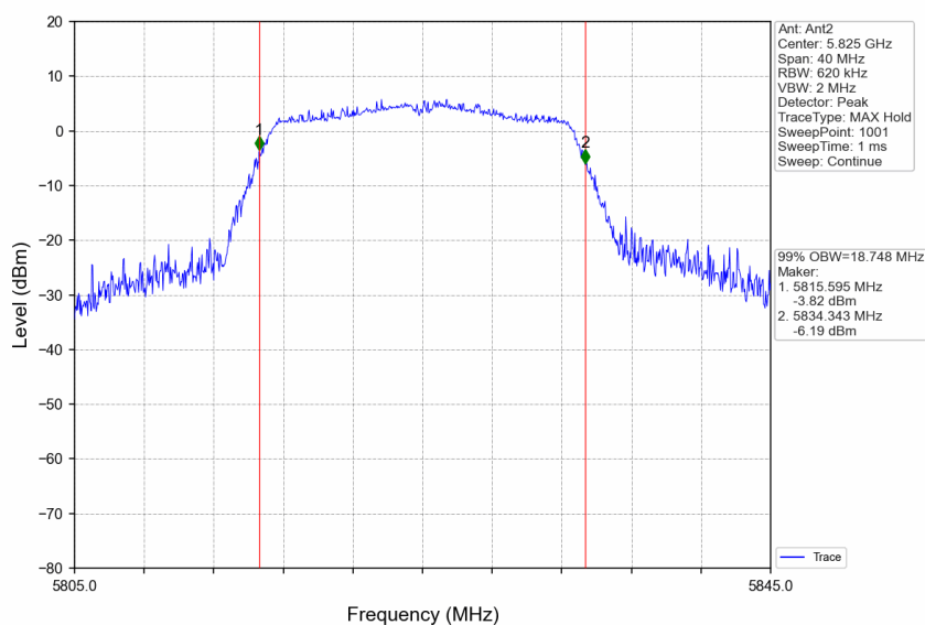
802.11ac(VHT20) HCH 5825MHz Ant2 NTNV
