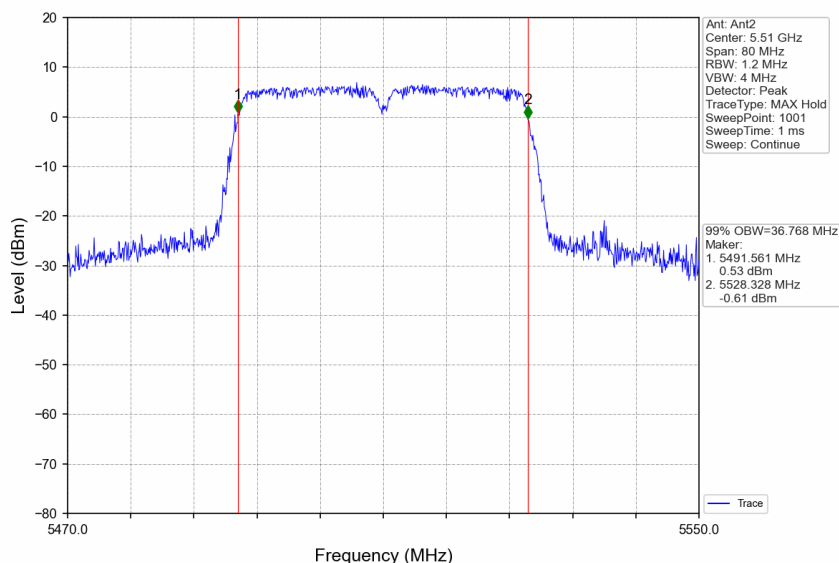
802.11ac(VHT40) LCH_5510MHz_Ant2_NTNV
