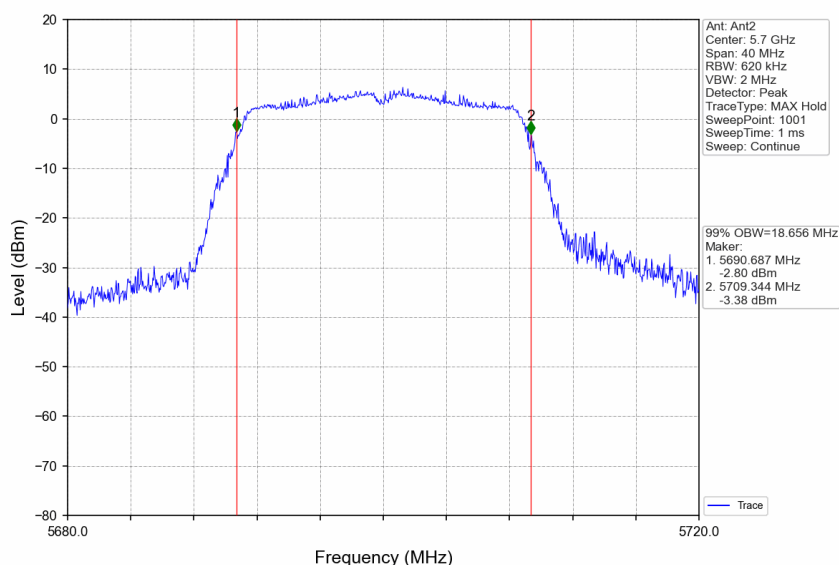
802.11n(HT20)_HCH_5700MHz_Ant2_NTNV
