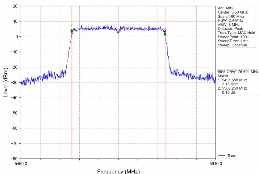
802.11ac(VHT80) LCH_5530MHz_Ant2_NTNV
