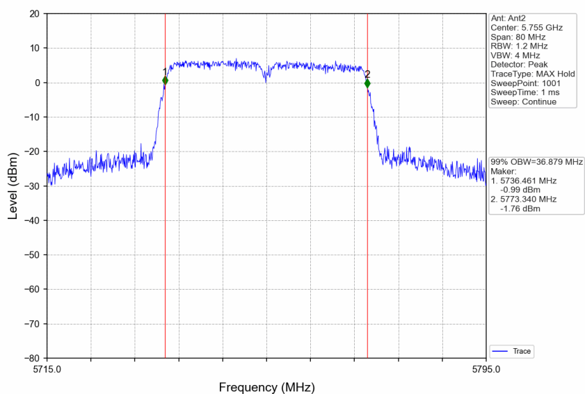
802.11ac(VHT40) LCH_5755MHz_Ant2_NTNV
