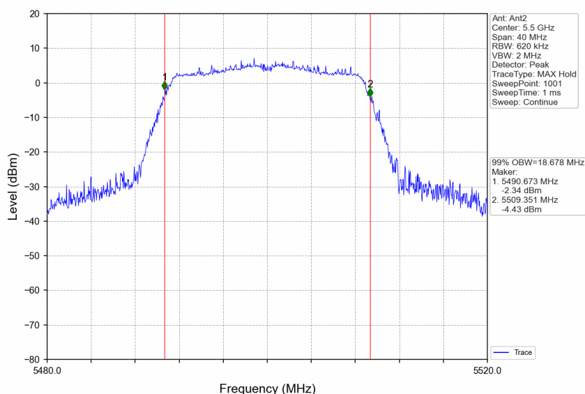
802.11ac(VHT20) LCH_5500MHz_Ant2_NTNV
