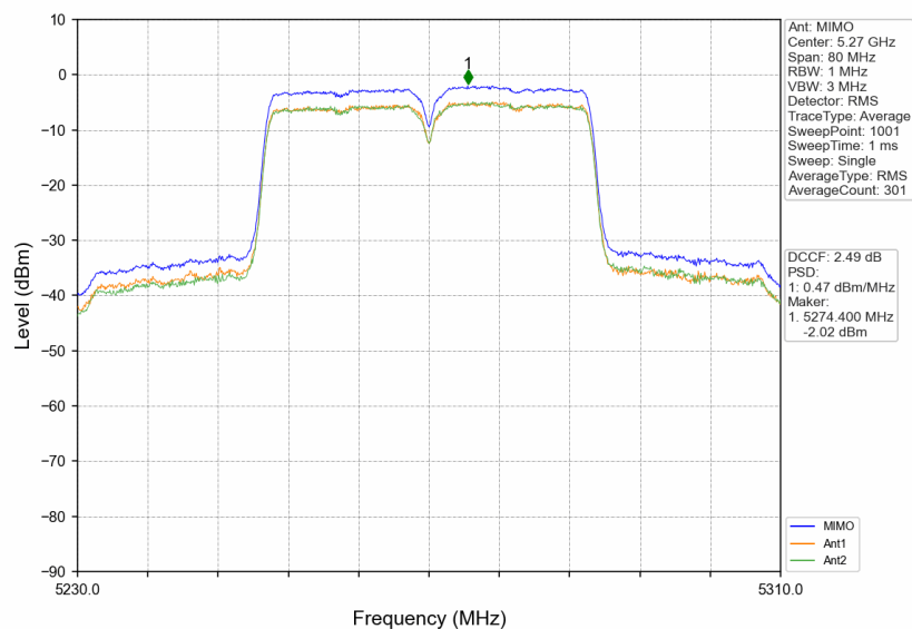
802.11n(HT40) LCH_5270MHz_MIMO_NTNV
