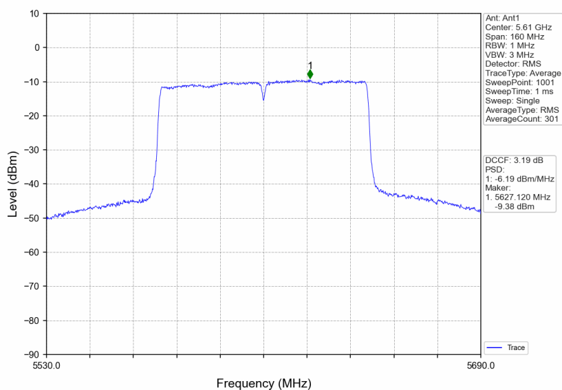
802.11ac(VHT80)_HCH_5610MHz_Ant1_NTNV
