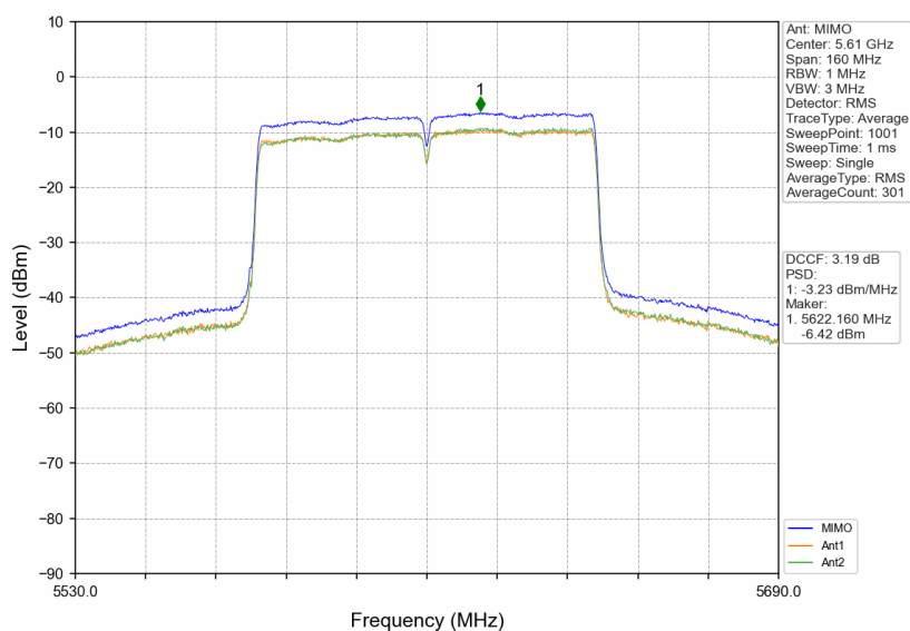
802.11ac(VHT80) HCH_5610MHz_MIMO_NTNV
