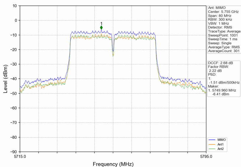
802.11n(HT40) LCH_5755MHz_MIMO_NTNV
