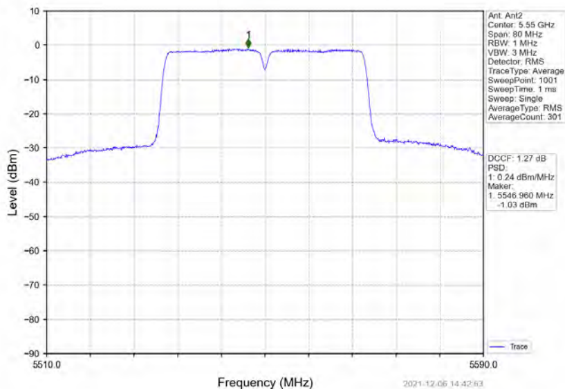
802.11n(HT40)_MCH_5550MHz_MIMO_NTNV
