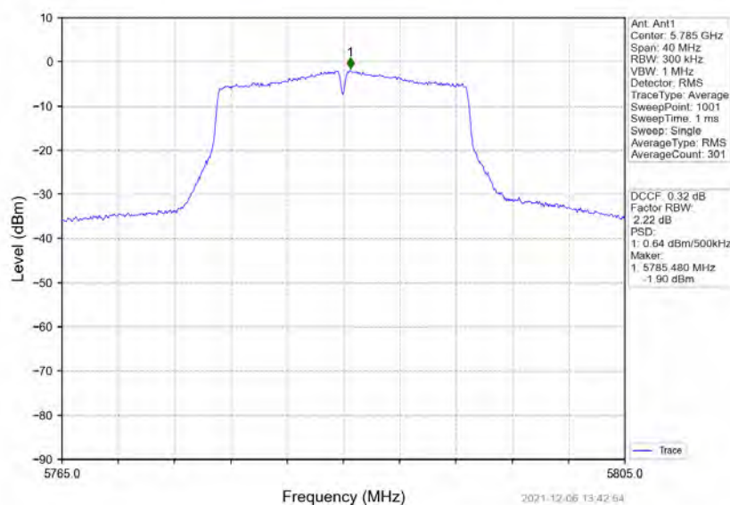
802.11n(HT20)_MCH_5785MHz_Ant1_NTNV
