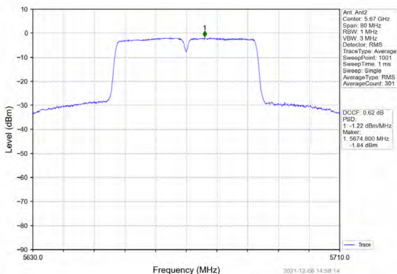
802.11n(HT40) HCH_5670MHz_MIMO_NTNV
