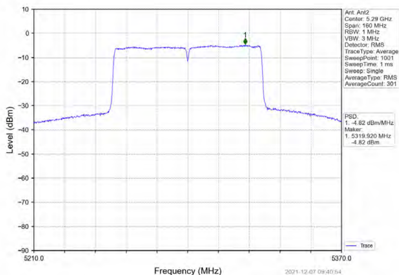
802.11ac(VHT80) MCH 5290MHz MIMO NTN
