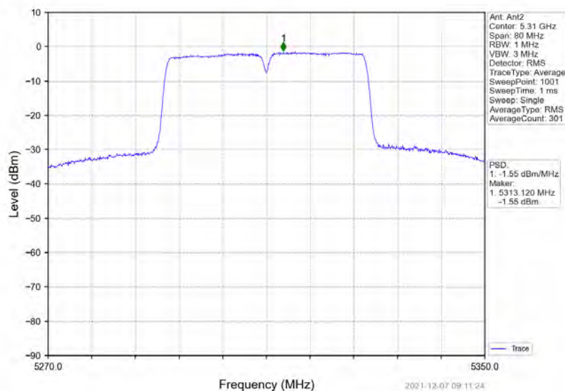
802.11ac(VHT40) HCH 5310MHz MIMO NTN
