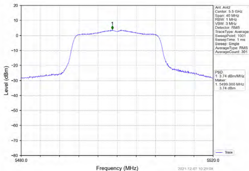
802.11ac(VHT20) LCH 5500MHz MIMO NTN
