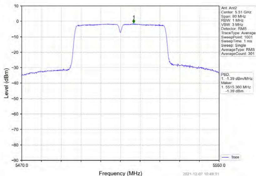
802.11ac(VHT40) LCH 5510MHz MIMO NTNv
