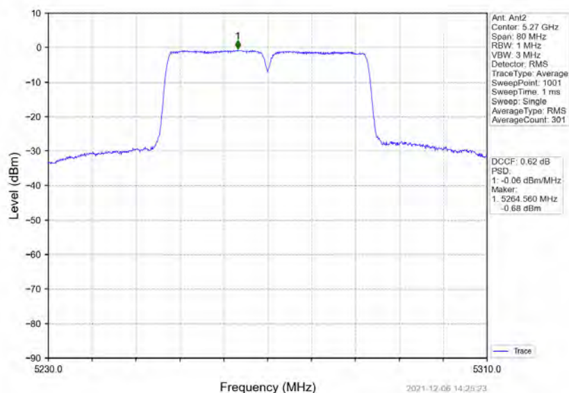
802.11n(HT40) LCH 5270MHz MIMO NTN
