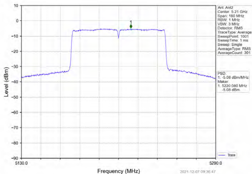
802.11ac(VHT80) MCH 5210MHz MIMO NTN
