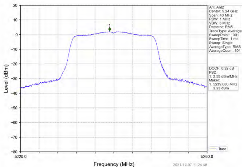
802.11n(HT20) HCH 5240MHz MIMO NTN
