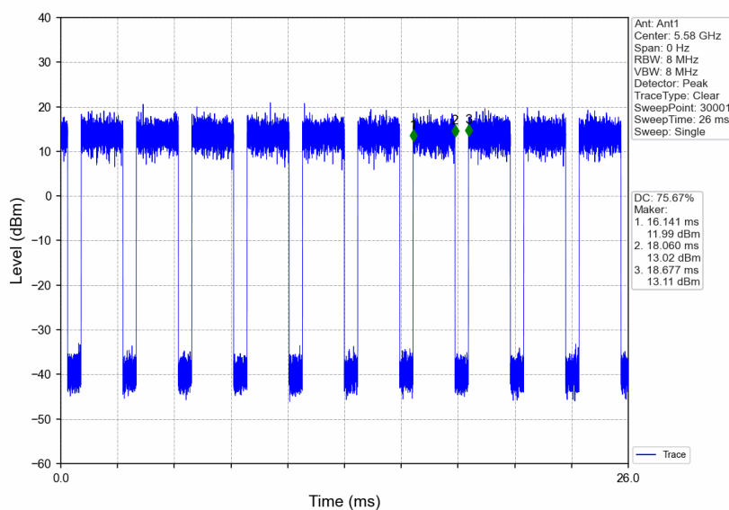
802.11n(HT20) MCH_5580MHz_Ant1_NTNV
