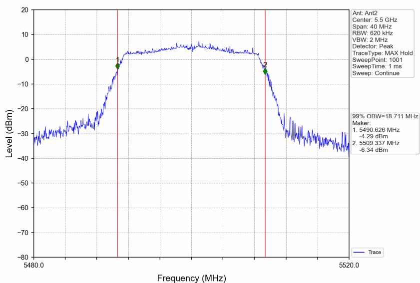
802.11ac(VHT20) LCH_5500MHz_Ant2_NTNV
