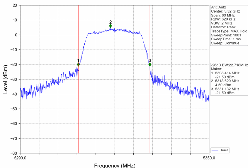
802.11n(HT20)_HCH_5320MHz_Ant2_NTNV
