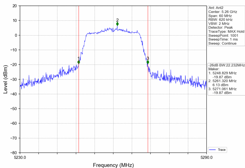
802.11n(HT20) LCH_5260MHz_Ant2_NTNV
