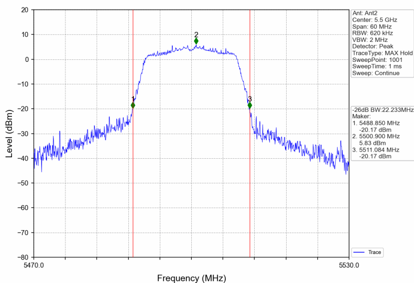
802.11n(HT20) LCH_5500MHz_Ant2_NTNV
