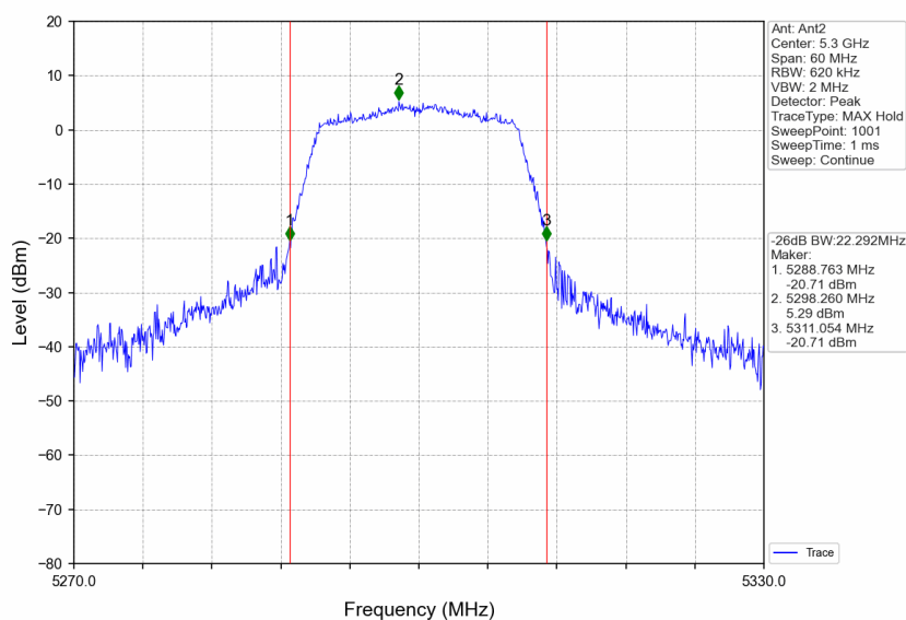
802.11n(HT20)_MCH_5300MHz_Ant2_NTNV
