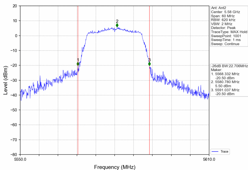
802.11ac(VHT20) MCH 5580MHz_Ant2_NTNV
