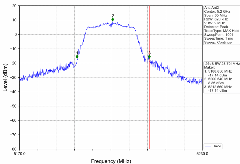
802.11a_MCH_5200MHz_Ant2_NTNV
