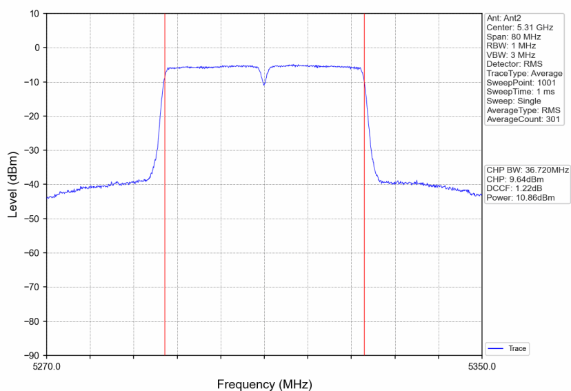
802.11ac(VHT40) HCH 5310MHz Ant2 NTNV
