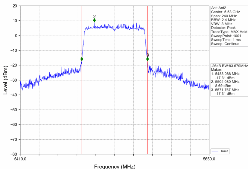
802.11ac(VHT80) LCH_5530MHz_Ant2_NTNV
