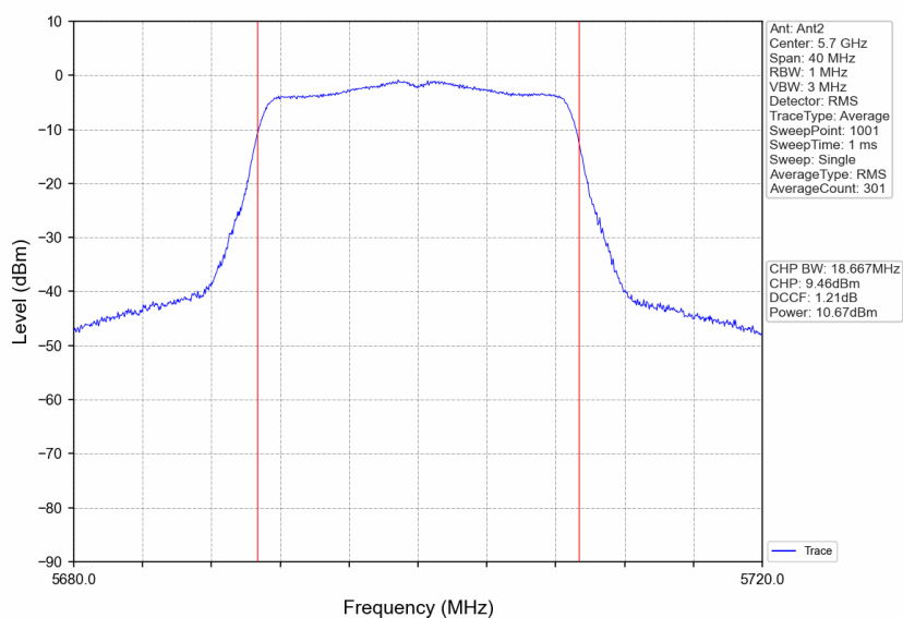
802.11ac(VHT20) HCH 5700MHz Ant2 NTV
