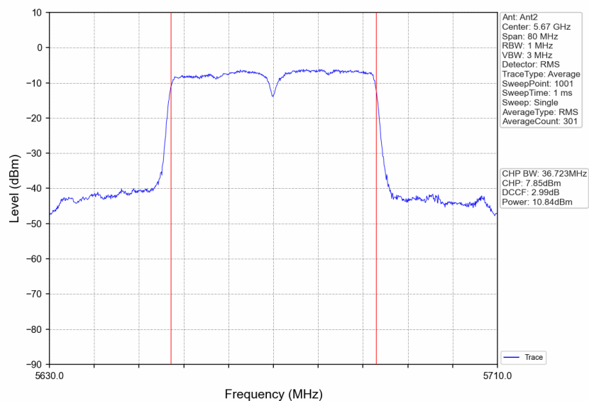
802.11n(HT40) HCH 5670MHz Ant2 NTV
