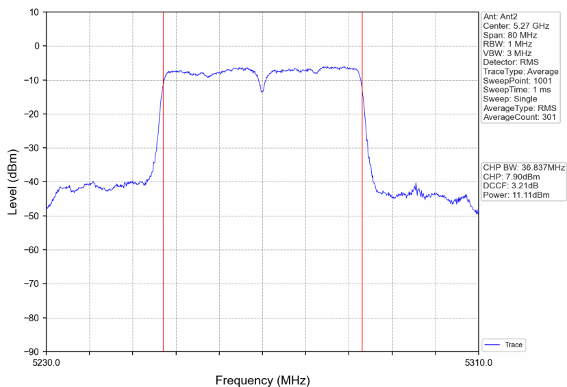
802.11n(HT40) LCH 5270MHz Ant2 NTNV
