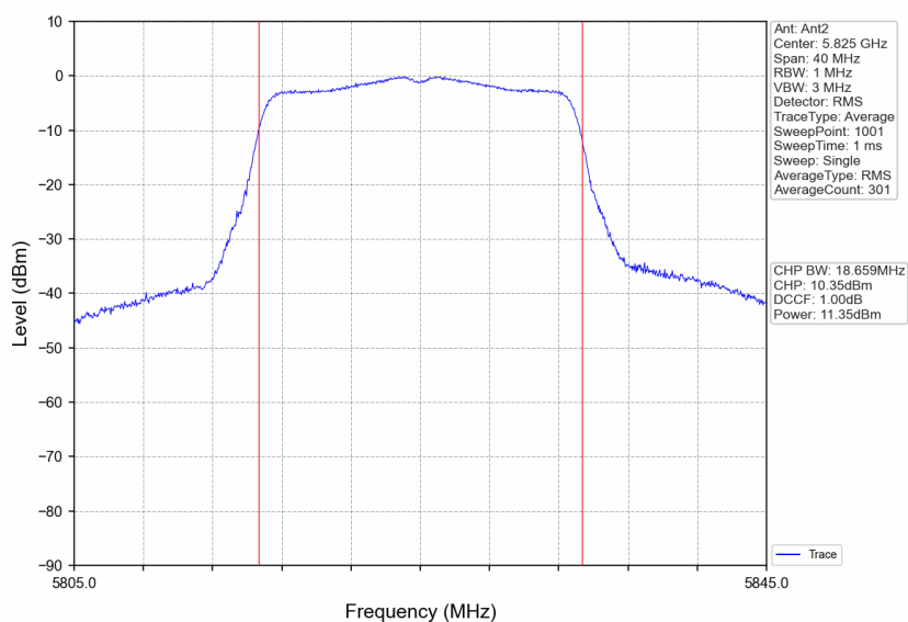
802.11n(HT20)_HCH_5825MHz_Ant2_NTNV
