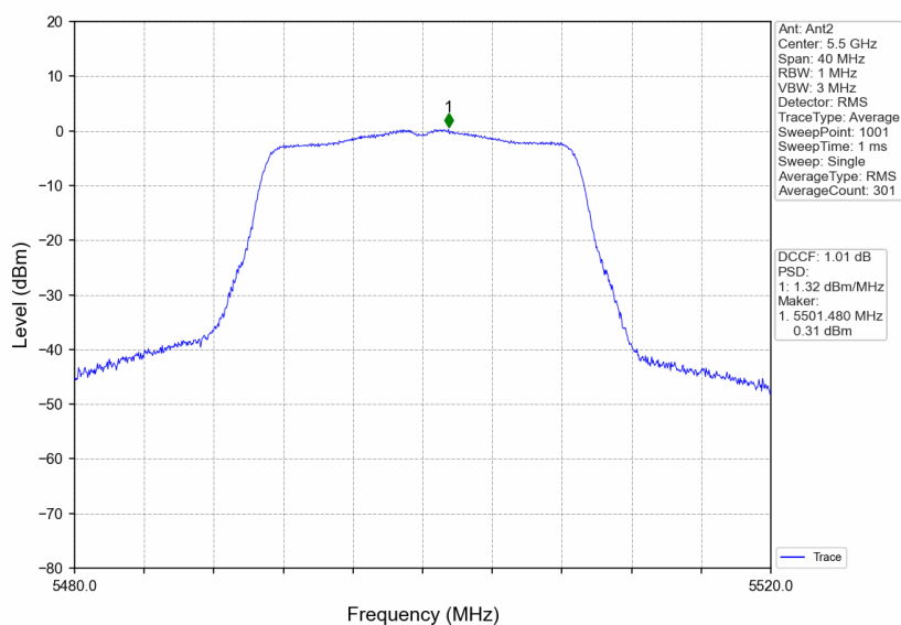
802.11n(HT20) LCH_5500MHz_Ant2_NTNV
