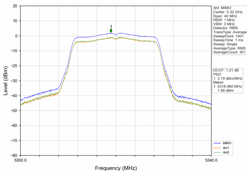
802.11n(HT20)_HCH_5320MHz_MIMO_NTNV
