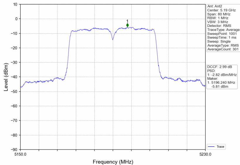
802.11n(HT40) LCH_5190MHz_MIMO_NTNV
