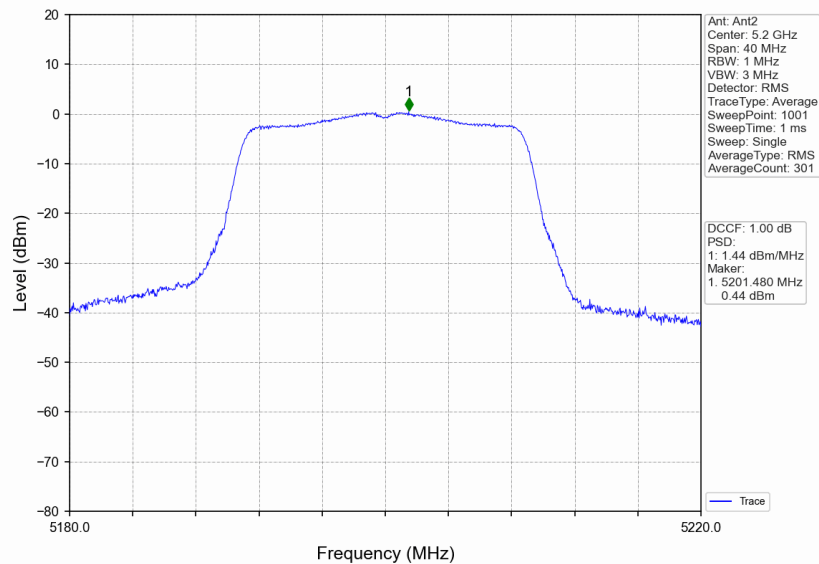
802.11n(HT20)_MCH_5200MHz_MIMO_NTNV
