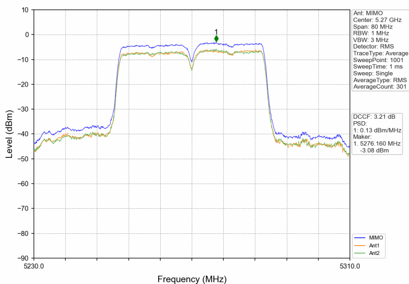
802.11n(HT40) LCH_5270MHz_MIMO_NTNV
