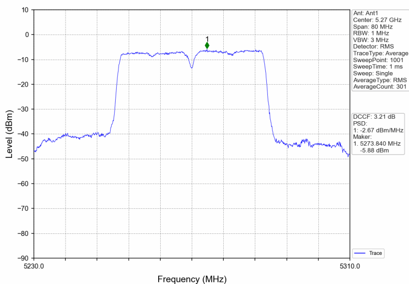
802.11n(HT40)_LCH_5270MHz_Ant1_NTNV
