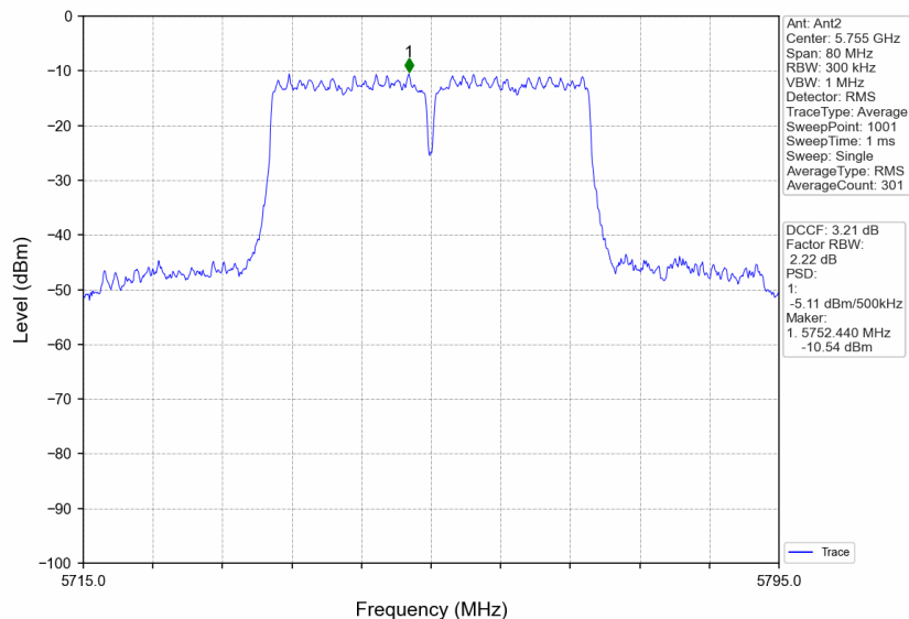
802.11n(HT40) LCH_5755MHz_MIMO_NTNV
