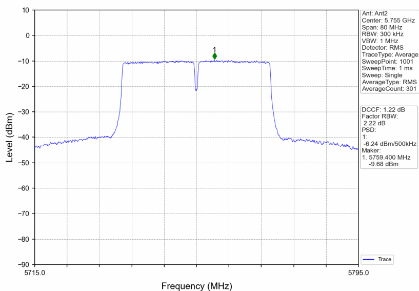
802.11ac(VHT40) LCH_5755MHz_Ant2_NTNV
