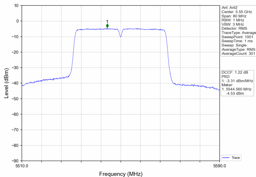
802.11ac(VHT40) MCH 5550MHz_Ant2_NTNV
