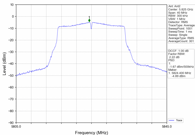
802.11n(HT20)_HCH_5825MHz_Ant2_NTNV
