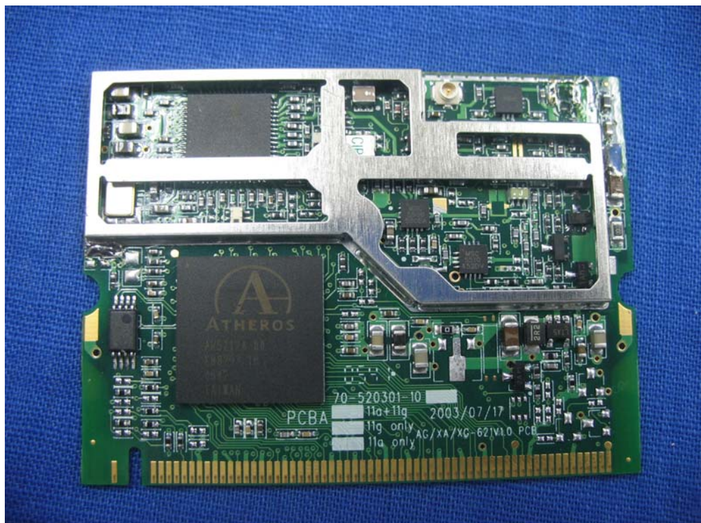
(10) EUT Photo (ZA-5000- I)
