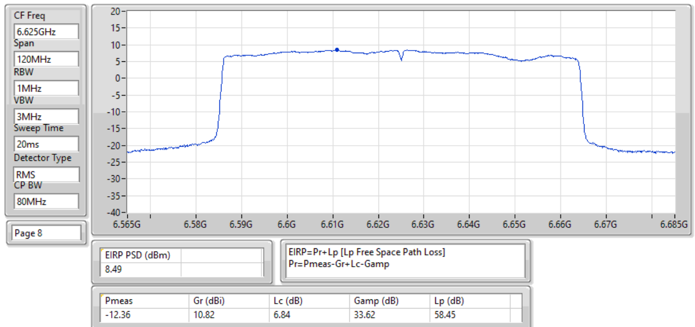
EIRP PSD;Band:6.7G;ax80;BWch:80MHz;Nss:1,(M0);Nant:1(1);Ch:6625MHz;TX
