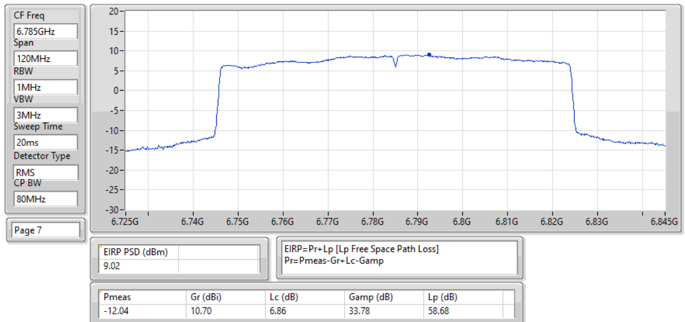
EIRP PSD;Band:6.7G;ax80;BWch:80MHz;Nss:1,(M0);Nant:1(2);Ch:6785MHz;TX
