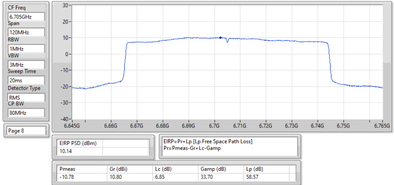
EIRP PSD;Band:6.7G;ax80;BWch:80MHz;Nss:1,(M0);Nant:1(1);Ch:6705MHz;TX
