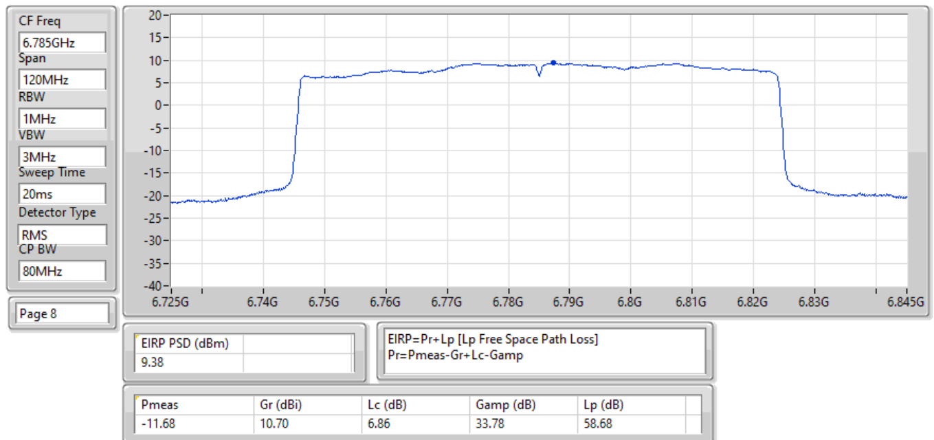
EIRP PSD;Band:6.7G;ax80;BWch:80MHz;Nss:1,(M0);Nant:1(1);Ch:6785MHz;TX
