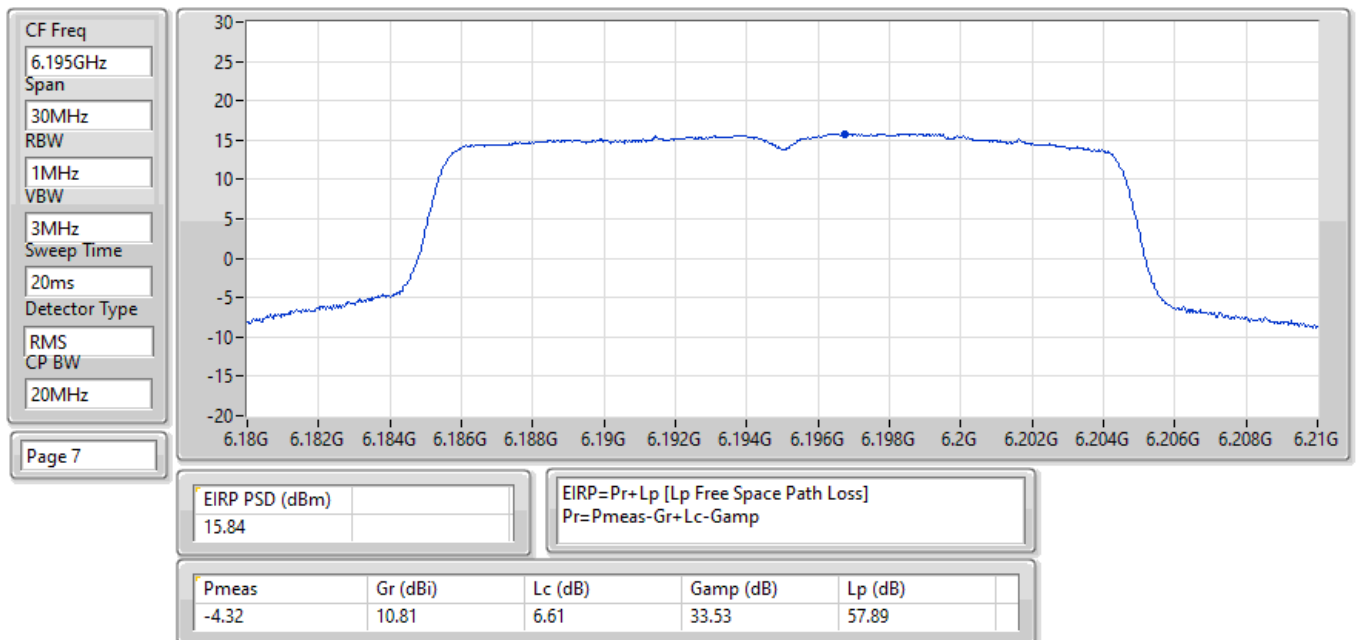
EIRP PSD;Band:6.2G;ax20;BWch:20MHz;Nss:1,(M0);Nant:1(1);Ch:6195MHz;TX
