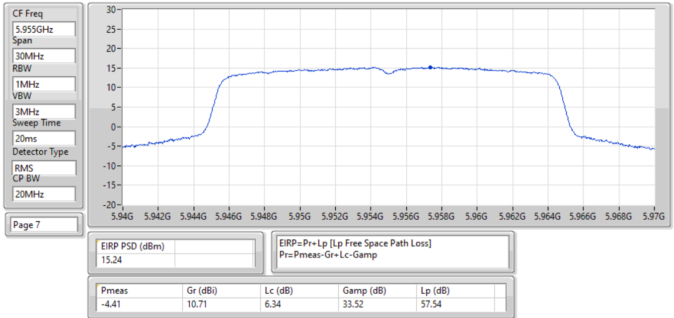
EIRP PSD;Band:6.2G;ax20;BWch:20MHz;Nss:1,(M0);Nant:1(1);Ch:5955MHz;TX
