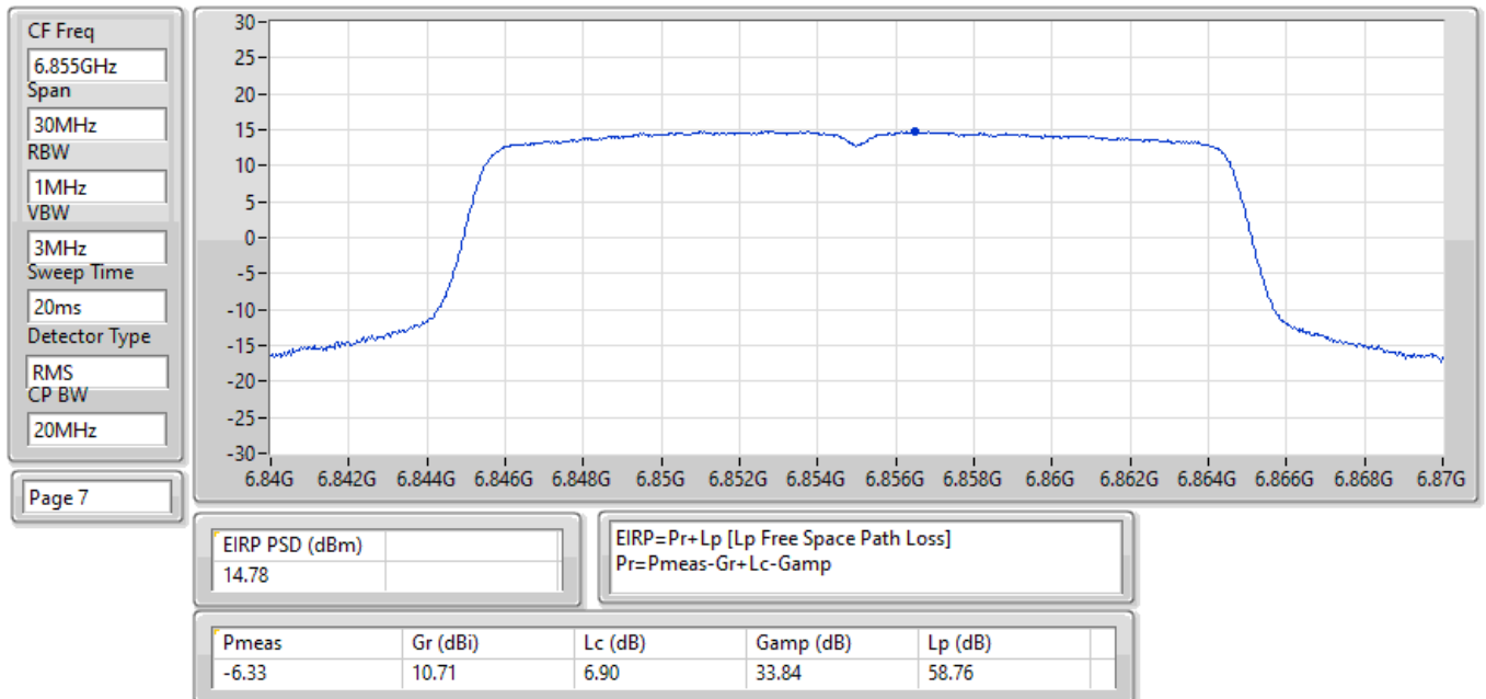
EIRP PSD;Band:6.7G;ax20;BWch:20MHz;Nss:1,(M0);Nant:1(1);Ch:6855MHz;TX
