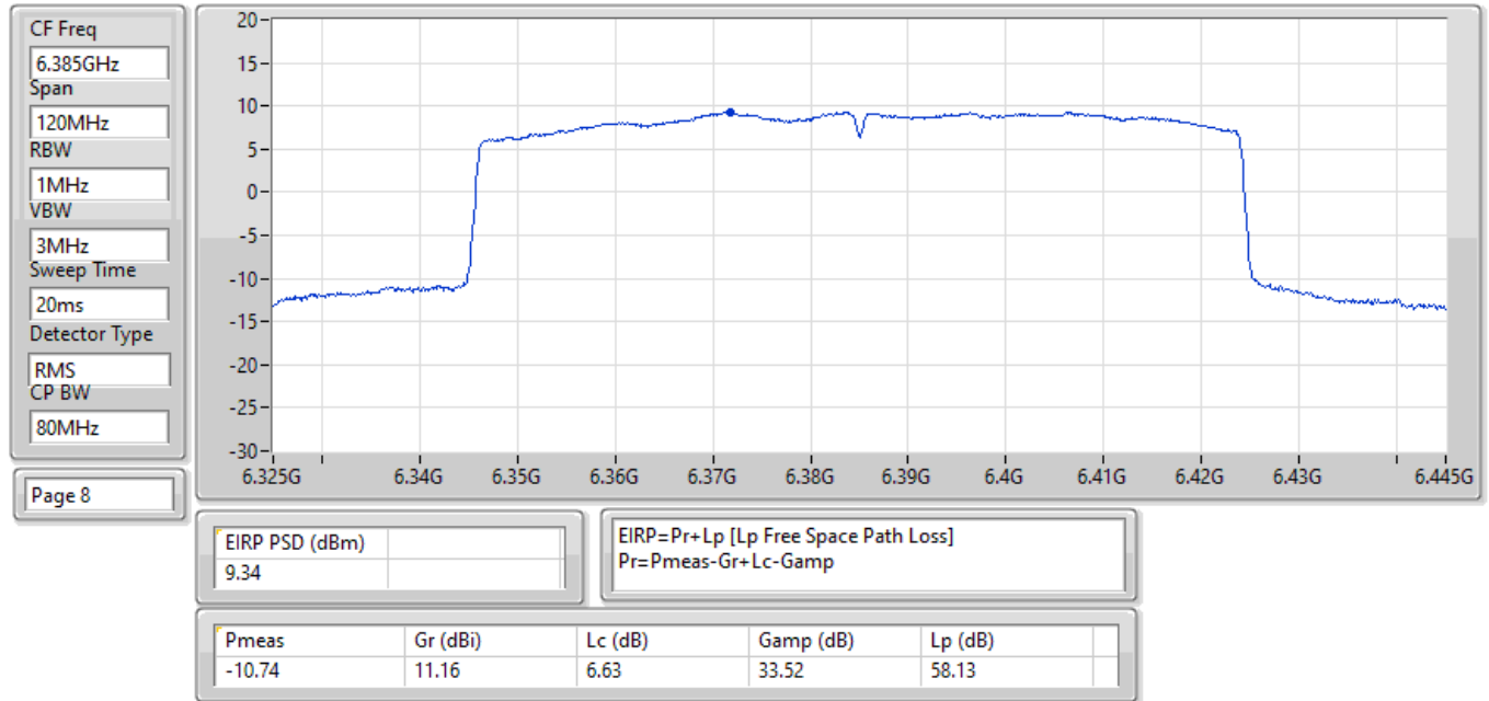
EIRP PSD;Band:6.2G;ax80;BWch:80MHz;Nss:1,(M0);Nant:1(1);Ch:6385MHz;TX
