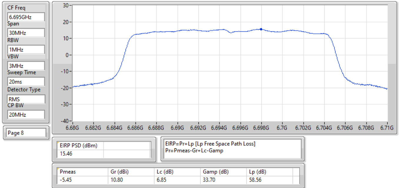
EIRP PSD;Band:6.7G;ax20;BWch:20MHz;Nss:1,(M0);Nant:1(1);Ch:6695MHz;TX
