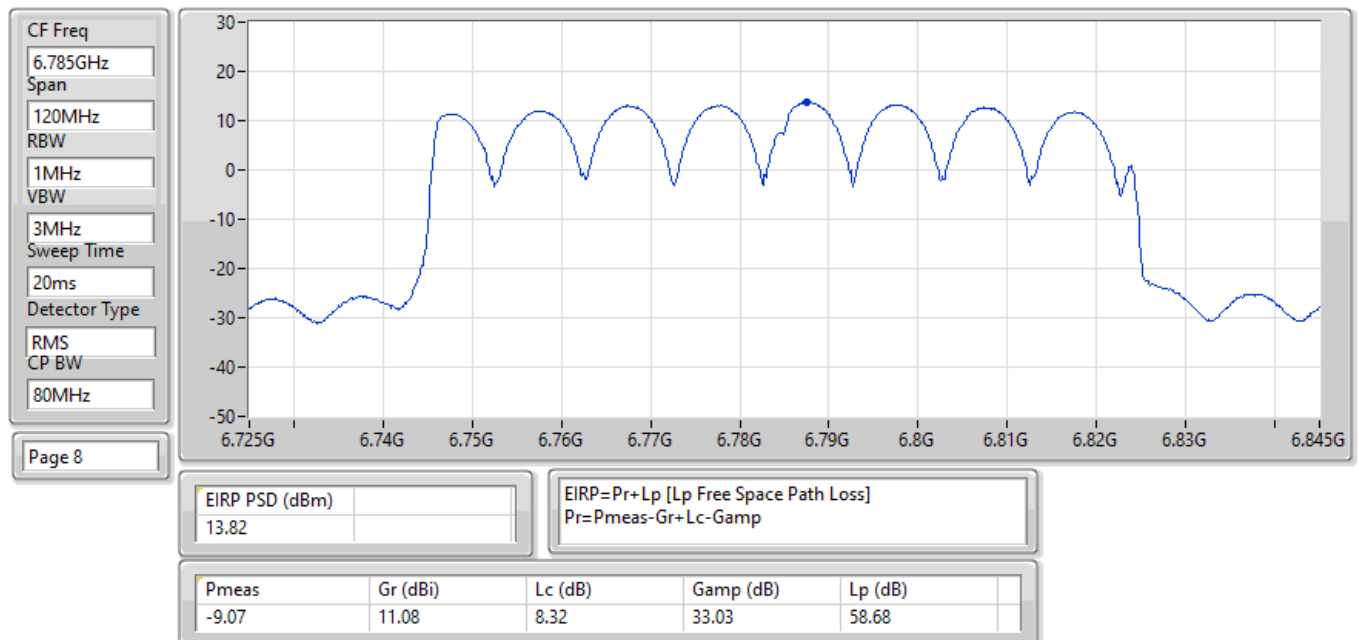
EIRP PSD;Band:6.7G;ax80;BWch:80MHz;Nss:1,(M0);Nant:2;Ch:6785MHz;TX
