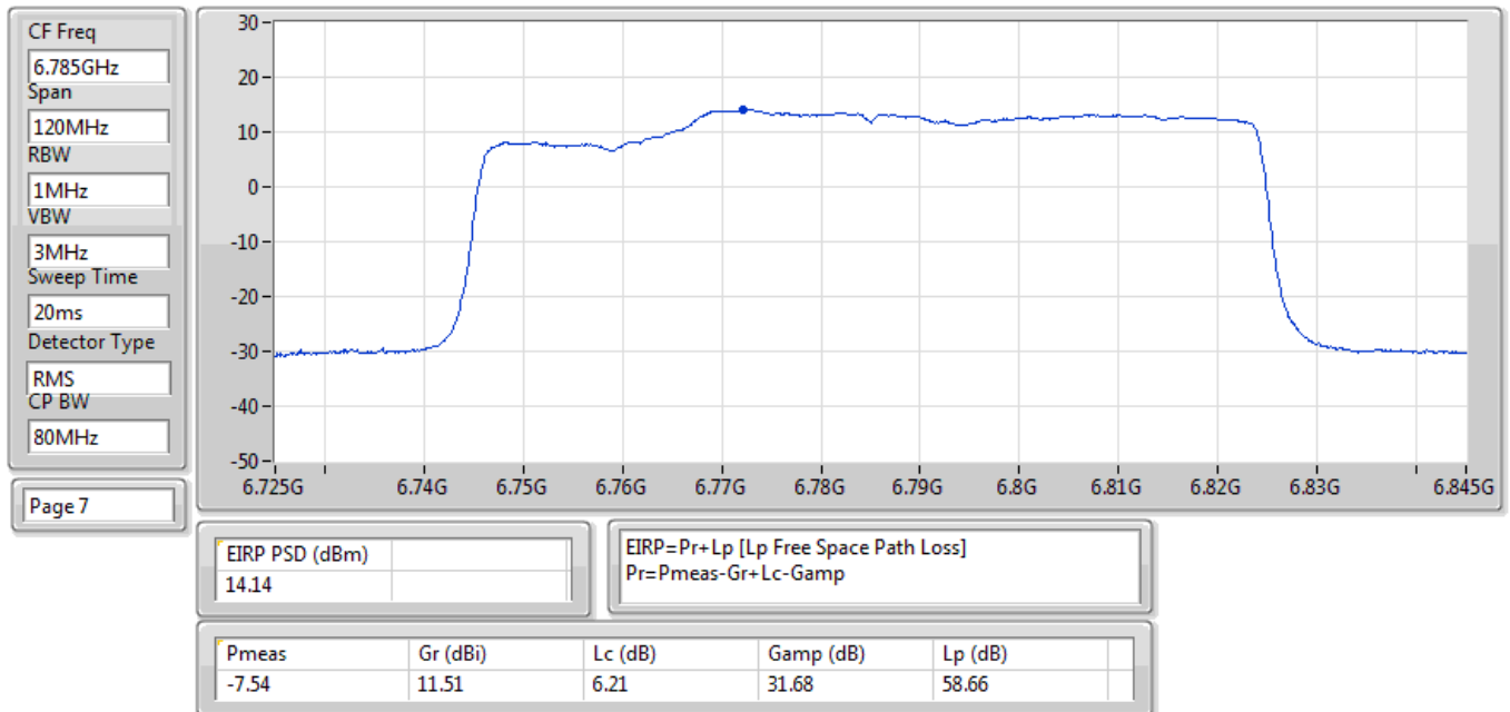
EIRP PSD;Band:6.7G;ax80,BF;BWch:80MHz;Nss:1,(M0);Nant:2;Ch:6785MHz;TX
