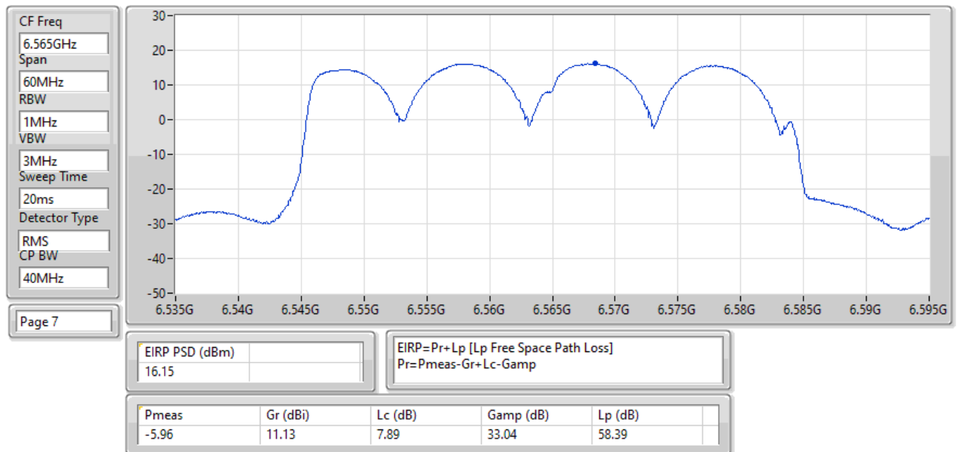
EIRP PSD;Band:6.7G;ax40;BWch:40MHz;Nss:1,(M0);Nant:2;Ch:6565MHz;TX
