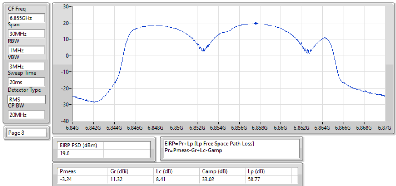
EIRP PSD;Band:6.7G;ax20;BWch:20MHz;Nss:1,(M0);Nant:2;Ch:6855MHz;TX
