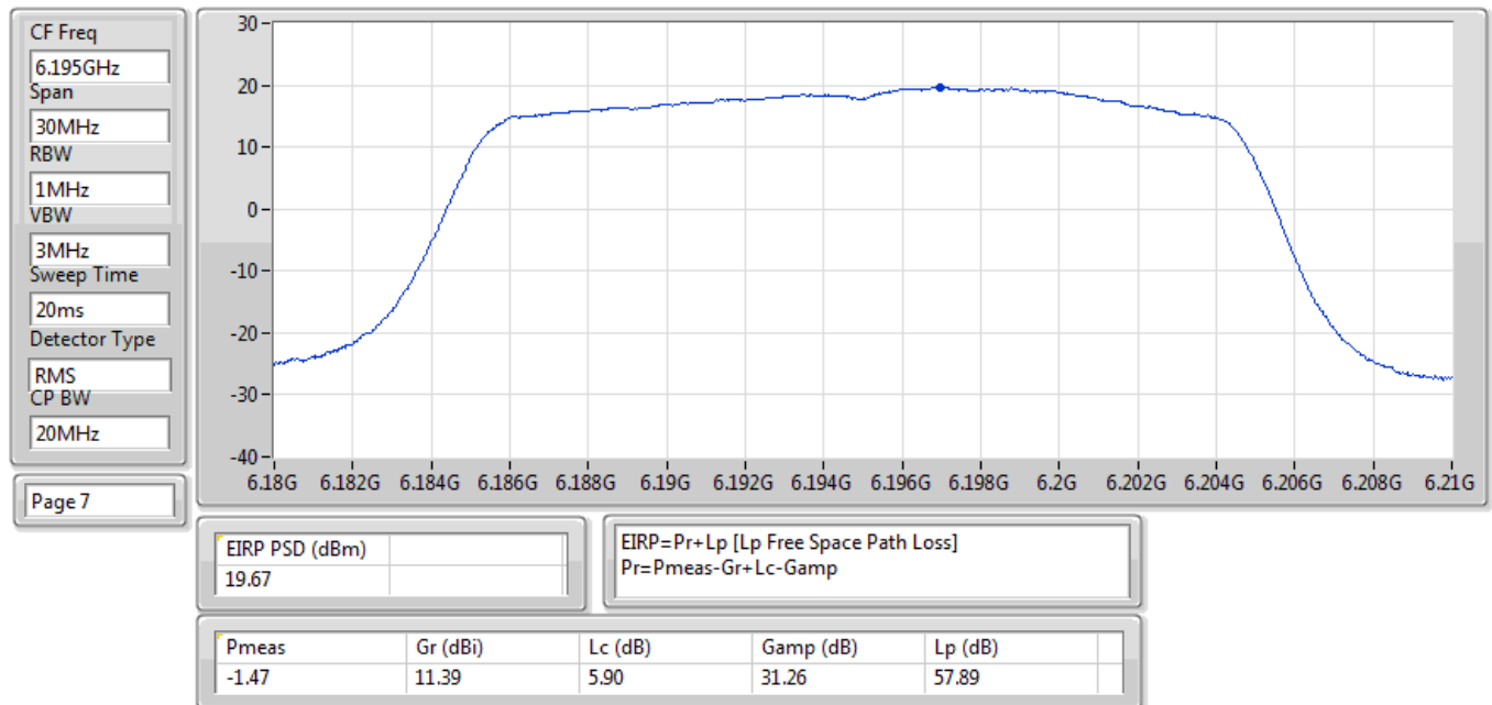
EIRP PSD;Band:6.2G;ax20,BF;BWch:20MHz;Nss:1,(M0);Nant:2;Ch:6195MHz;TX
