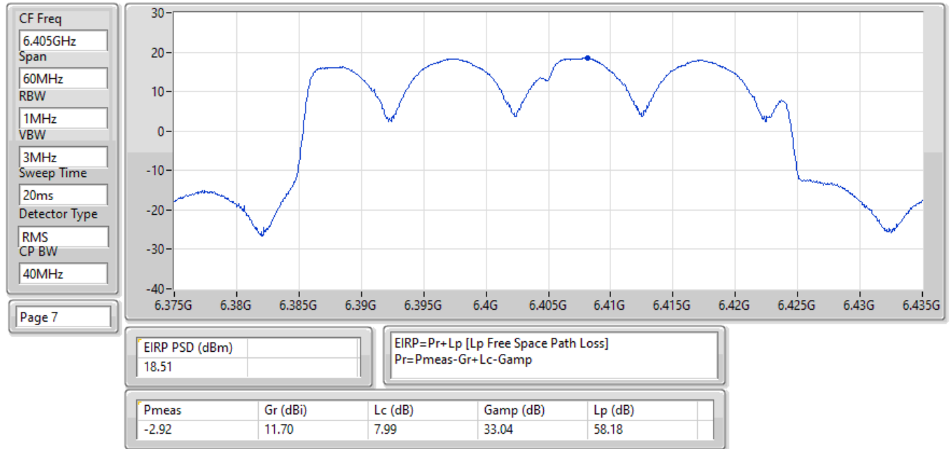
EIRP PSD;Band:6.2G;ax40;BWch:40MHz;Nss:1,(M0);Nant:2;Ch:6405MHz;TX
