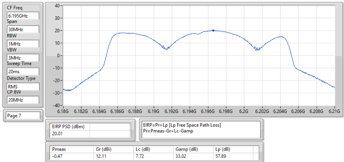
EIRP PSD;Band:6.2G;ax20;BWch:20MHz;Nss:1,(M0);Nant:2;Ch:6195MHz;TX
