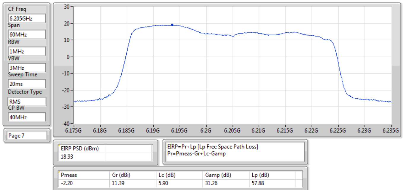
EIRP PSD;Band:6.2G;ax40,BF;BWch:40MHz;Nss:1,(M0);Nant:2;Ch:6205MHz;TX
