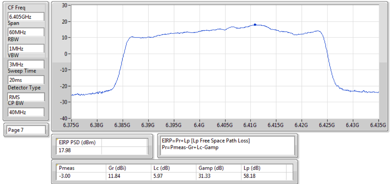
EIRP PSD;Band:6.2G;ax40,BF;BWch:40MHz;Nss:1,(M0);Nant:2;Ch:6405MHz;TX
