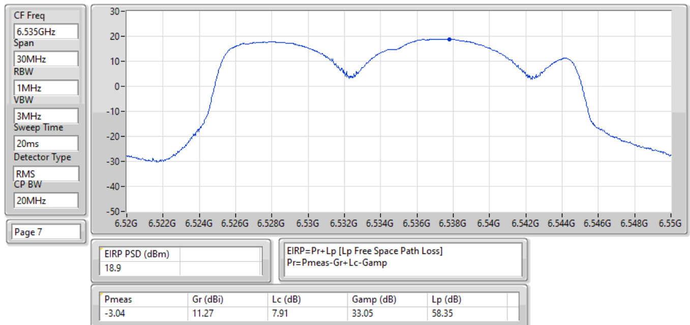
EIRP PSD;Band:6.7G;ax20;BWch:20MHz;Nss:1,(M0);Nant:2;Ch:6535MHz;TX
