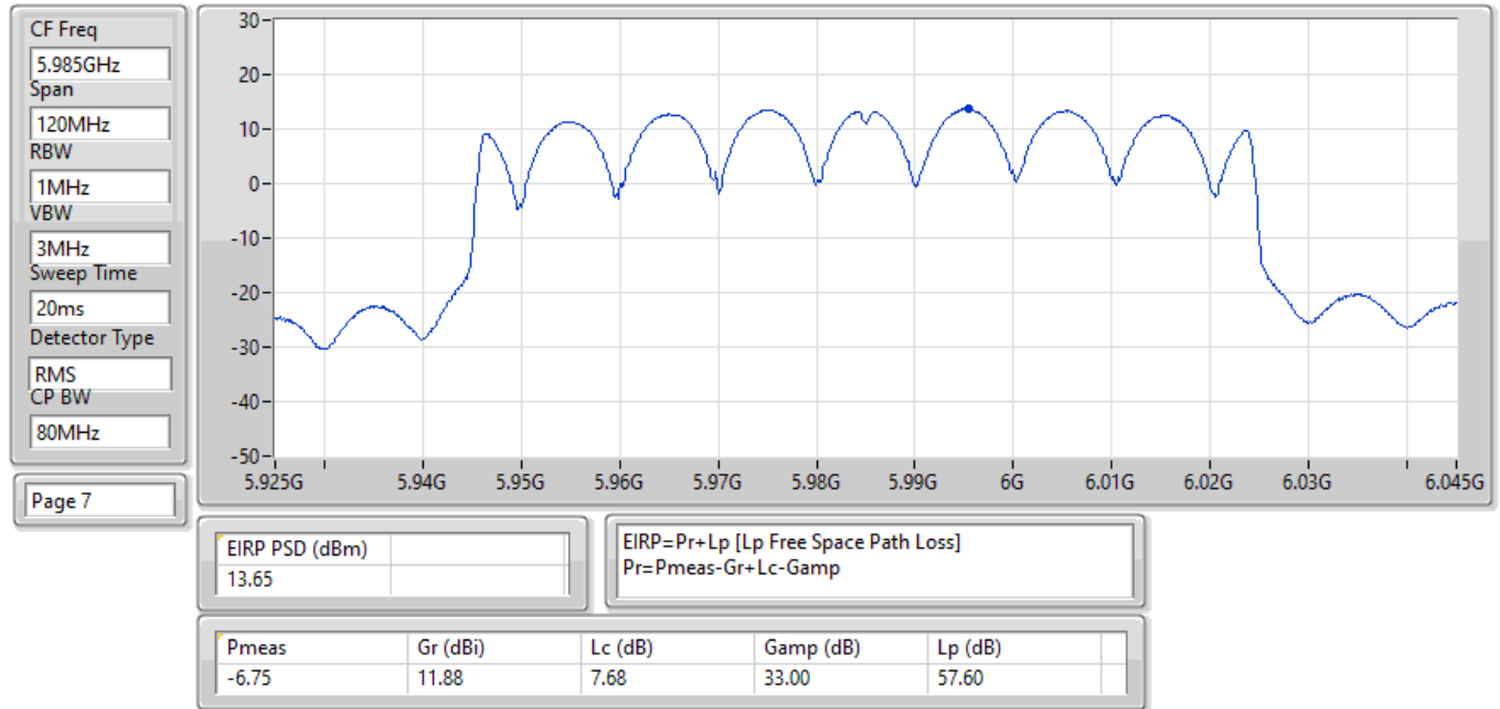
EIRP PSD;Band:6.2G;ax80;BWch:80MHz;Nss:1,(M0);Nant:2;Ch:5985MHz;TX
