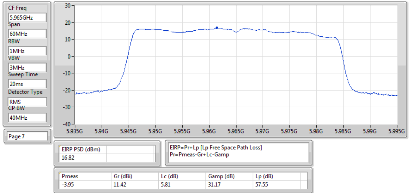
EIRP PSD;Band:6.2G;ax40,BF;BWch:40MHz;Nss:1,(M0);Nant:2;Ch:5965MHz;TX
