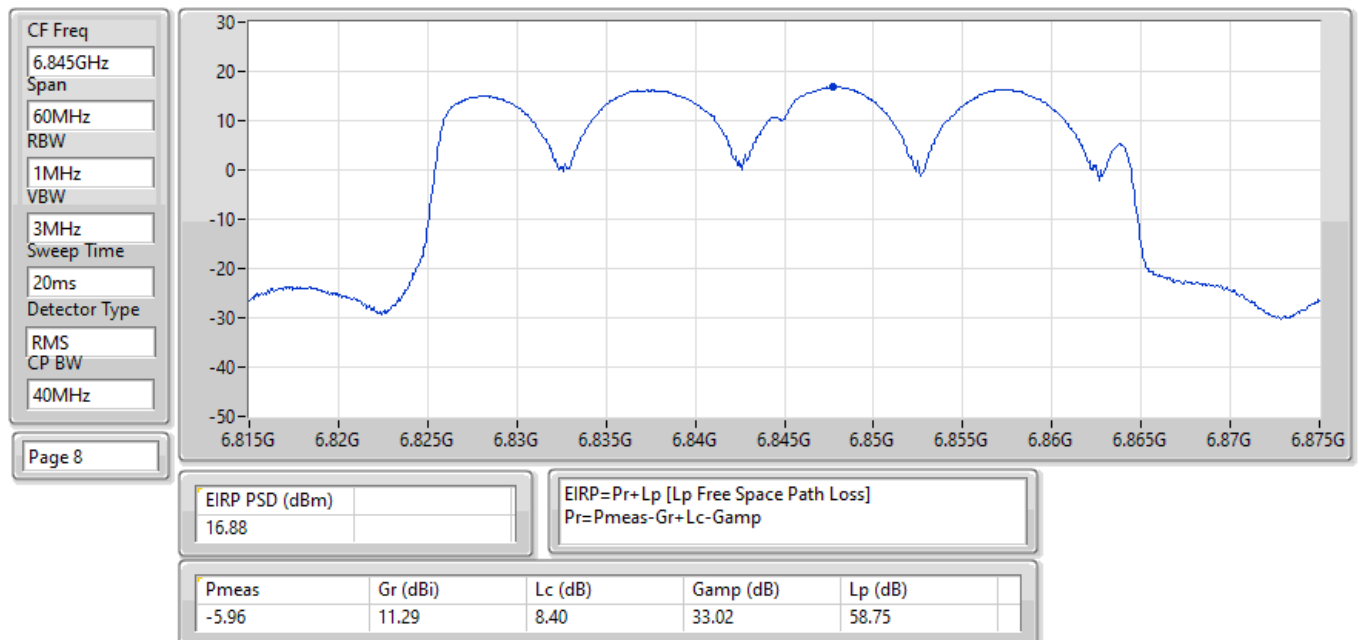
EIRP PSD;Band:6.7G;ax40;BWch:40MHz;Nss:1,(M0);Nant:2;Ch:6845MHz;TX
