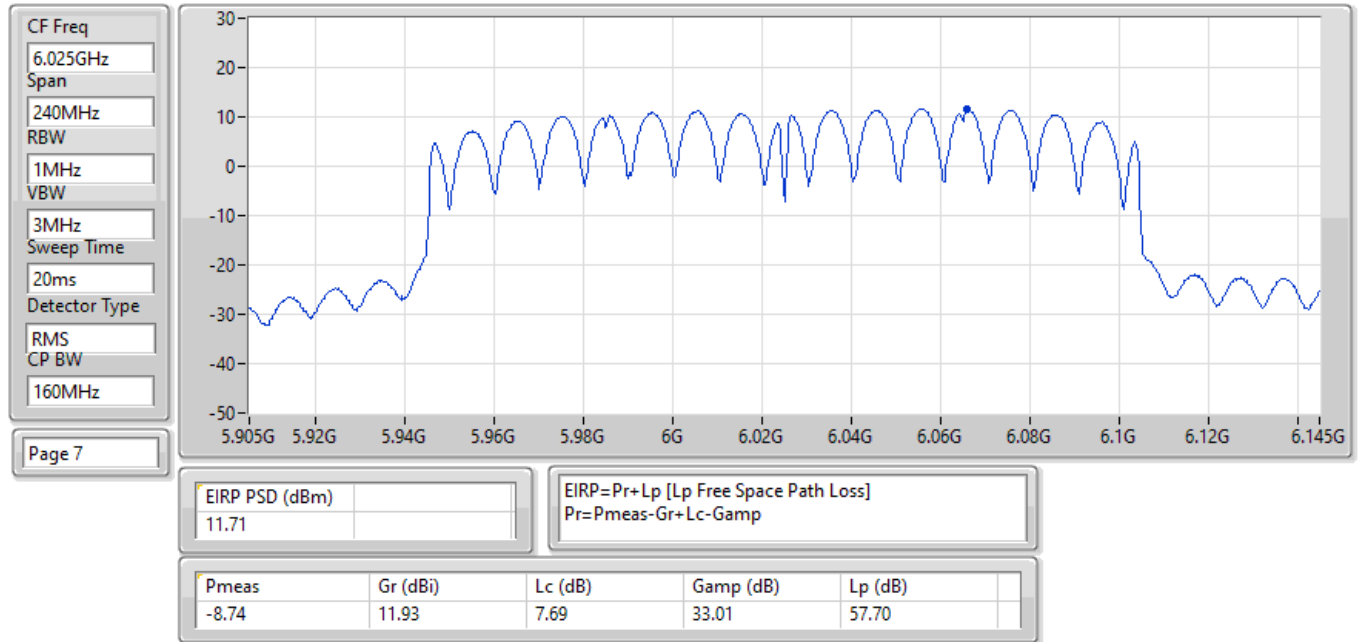
EIRP PSD;Band:6.2G;ax160;BWch:160MHz;Nss:1,(M0);Nant:2;Ch:6025MHz;TX
