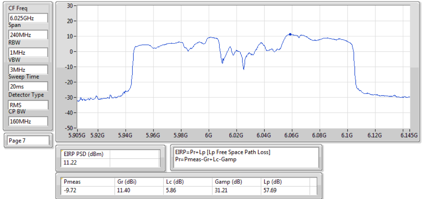
EIRP PSD;Band:6.2G;ax160,BF;BWch:160MHz;Nss:1,(M0);Nant:2;Ch:6025MHz;TX
