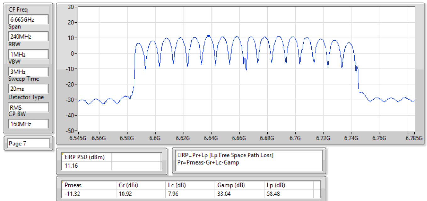
EIRP PSD;Band:6.7G;ax160;BWch:160MHz;Nss:1,(M0);Nant:2;Ch:6665MHz;TX
