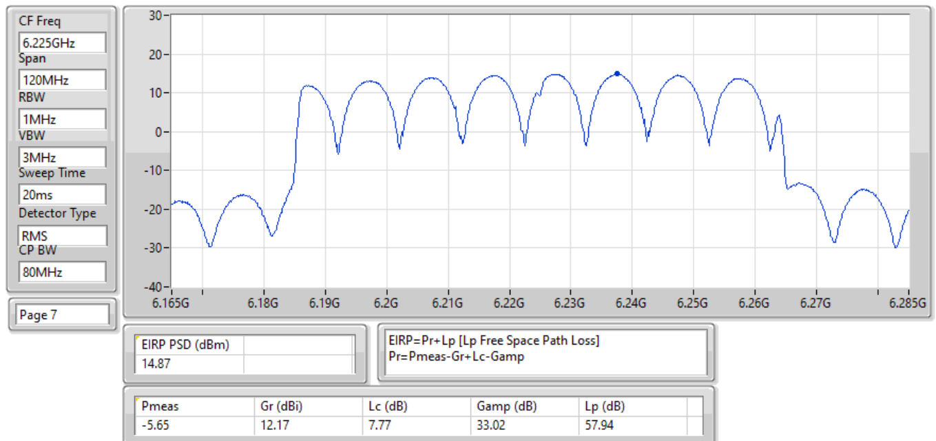
EIRP PSD;Band:6.2G;ax80;BWch:80MHz;Nss:1,(M0);Nant:2;Ch:6225MHz;TX
