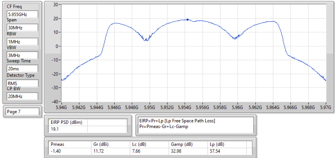
EIRP PSD;Band:6.2G;ax20;BWch:20MHz;Nss:1,(M0);Nant:2;Ch:5955MHz;TX
