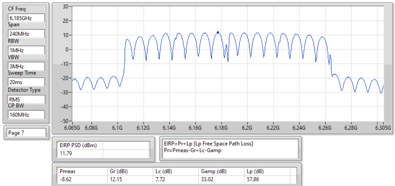
EIRP PSD;Band:6.2G;ax160;BWch:160MHz;Nss:1,(M0);Nant:2;Ch:6185MHz;TX
