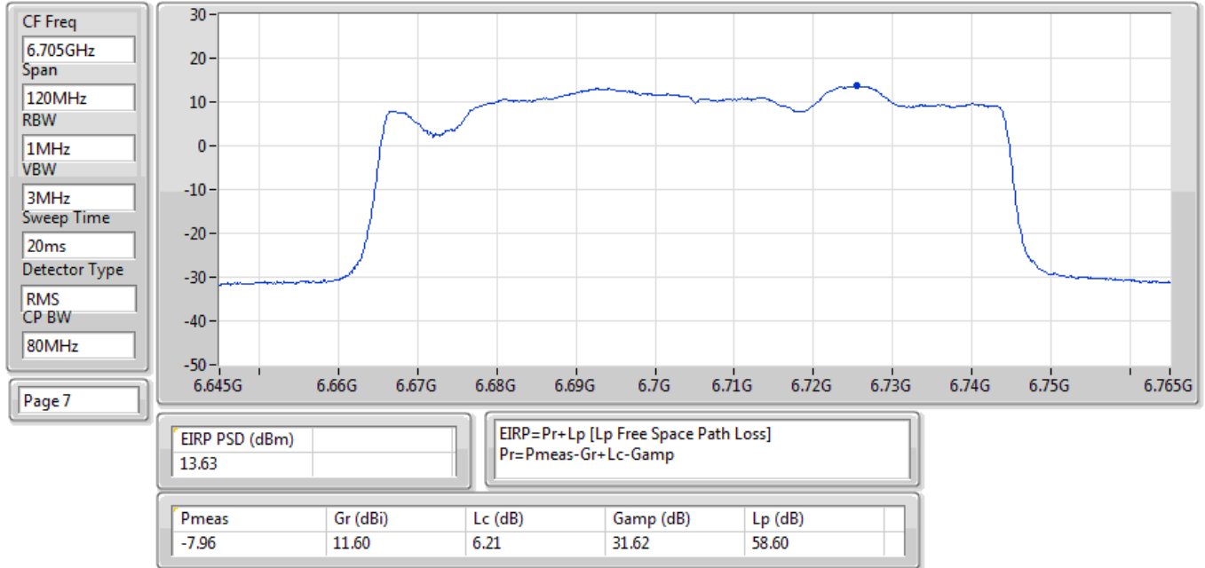
EIRP PSD;Band:6.7G;ax80,BF;BWch:80MHz;Nss:1,(M0);Nant:2;Ch:6705MHz;TX
