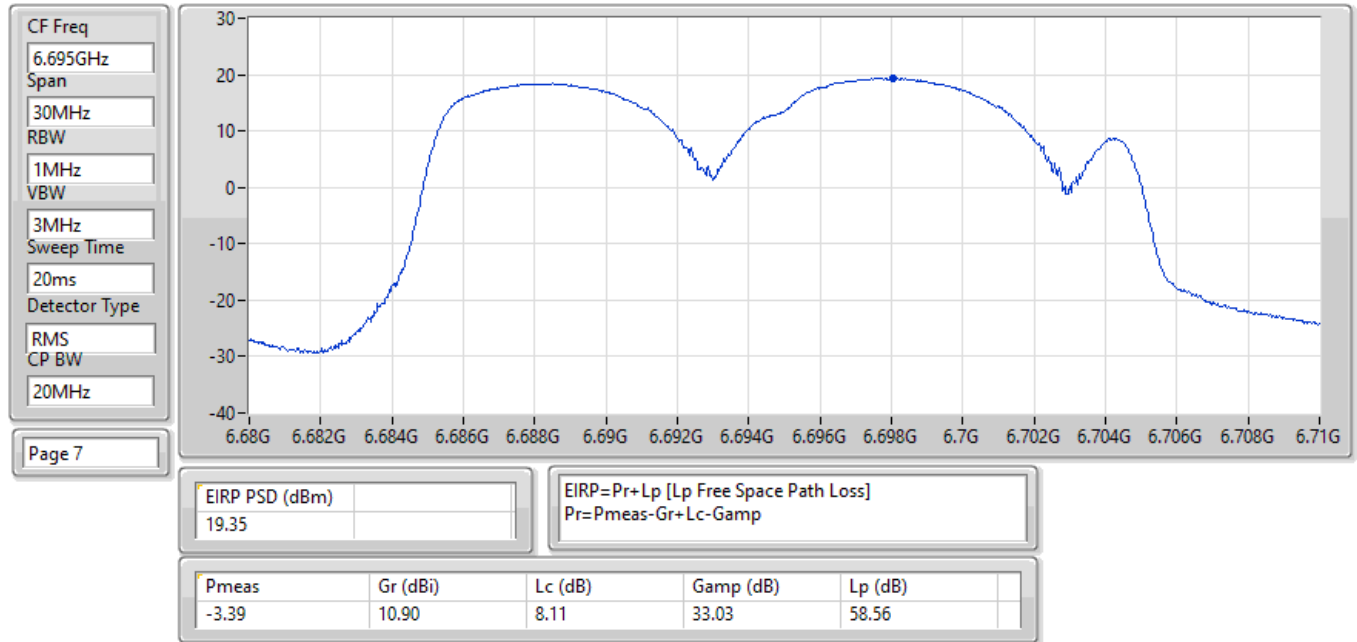
EIRP PSD;Band:6.7G;ax20;BWch:20MHz;Nss:1,(M0);Nant:2;Ch:6695MHz;TX
