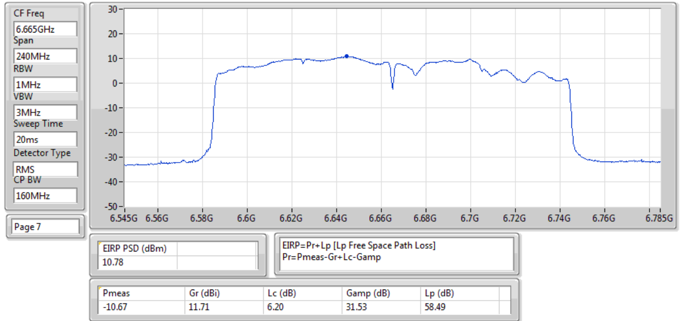
EIRP PSD;Band:6.7G;ax160,BF;BWch:160MHz;Nss:1,(M0);Nant:2;Ch:6665MHz;TX
