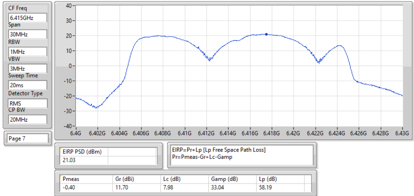
EIRP PSD;Band:6.2G;ax20;BWch:20MHz;Nss:1,(M0);Nant:2;Ch:6415MHz;TX
