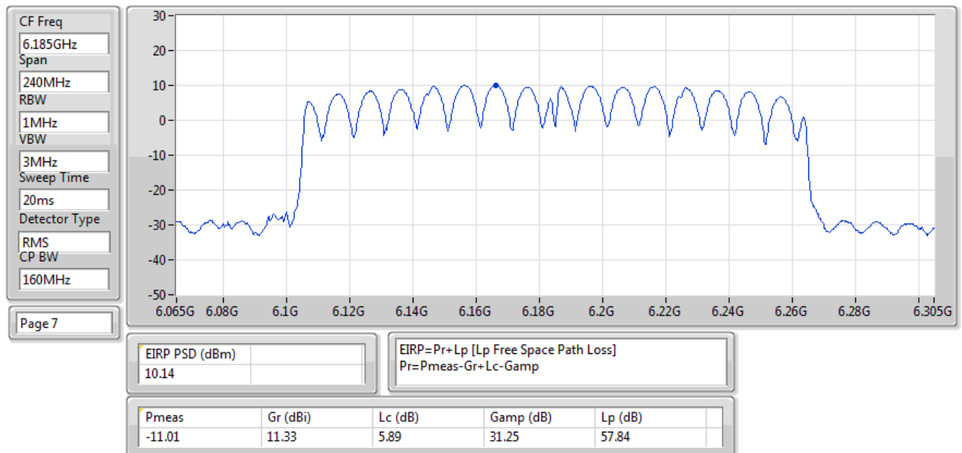
EIRP PSD;Band:6.2G;ax160,BF;BWch:160MHz;Nss:1,(M0);Nant:2;Ch:6185MHz;TX
