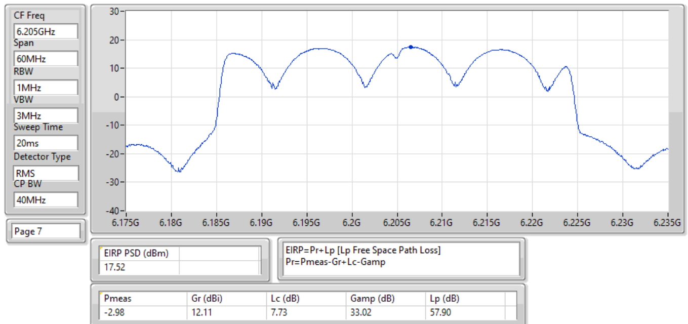
EIRP PSD;Band:6.2G;ax40;BWch:40MHz;Nss:1,(M0);Nant:2;Ch:6205MHz;TX
