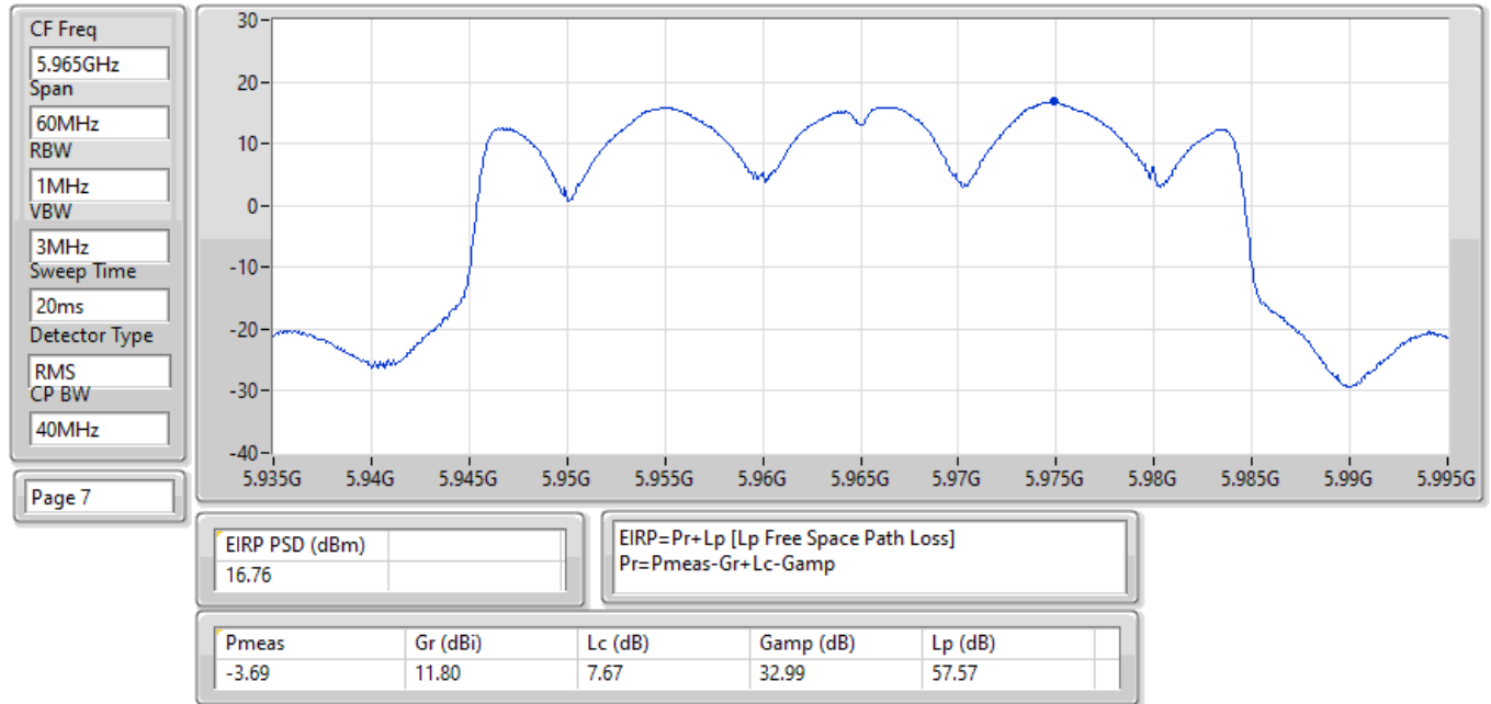
EIRP PSD;Band:6.2G;ax40;BWch:40MHz;Nss:1,(M0);Nant:2;Ch:5965MHz;TX
