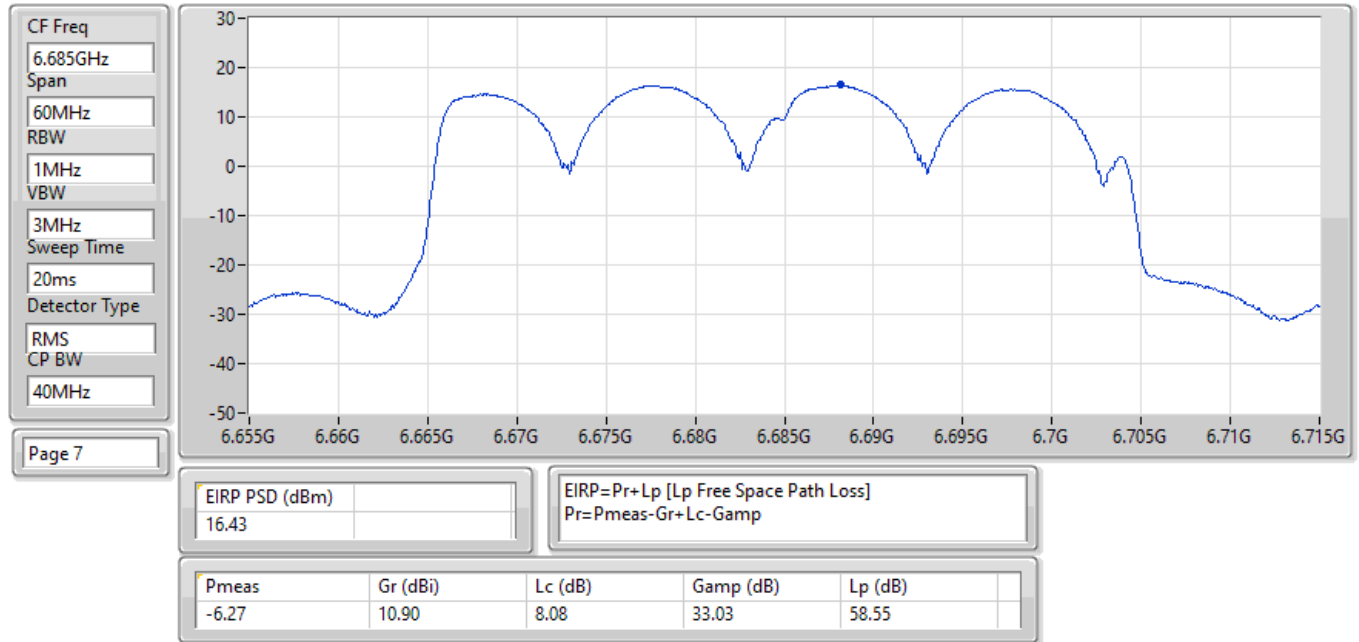
EIRP PSD;Band:6.7G;ax40;BWch:40MHz;Nss:1,(M0);Nant:2;Ch:6685MHz;TX
