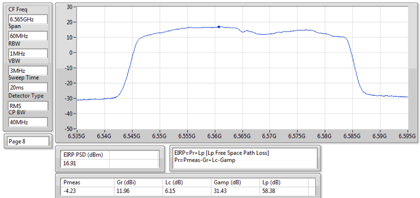
EIRP PSD;Band:6.7G;ax40,BF;BWch:40MHz;Nss:1,(M0);Nant:2;Ch:6565MHz;TX
