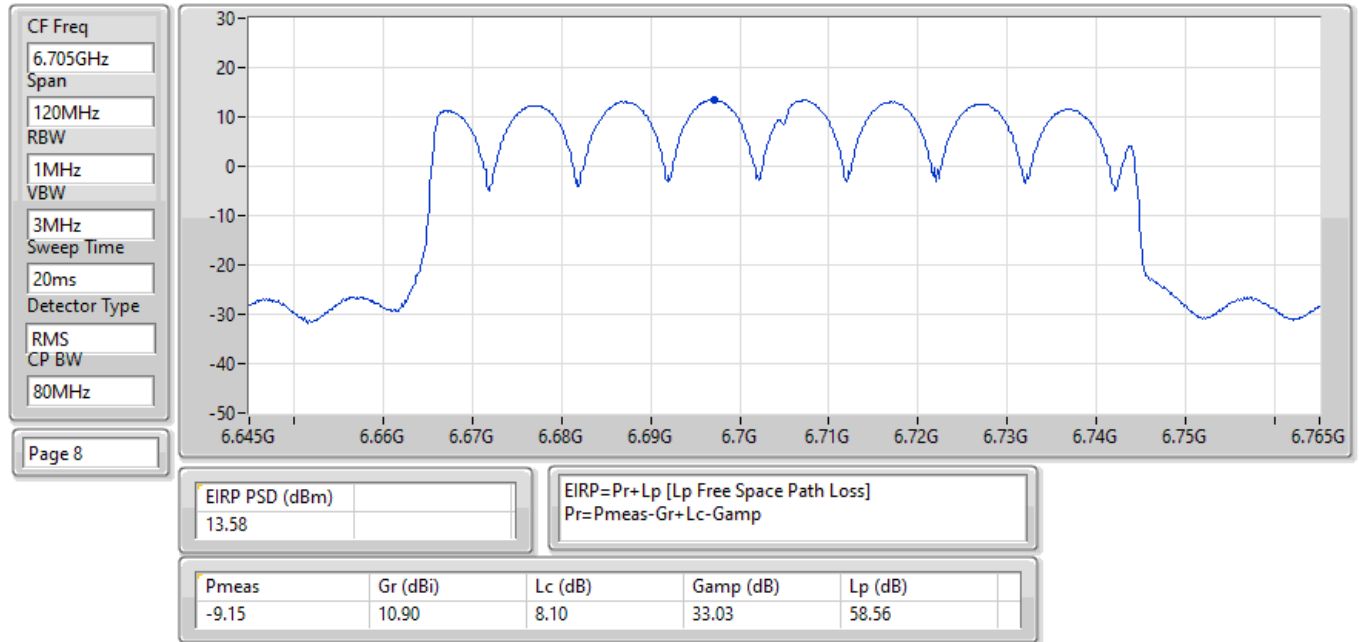
EIRP PSD;Band:6.7G;ax80;BWch:80MHz;Nss:1,(M0);Nant:2;Ch:6705MHz;TX
