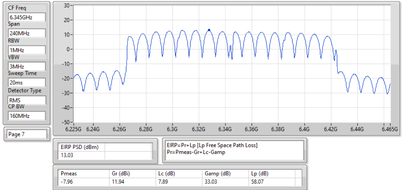
EIRP PSD;Band:6.2G;ax160;BWch:160MHz;Nss:1,(M0);Nant:2;Ch:6345MHz;TX
