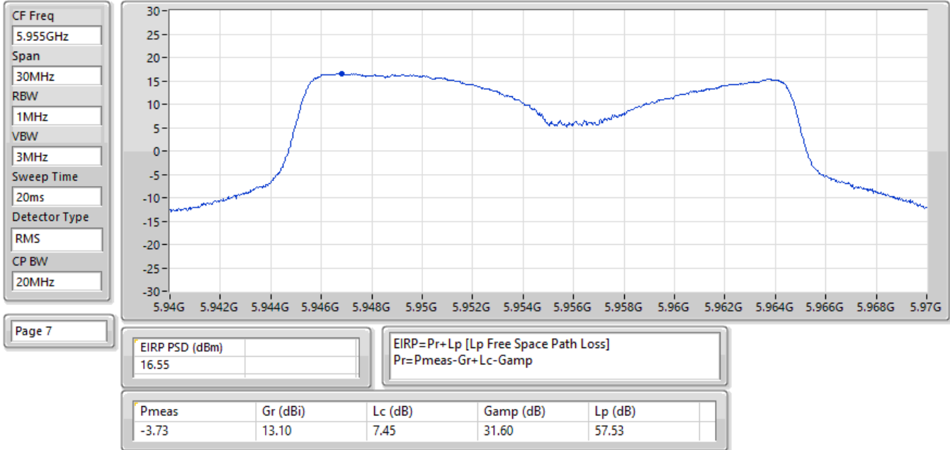
EIRP PSD;Band:6.2G;be20,BF;BWch:20MHz;Nss:1,(M0);Nant:2;Ch:5955MHz;TX
