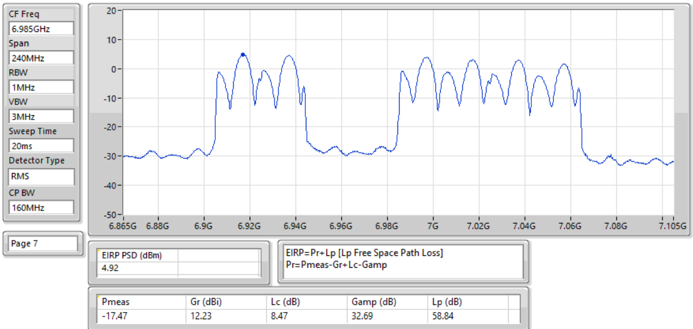
EIRP PSD;Band:7.0G;be160;BWch:160MHz;Nss:1,(M0),RU996+RU484 MRU 2;Nant:4;Ch:6985MHz;TX
