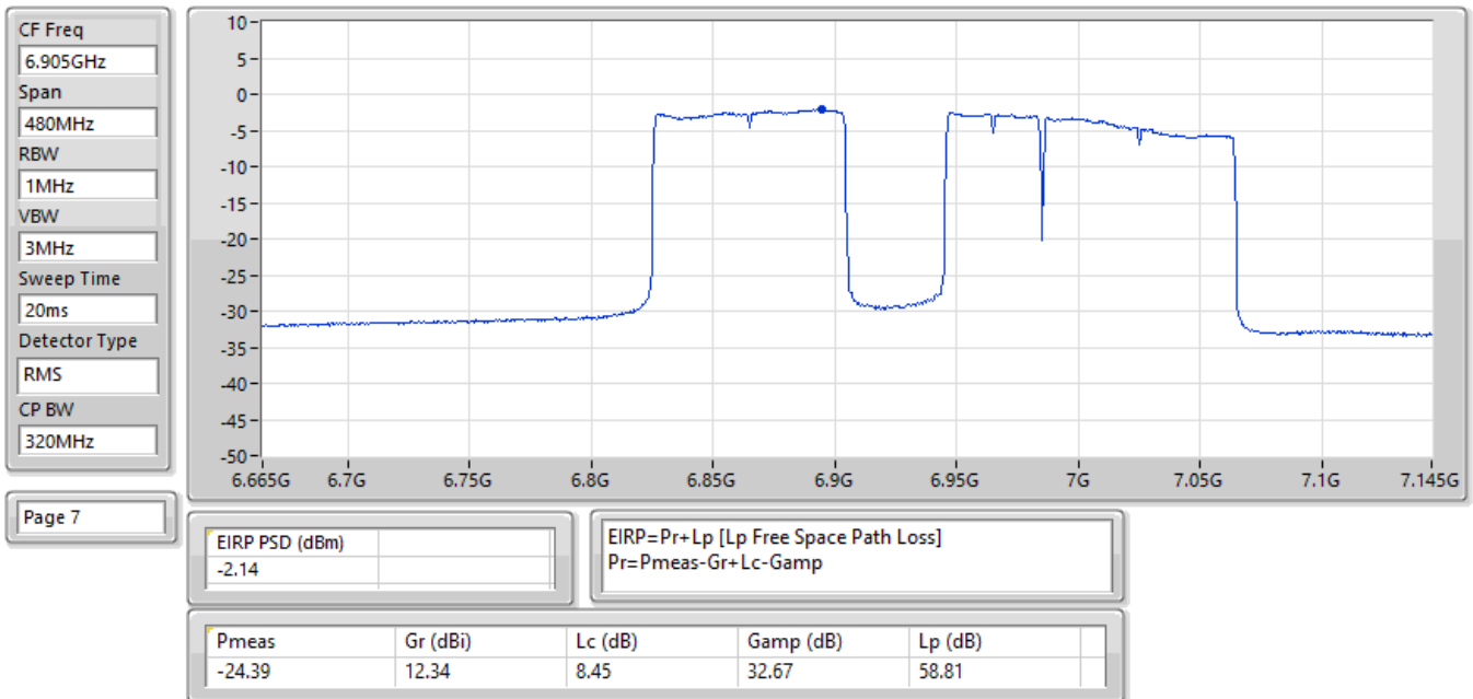
EIRP PSD;Band:6.7G;be320;BWch:320MHz;Nss:1,(M0),2xRU996+RU484 CP 9;Nant:1;Ch:6905MHz;TX
