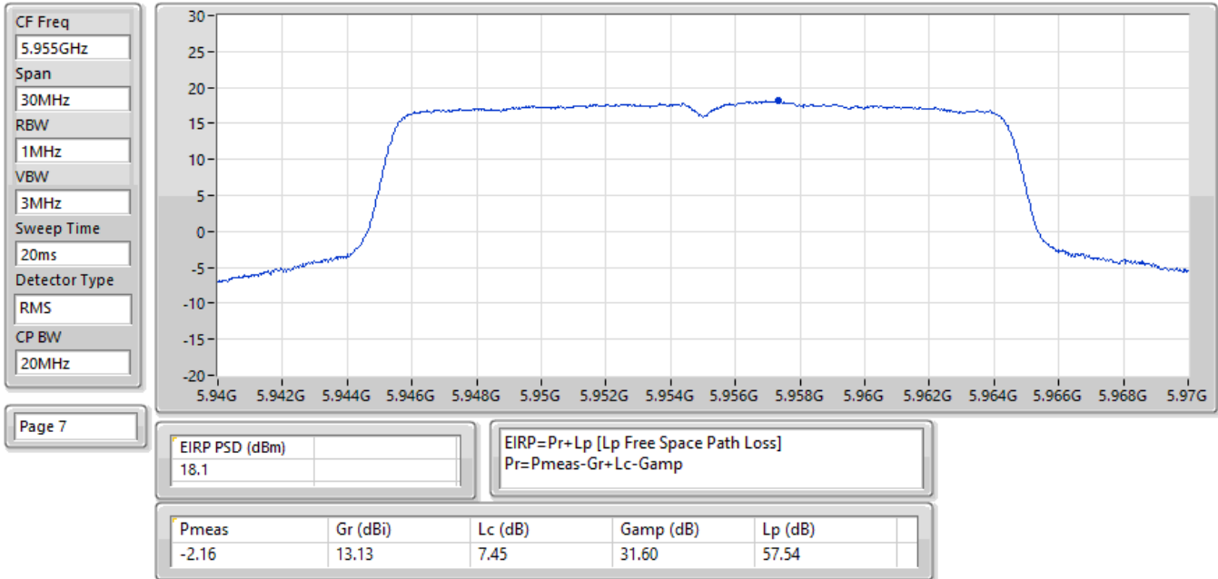
EIRP PSD;Band:6.2G;be20,BF;BWch:20MHz;Nss:1,(M0);Nant:4;Ch:5955MHz;TX
