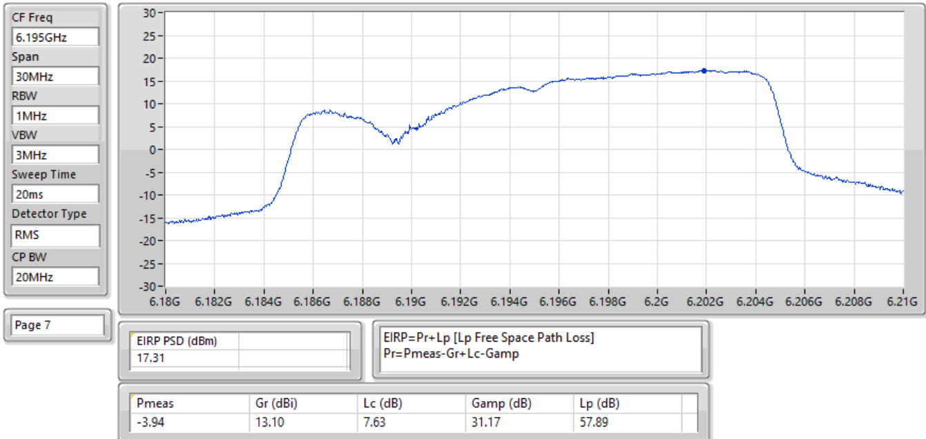
EIRP PSD;Band:6.2G;be20,BF;BWch:20MHz;Nss:1,(M0);Nant:2;Ch:6195MHz;TX
