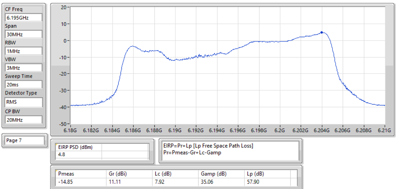
EIRP PSD;Band:6.2G;be20,BF;BWch:20MHz;Nss:1,(M0);Nant:2;Ch:6195MHz;TX
