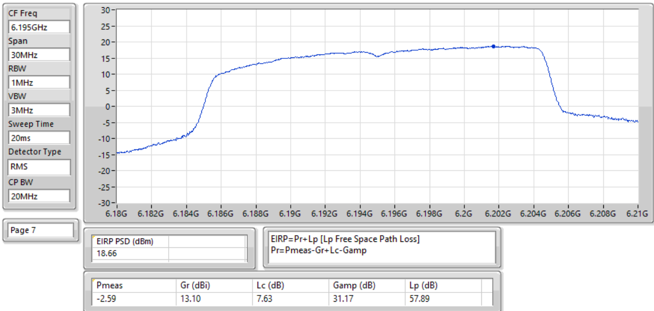
EIRP PSD;Band:6.2G;be20,BF;BWch:20MHz;Nss:1,(M0);Nant:4;Ch:6195MHz;TX
