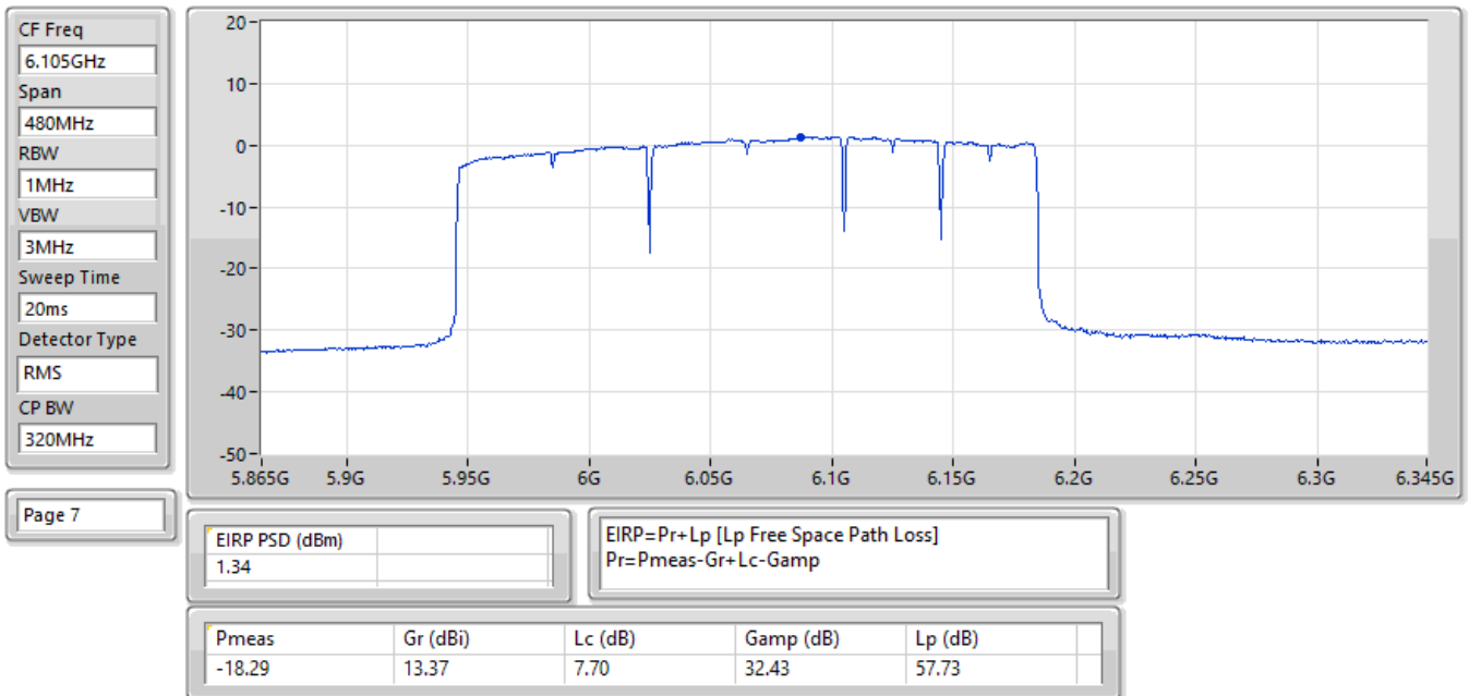
EIRP PSD;Band:6.2G;be320;BWch:320MHz;Nss:1,(M0),3xRU996 MRU 4;Nant:1;Ch:6105MHz;TX
