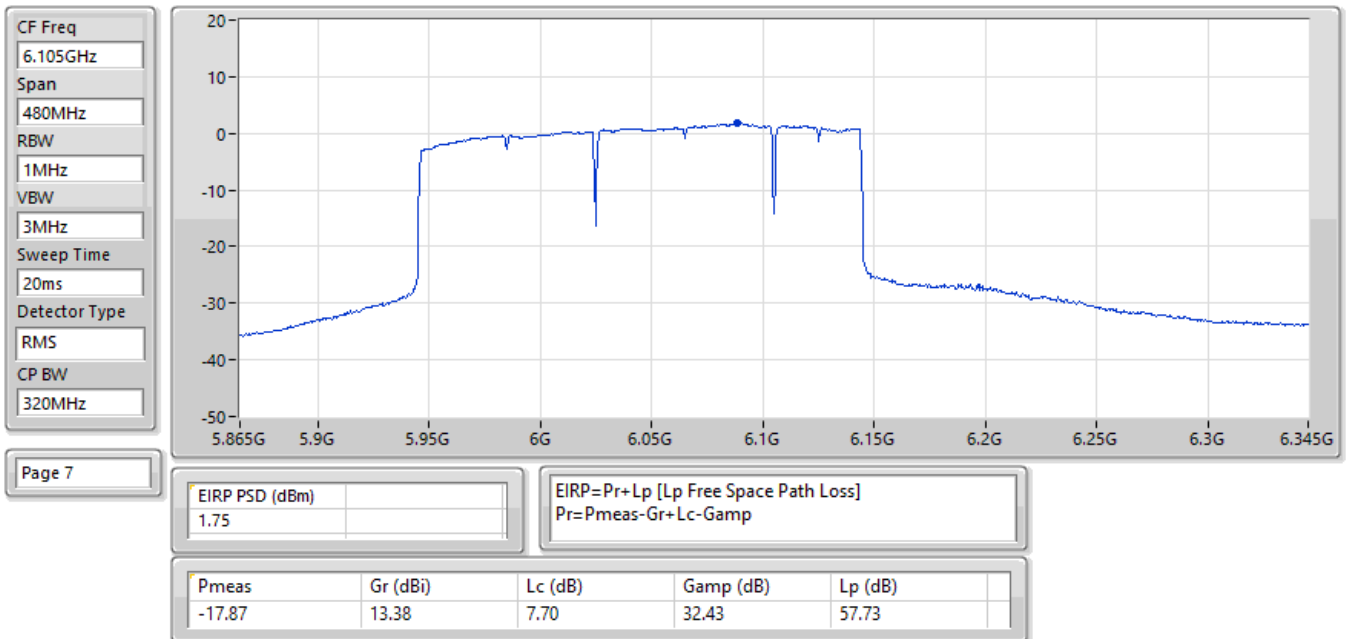
EIRP PSD;Band:6.2G;be320;BWch:320MHz;Nss:1,(M0),2xRU996+RU484 CP 6;Nant:1;Ch:6105MHz;TX
