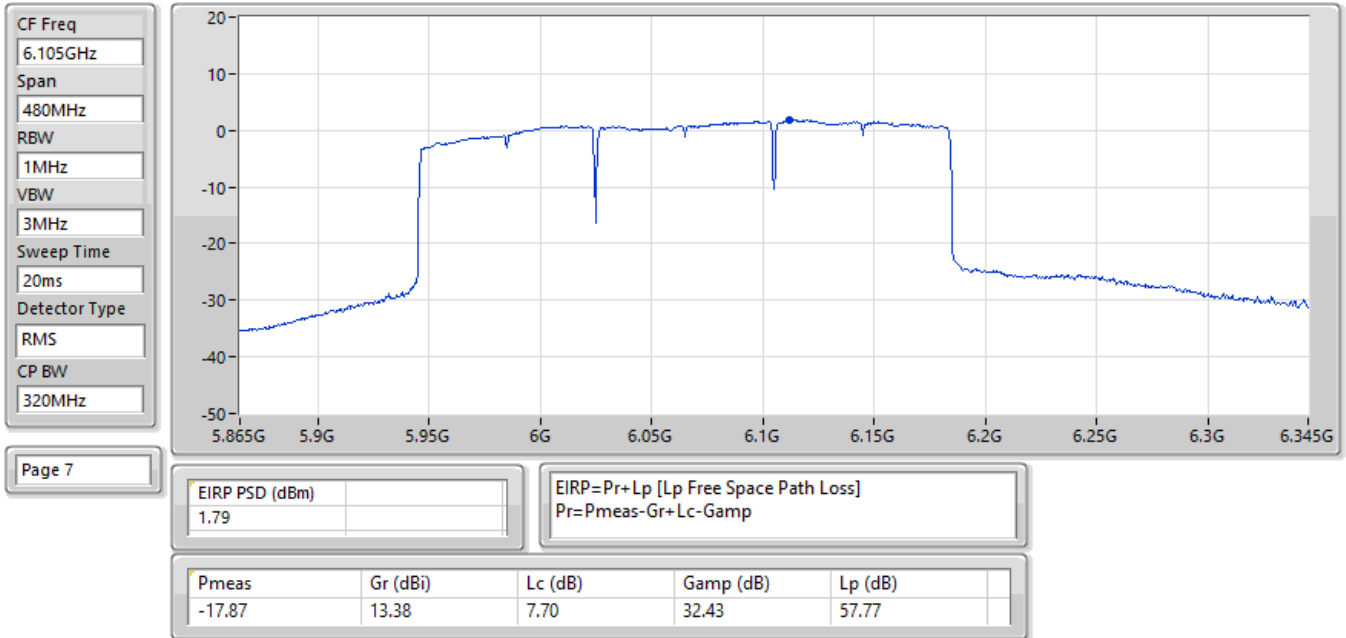
EIRP PSD;Band:6.2G;be320;BWch:320MHz;Nss:1,(M0),3xRU996 CP 4;Nant:1;Ch:6105MHz;TX
