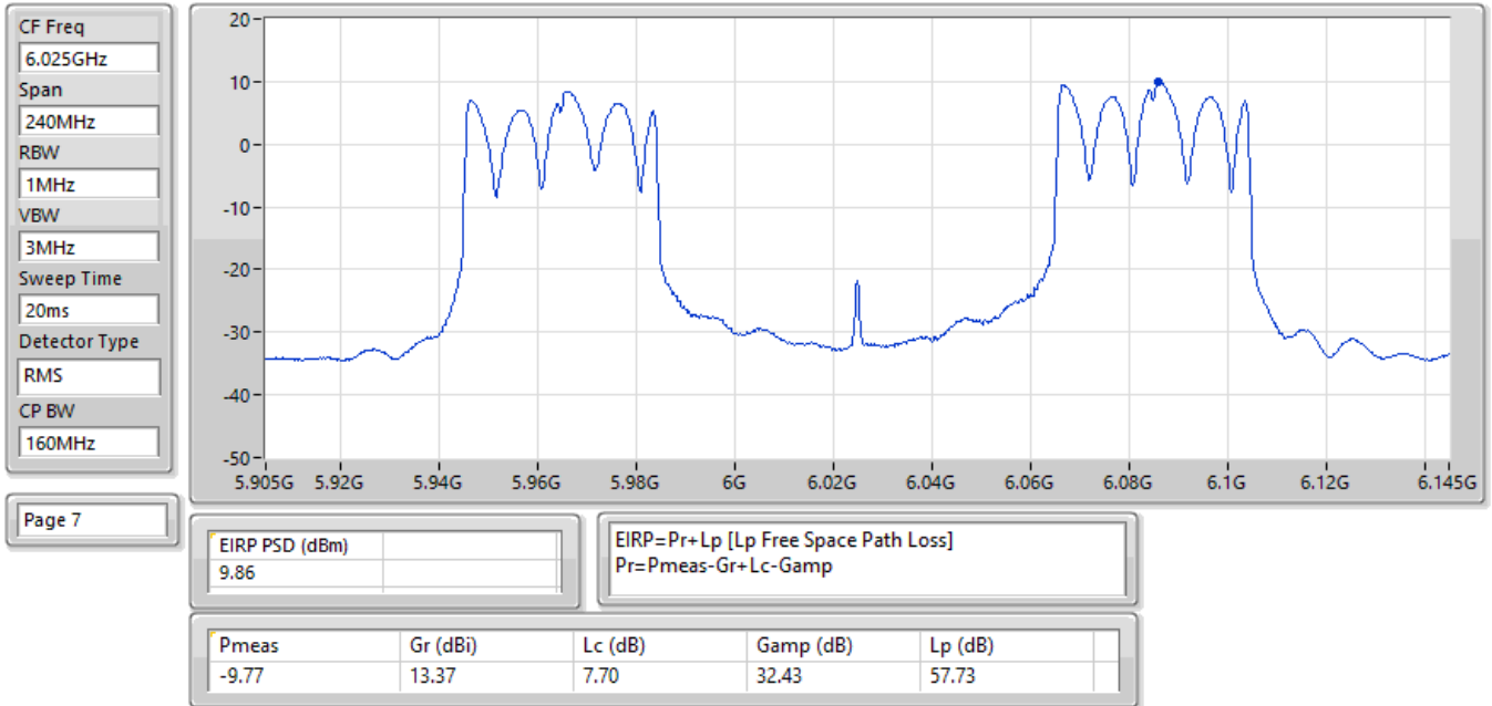
EIRP PSD;Band:6.2G;be160;BWch:160MHz;Nss:1,(M0),RU484+RU484 MRU 1;Nant:4;Ch:6025MHz;TX
