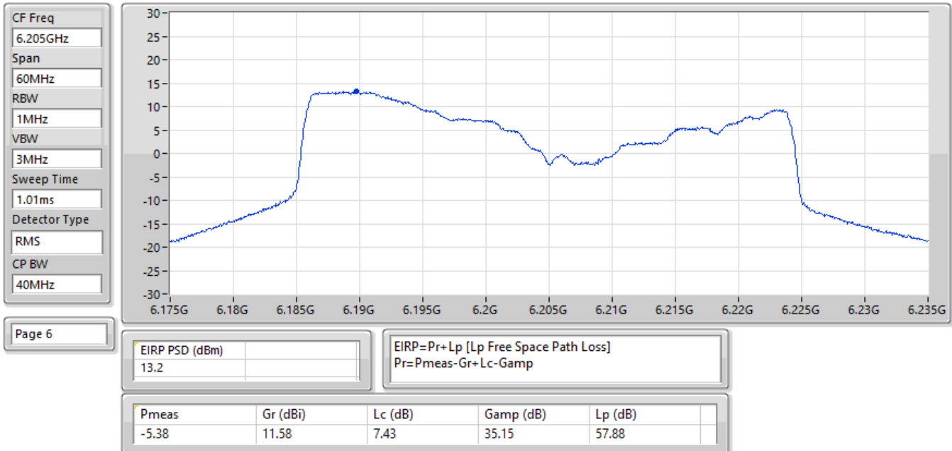
EIRP PSD;Band:6.2G;be40,BF;BWch:40MHz;Nss:1,(M0);Nant:2;Ch:6205MHz;TX
