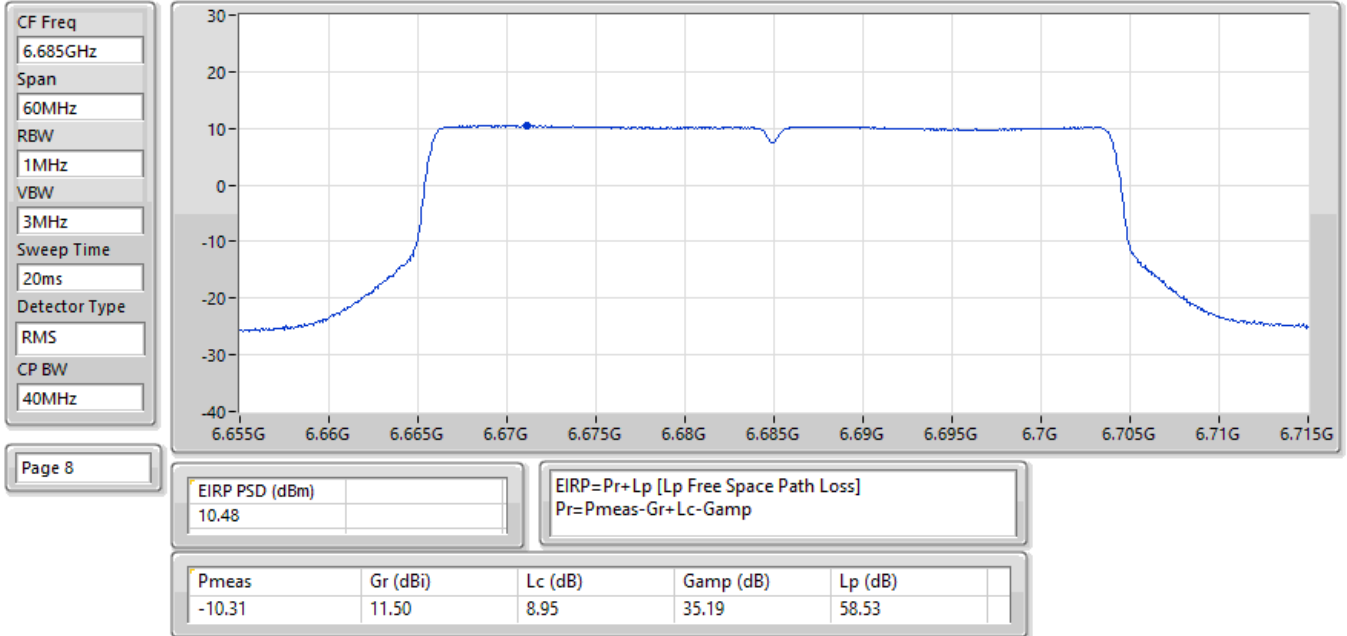
EIRP PSD;Band:6.7G;be40;BWch:40MHz;Nss:1,(M0);Nant:1(1);Ch:6685MHz;TX
