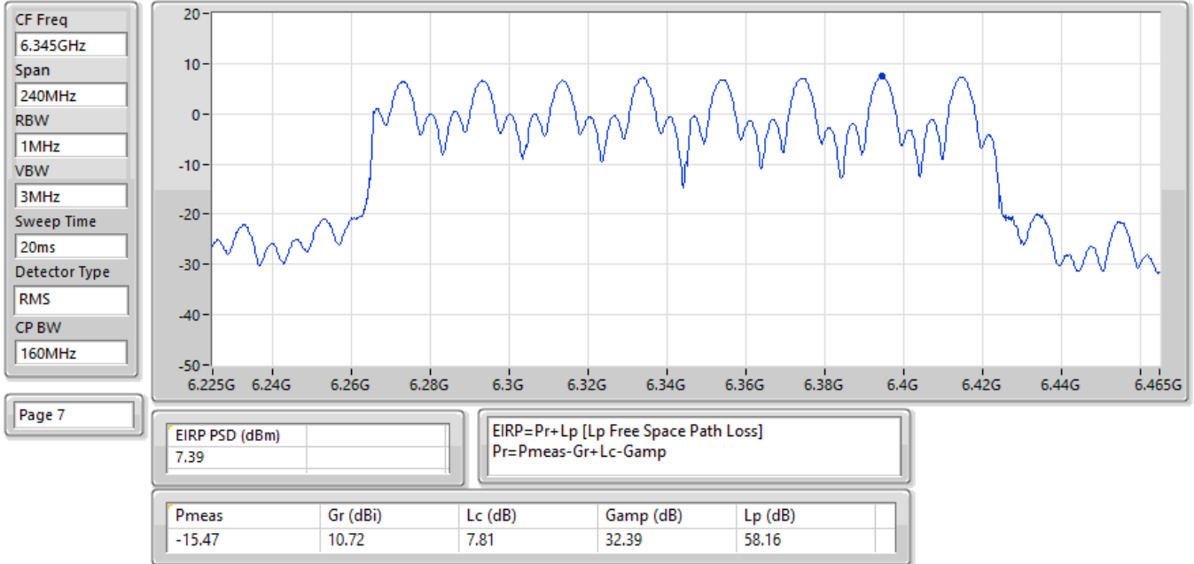
EIRP PSD;Band:6.2G;be160;BWch:160MHz;Nss:1,(M0);Nant:4;Ch:6345MHz;TX
