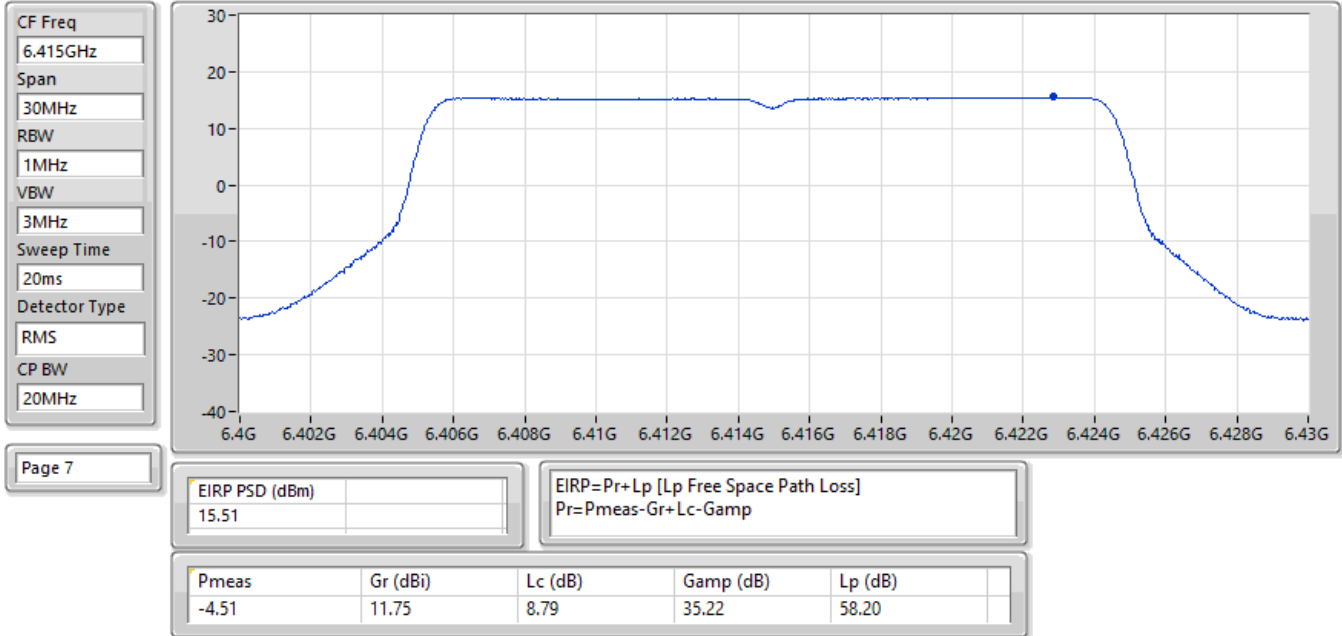
EIRP PSD;Band:6.2G;be20;BWch:20MHz;Nss:1,(M0);Nant:1(1);Ch:6415MHz;TX
