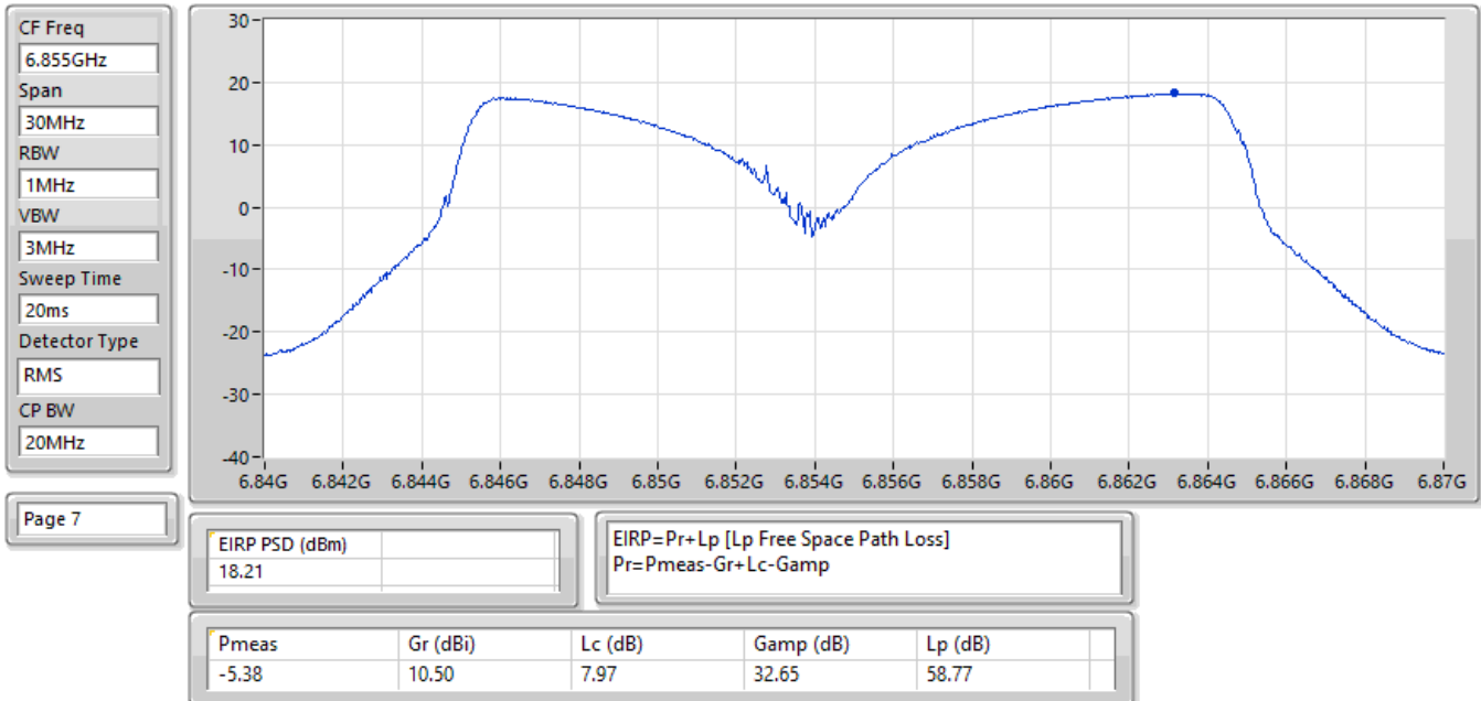
EIRP PSD;Band:6.7G;be20;BWch:20MHz;Nss:1,(M0);Nant:2(1,2);Ch:6855MHz;TX
