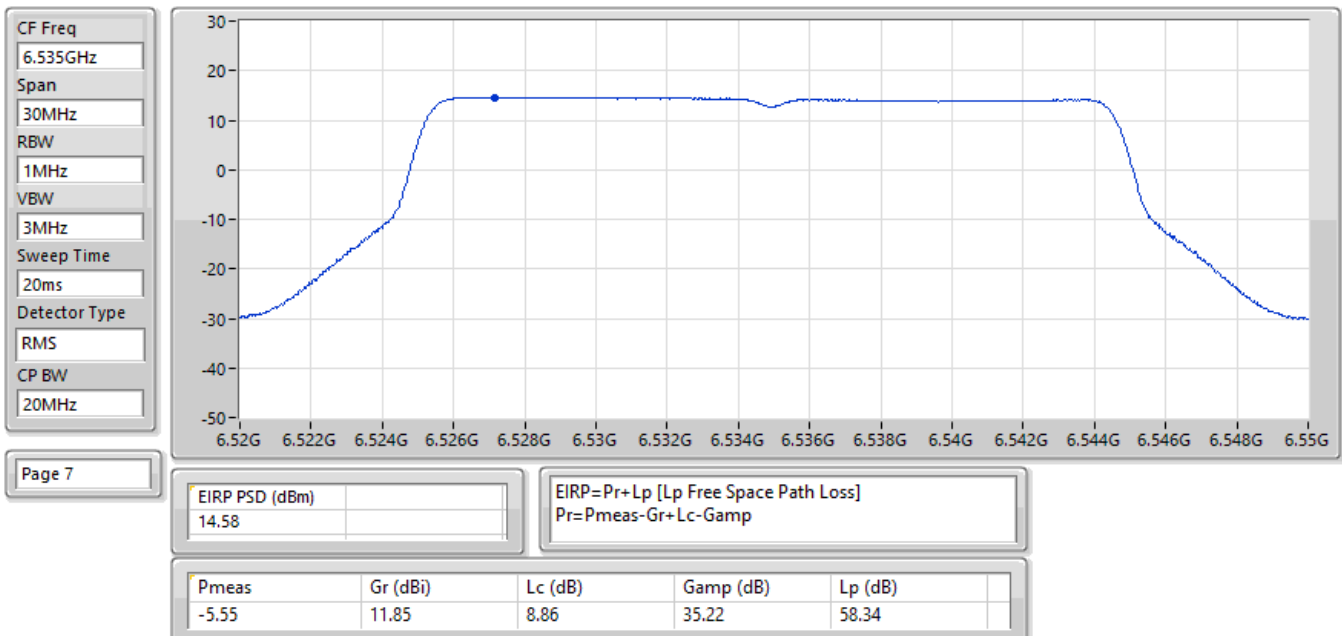
EIRP PSD;Band:6.7G;be20;BWch:20MHz;Nss:1,(M0);Nant:1(1);Ch:6535MHz;TX
