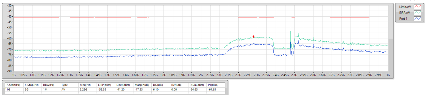
2.4-2.4835GHz_BT-LE(2Mbps)
