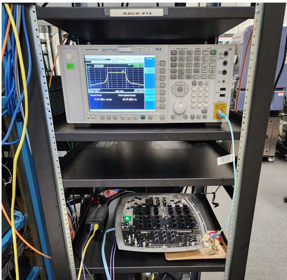
Title: AFC Setup - EUT
