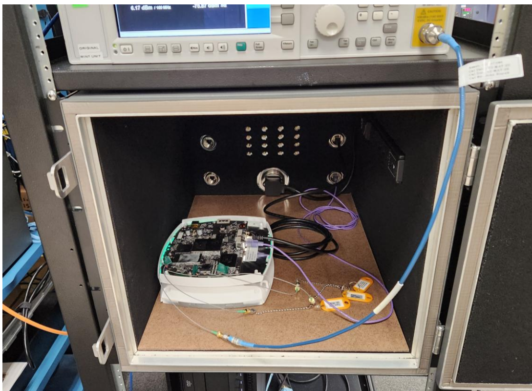
Title: AFC Setup - EUT
