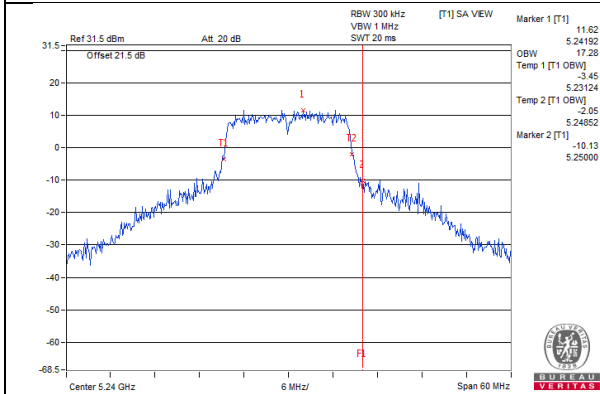
802.11a_Chain 2 / CH48
