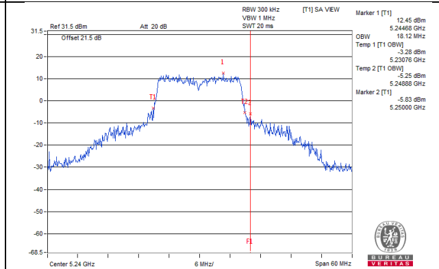
802.11a_Chain 3 / CH48
