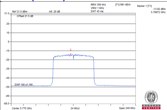
802.11ax (HE80+80) / Chain 3 : CH155
