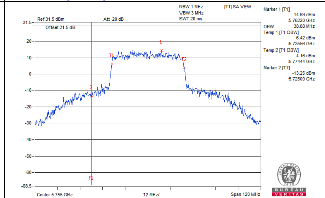
802.11ax (HE40)_Chain 3 / CH151
