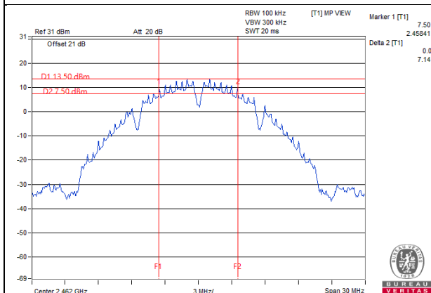
802.11ax (HE20) / Chain 2 : CH11
