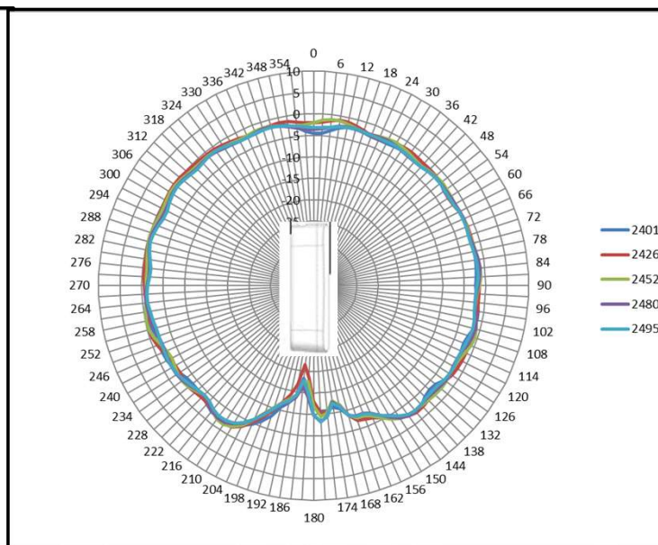
YZ-plane
