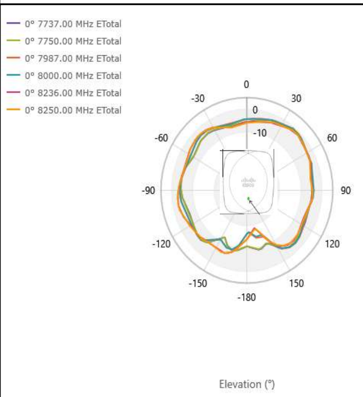
XZ-plane
