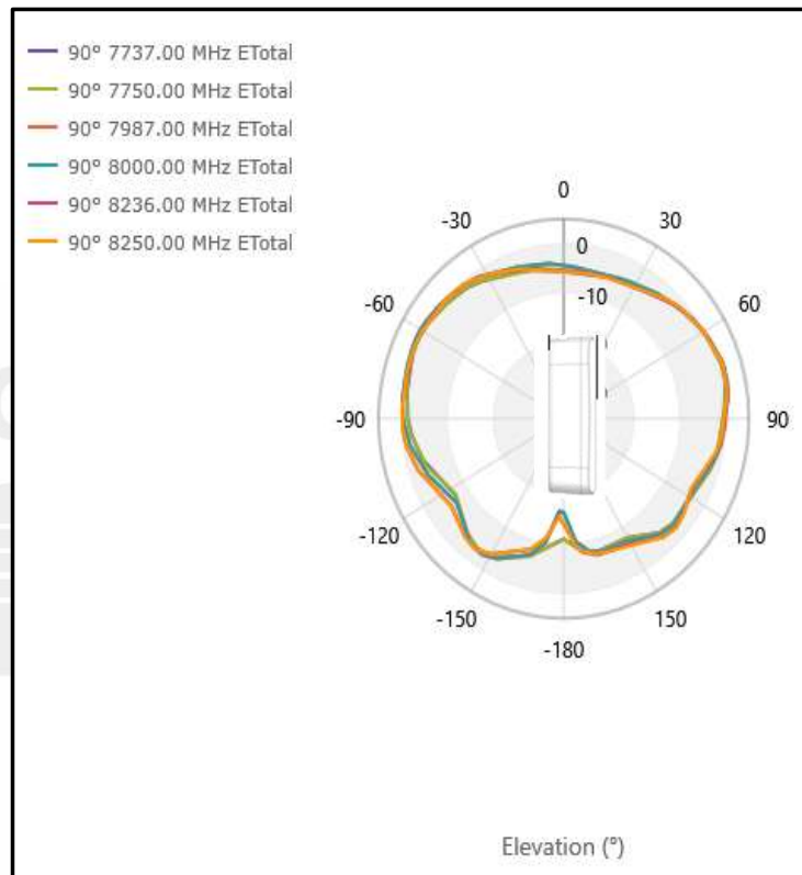
YZ-plane
