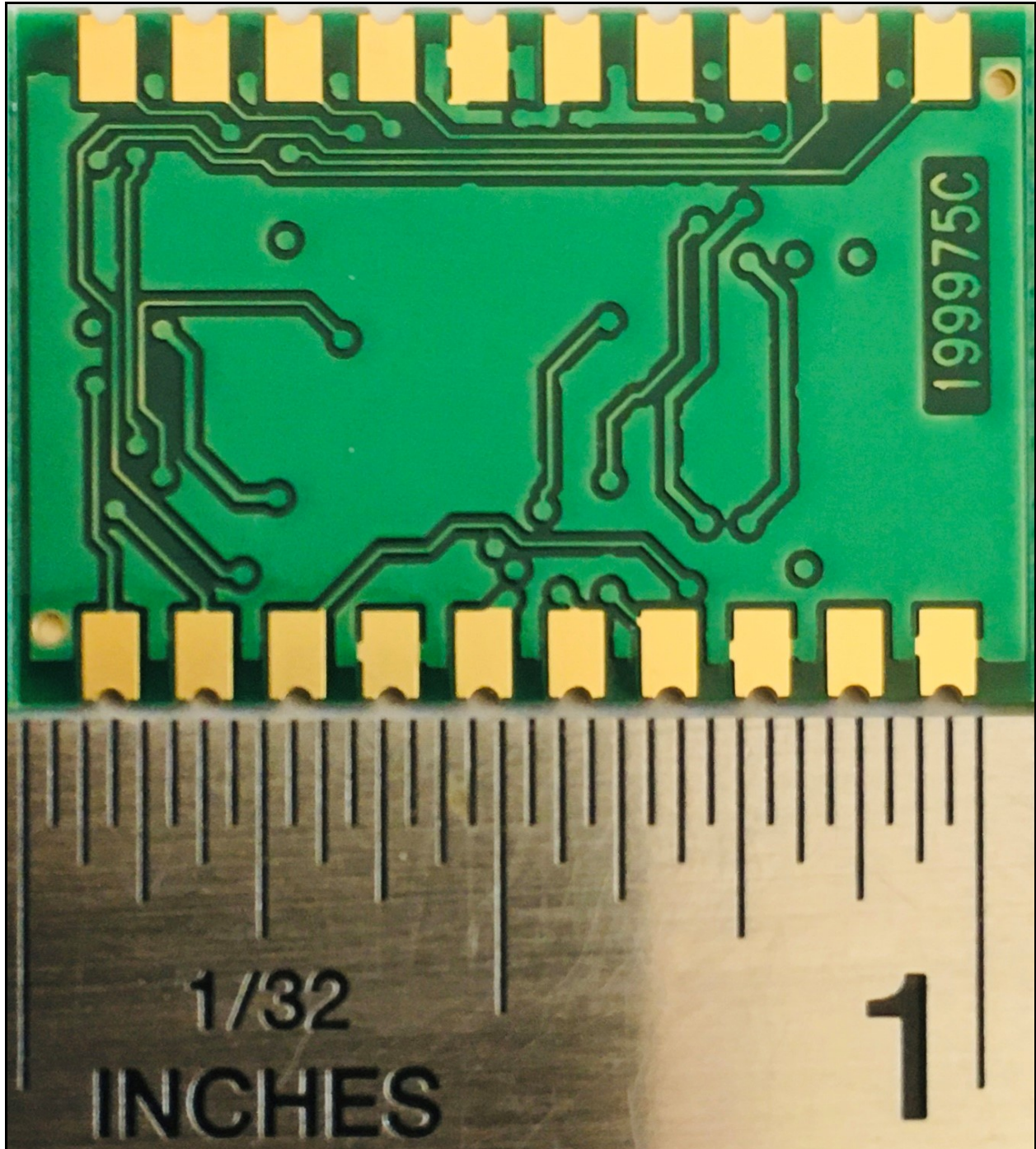
SX243 Module External Photos
